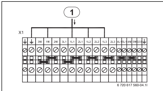
Bild 12 Standardausführung, STE 60-1 - 100-1 und STM 60-1 - 100-1
