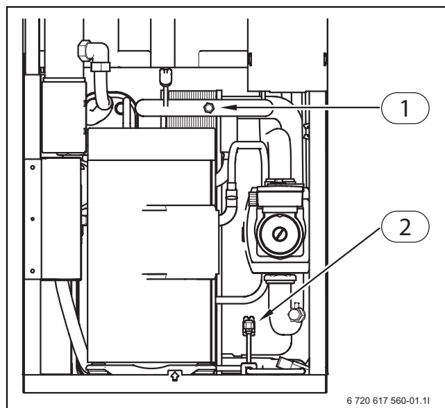
Bild 41 Lage der Schraderventile
