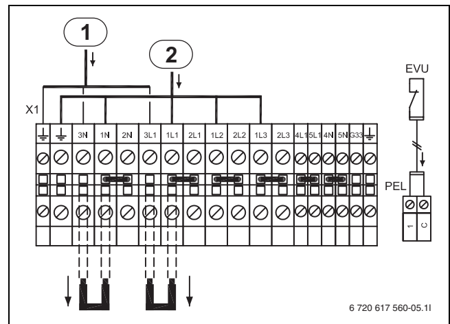
Bild 13 Alternative A, STE 60-1 - 100-1 und STM 60-1 - 100-1
