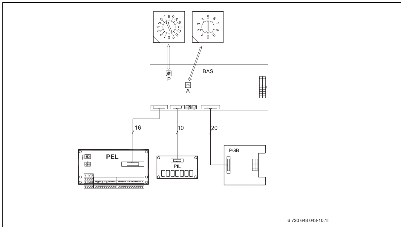
Bild 9 Leiterplattenverbindungen
