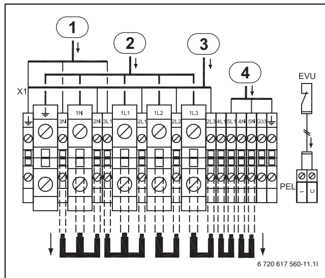
Bild 19 Alternative C, STE 130-1 - 170-1
