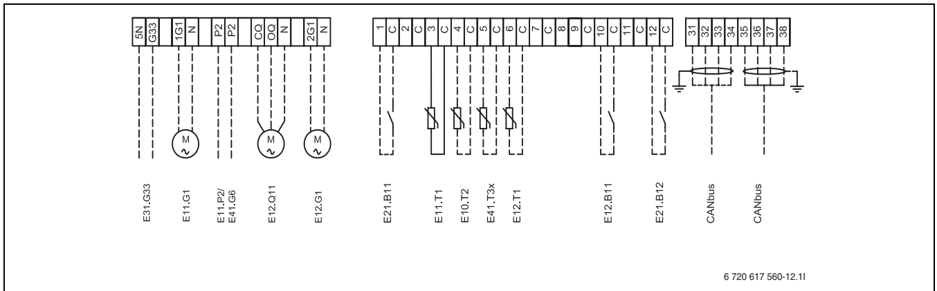
Bild 20 Externe Anschlüsse
