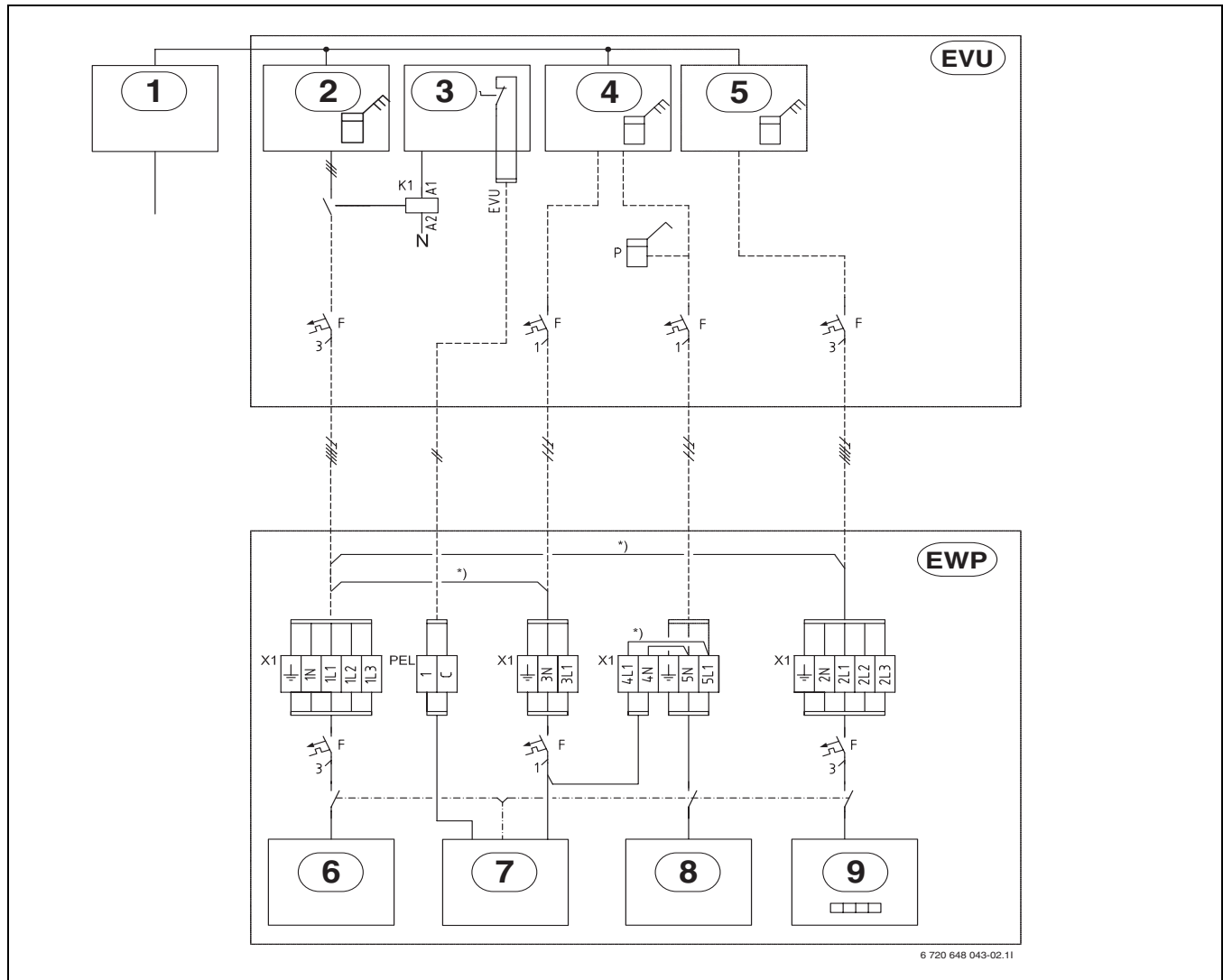
Bild 6 Anschlussübersicht Elektroschaltschrank - Wärmepumpe
