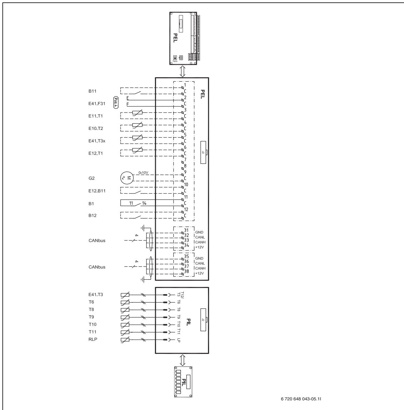
Bild 23 Kompletter Anschlussschaltplan (Niederspannung)
