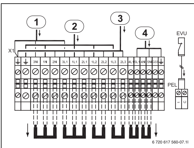
Bild 15 Alternative C, STE 60-1 - 100-1 und STM 60-1 - 100-1
