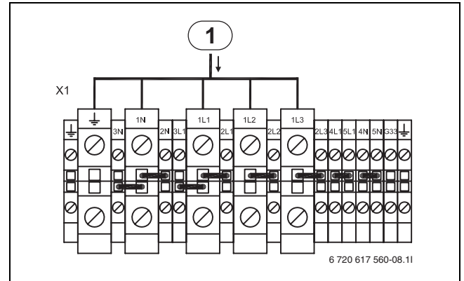
Bild 16 Standardausführung, STE 130-1 - 170-1
