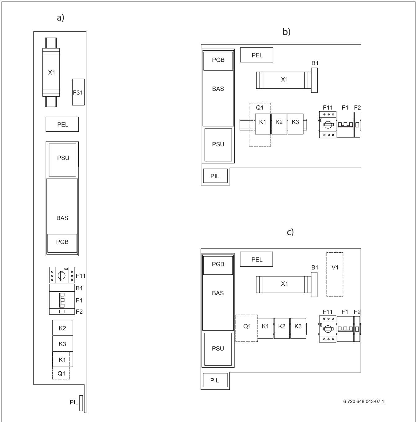
Bild 7 Übersicht Leiterplatte
