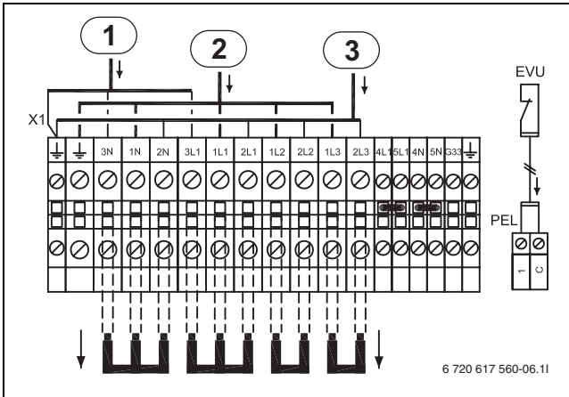
Bild 14 Alternative B, STE 60-1 - 100-1 und STM 60-1 - 100-1
