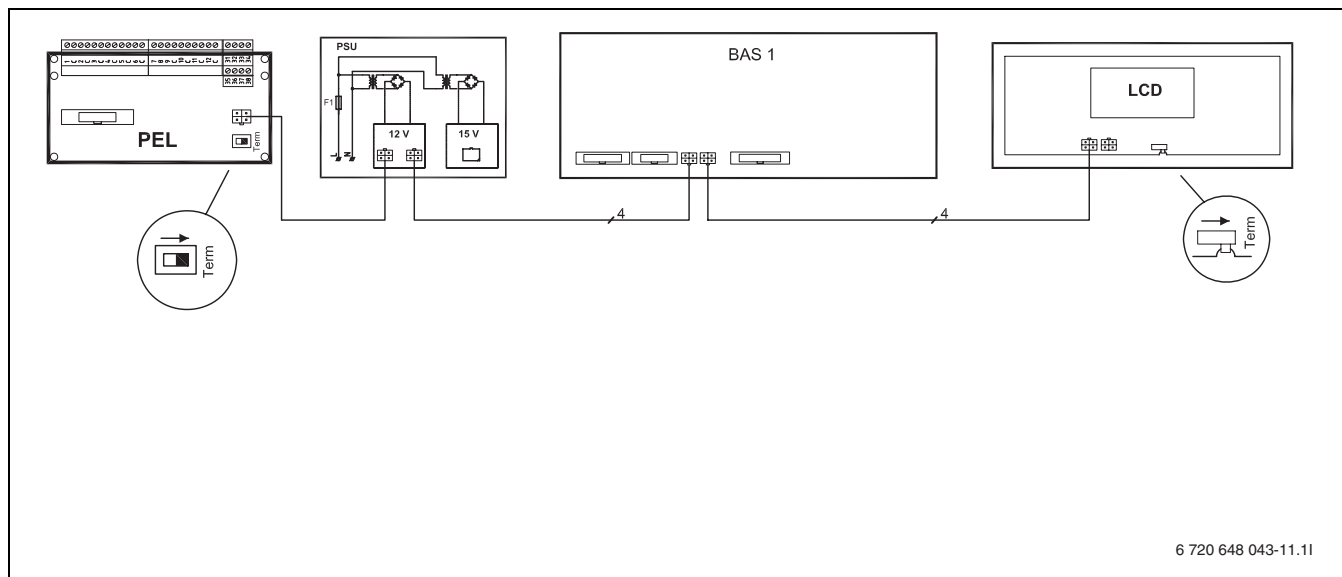
Bild 8 CAN-BUS-Übersicht
