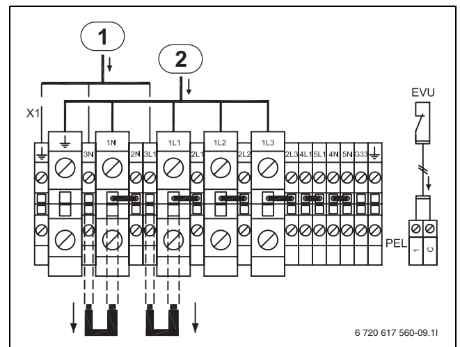
Bild 17 Alternative A, STE 130-1 - 170-1
