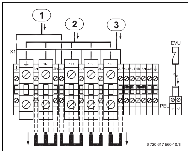
Bild 18 Alternative B, STE 130-1 - 170-1
