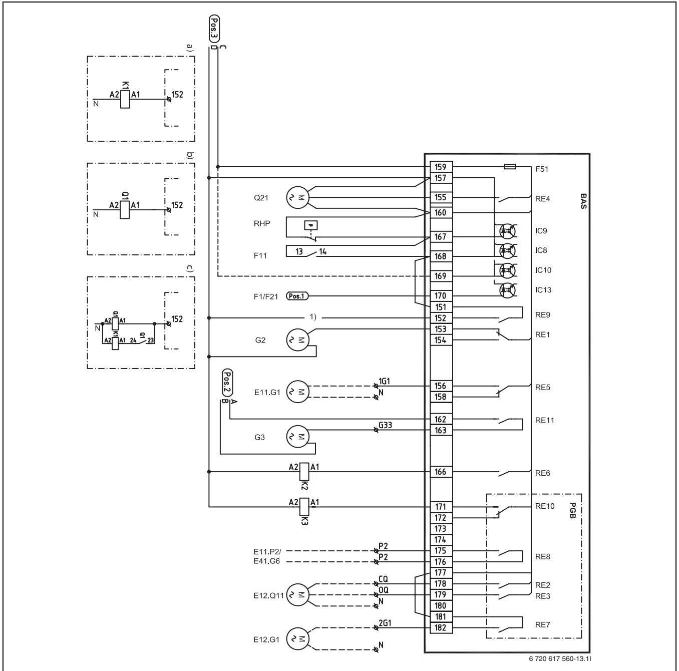
Bild 22 Kompletter Anschlusschaltplan (230 V)
