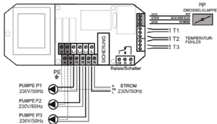
Abb. 3_Elektroinstallationschema
