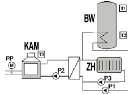
Abb.1c: Betriebsschema der Steuerung in Verbindung mit Wärmeaustauscher für die ZH Schaltung und BW Schaltung.
