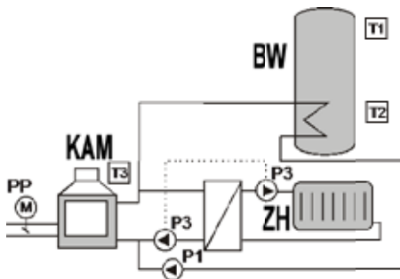
Abb.1b: Betriebsschema der Steuerung in Verbindung mit Wärmeaustauscher für die ZH Schaltung (Die Pumpe des Wärmeaustauschers und der ZH wird an den Ausgang P3 angeschlossen.)
