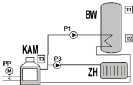
Abb.1a: Grundbetriebsschema der Steuerung
