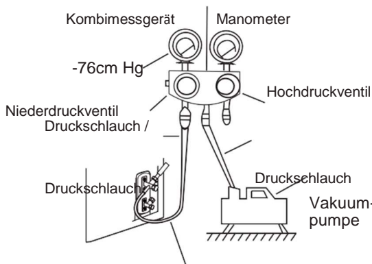
Niederdruckventil
