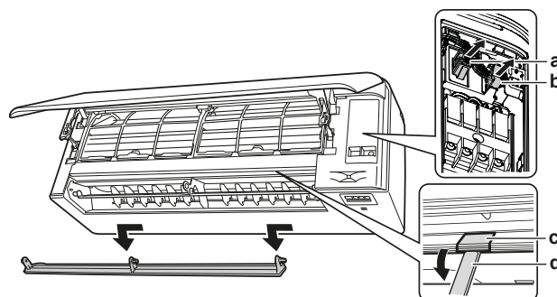
a Konnektor b Drahtklammer c Schraubenabdeckung d Langer flacher, in ein Tuch gewickelter Gegenstand
