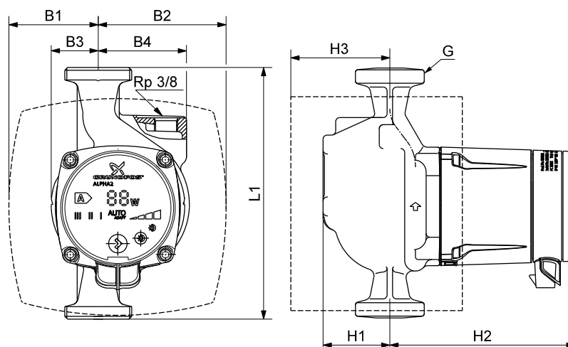
Abb. 16 Maßskizzen, ALPHA2 25-40 A, 25-60 A
