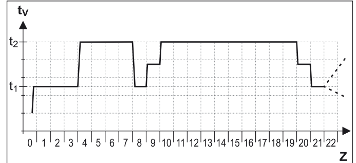
Bild 3-19 Zeitlicher Ablauf des Estrichprogramms beim kombinierten Funktions- und Belegreifheizen (Legende siehe Bild 3-18)
