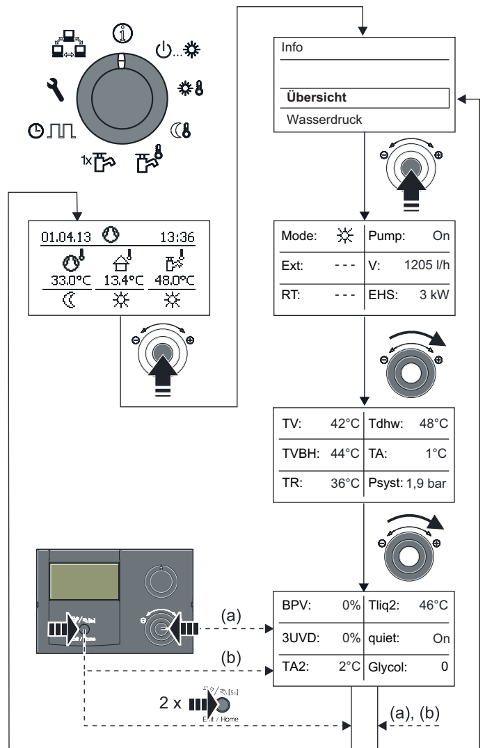
Bild 3-5 Betriebsdatenübersicht anzeigen
