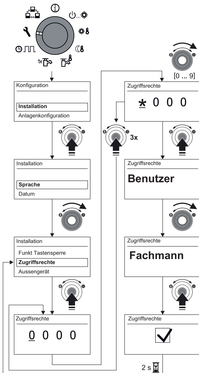
Bild 3-13 Zugangscode eingeben
