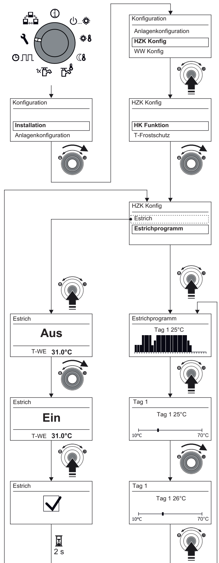
Bild 3-20 Estrichprogramm einstellen
