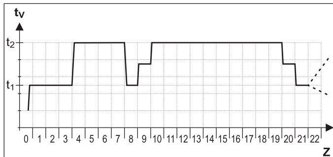
Bild 3-20 Zeitlicher Ablauf des Estrichprogramms beim kombinierten Funktions- und Belegreifheizen (Legende siehe Bild 3-19)
