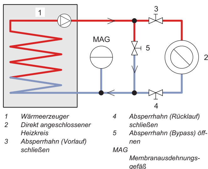
Bild 3-14 Hydraulikschaltung für STB Test bei Heizkreisinstallation mit Wärmebeständigkeit unter 105 °C
