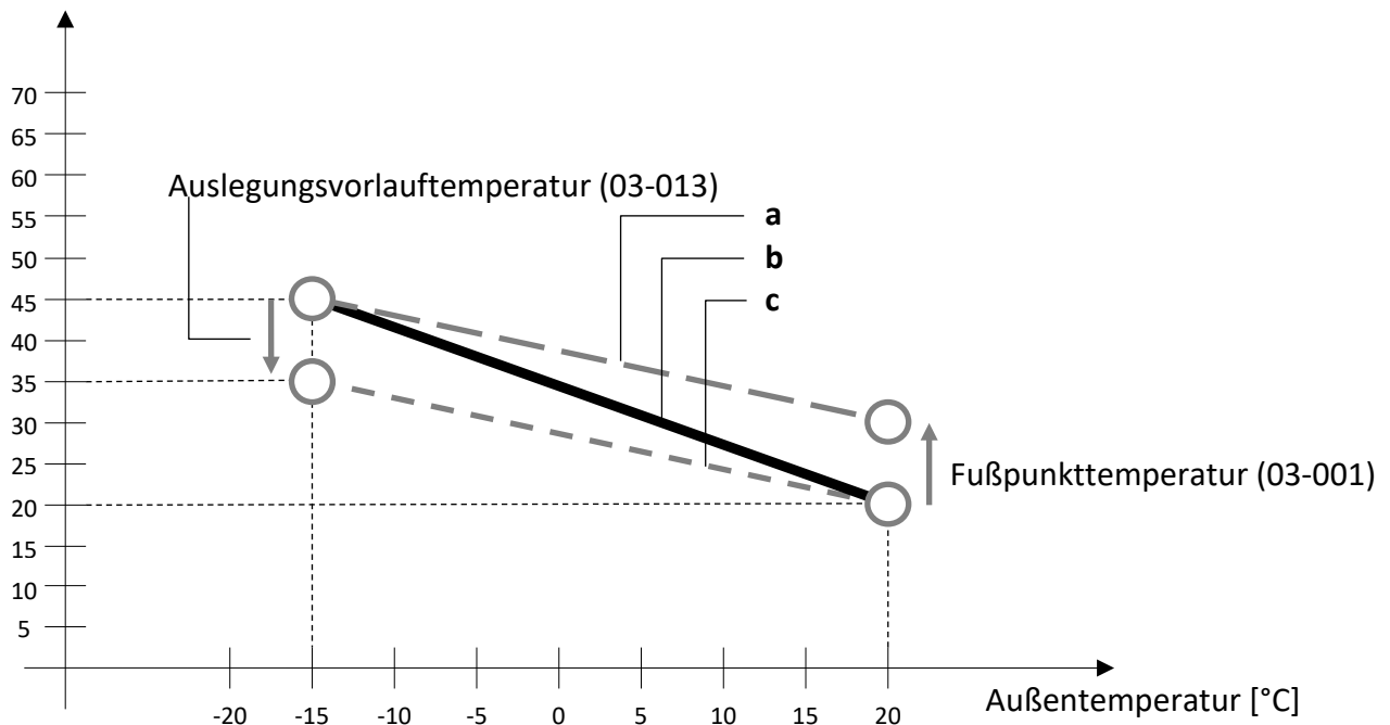
Abbildung 9: Heizkurve Korrektur
