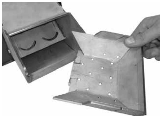
Herausnehmbare Verbrennungskammer mit den Öffnungen für die Luftzufuhr – muss regelmäßig gereinigt werden
