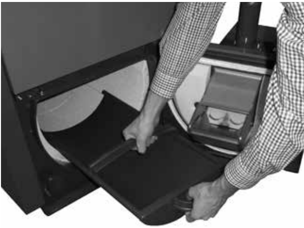
Verbrennungsraum des Kessels mit beispielhafter Entleerung mit dem Aschekasten
