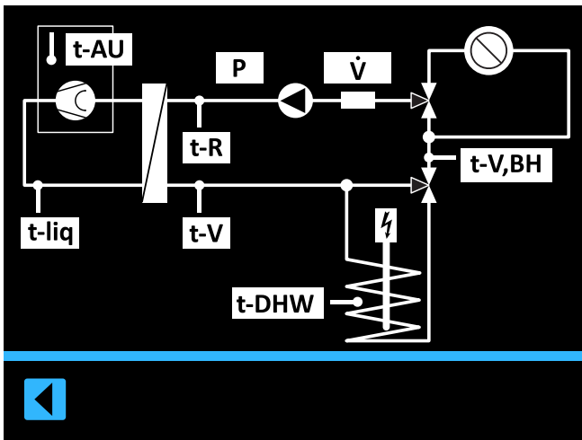
Bild 4-7 Hydraulikschaftbild - Erste Seite
