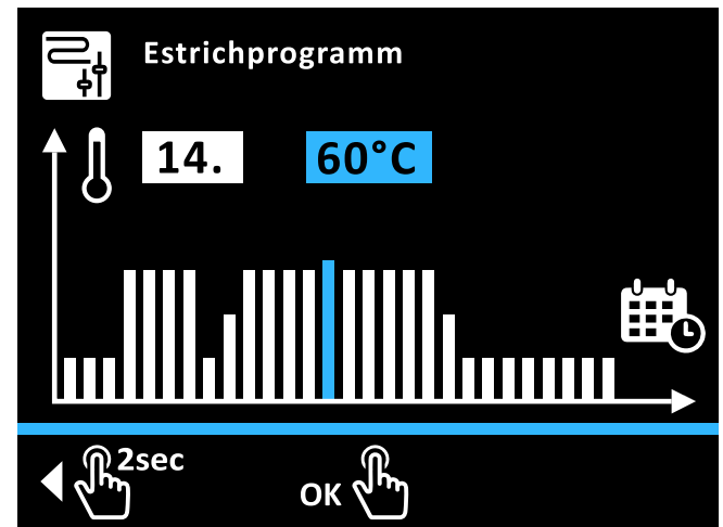
Bild 4-4 Estrichprogramm ändern
