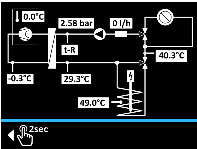
Bild 4-8 Hydraulikschaftbild - Zweite Seite
