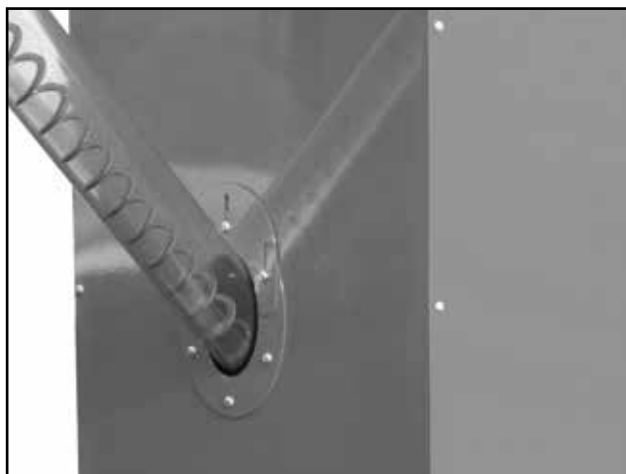
Aufgestellter Pelletsförderer. Die ovalförmige Reduktion dient zur Verkleinerung der Öffnungen bei den Förderanlagen Typ DAxxxx. Das Hufeisen dichtet die Öffnung bei verschiedenem Gefälle des Förderer ab.
