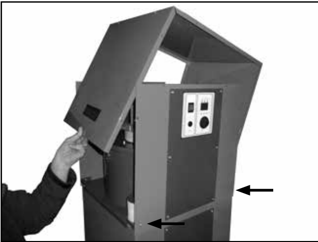
Bei der Kontrolle des Motors oder des Abscheidebehälters kann das mittlere Gehäuse entfernt werden
