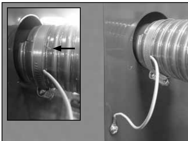
Empfohlene Erdung beider Schläuche als Schutz gegen elektrostatische Aufladung. Abisolierter Schlauchseil mit dem Erdungsleiter und Klemmband.
