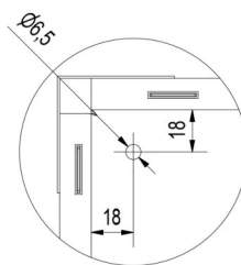
Otwór montażowy mierzony od krawędzi komory spalania
