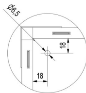
Otwór montażowy mierzony od krawędzi komory spalania
