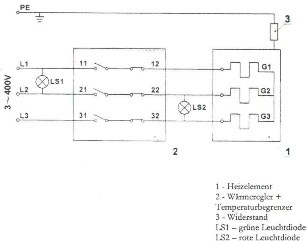
Abb. 2 Das elektrische Schema
