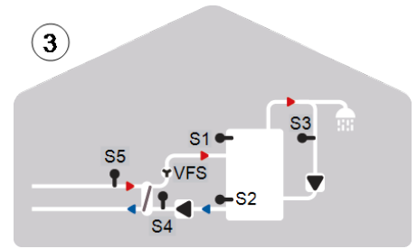
Speicherladung mit VFS und Zirkulation
