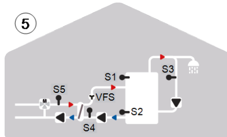
Speicherladung mit VFS, Primärpumpe, Primärmischer und Zirkulation
