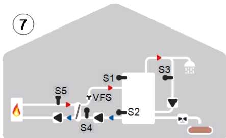
Speicherladung mit VFS, Primärpumpe, AL Aufheizung, Zirkulation und Spülung
