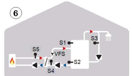
Speicherladung mit VFS, Primärpumpe, AL Aufheizung und Zirkulation
