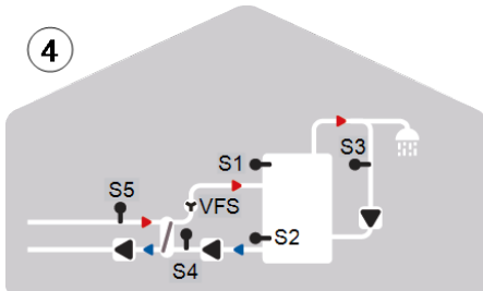
Speicherladung mit VFS, Primärpumpe und Zirkulation
