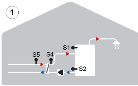
Speicherladung ohne VFS
