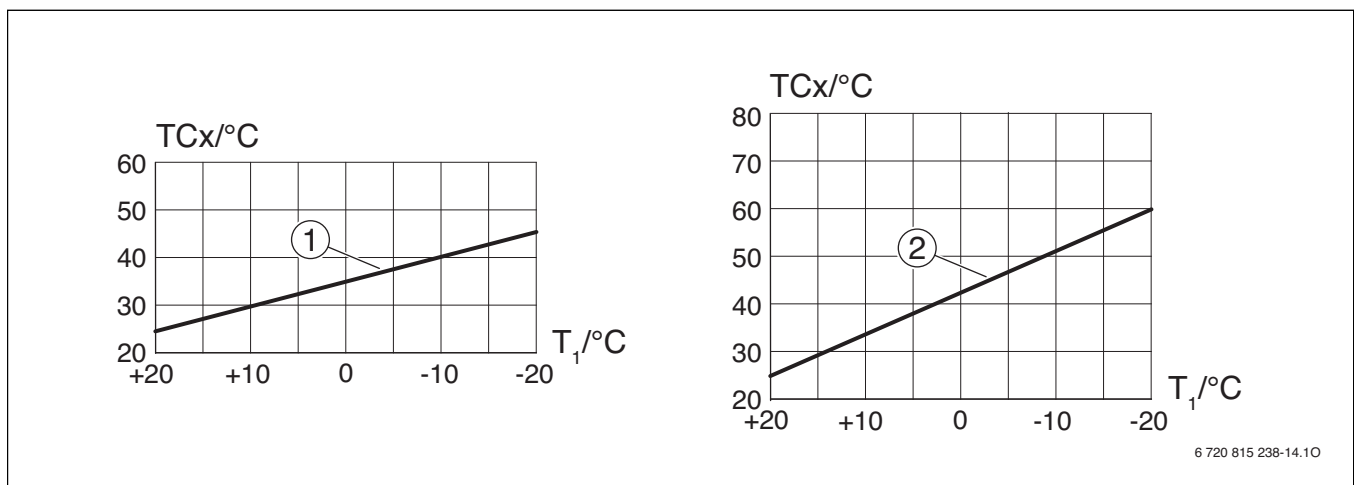
Bild 10 Instellungen der einfachen Heizkurven
