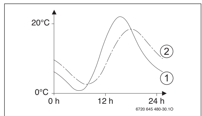
Bild 7 Beispiel für die gedämpfte Außentemperatur
