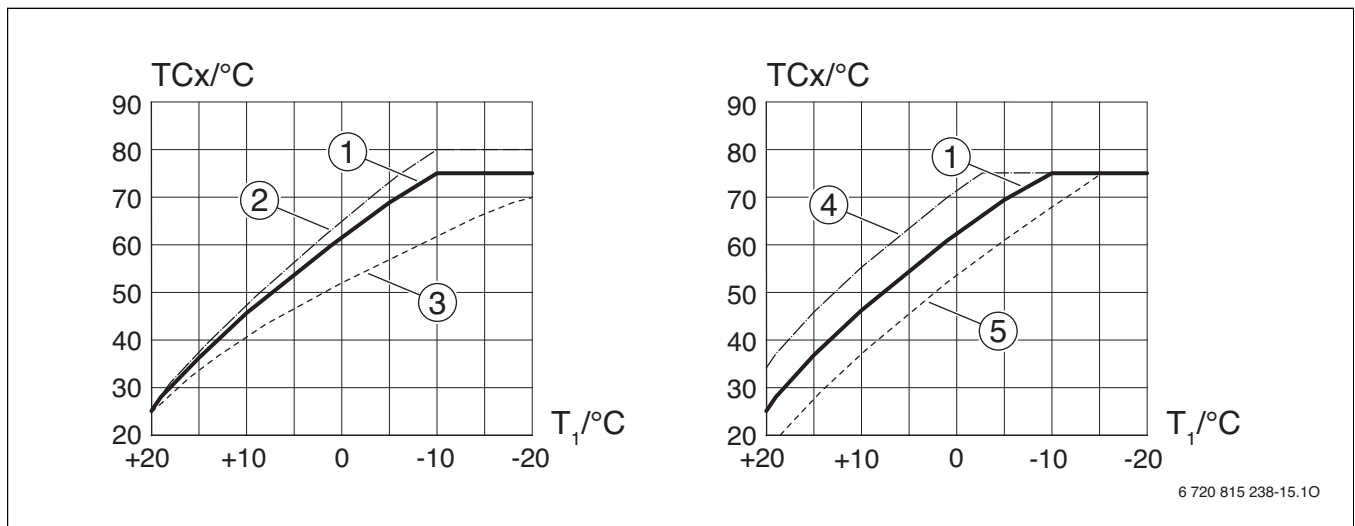
Bild 9 Einstellung der Heizkurve für Heizkörper / Konvektoren Links: Steigung über Auslegungstemperatur T AL und minimale Außentemperatur T 1,min Rechts: Parallelverschiebung über Raumtemperatur-Offset oder über gewünschte Raumtemperatur
