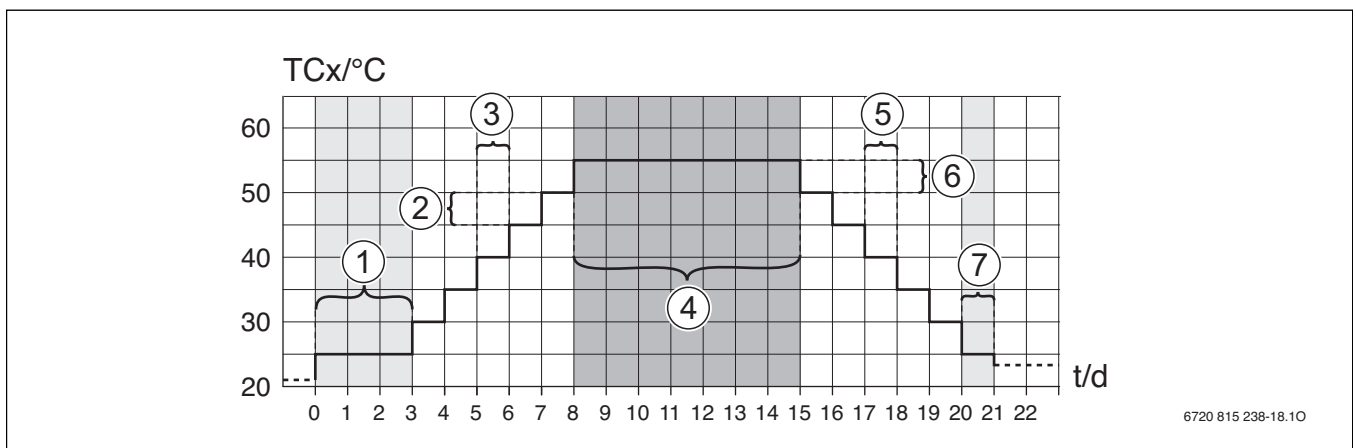
Bild 13 Ablauf der Estrichrocknung mit Grundeinstellungen
