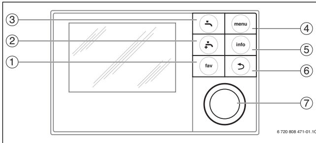
Bild 1 Bedienelemente
