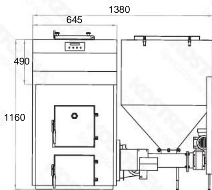
Frontansicht
