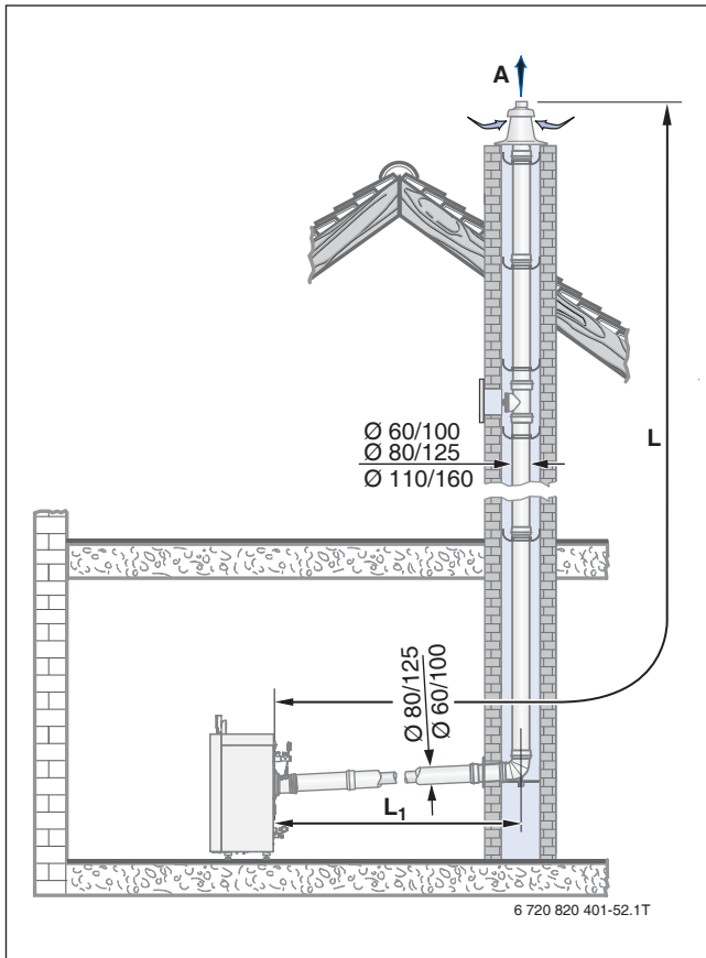
Bild 115 Montagevarianten mit dem Bausatz DO-S
