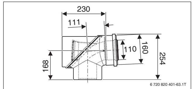
Bild 149 Konzentrisches T-Stück mit Prüföffnung Ø 110/160 (Maße in mm)
