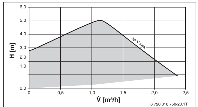
Bild 74 Restförderhöhe HSM25 V3: \Delta p -V
