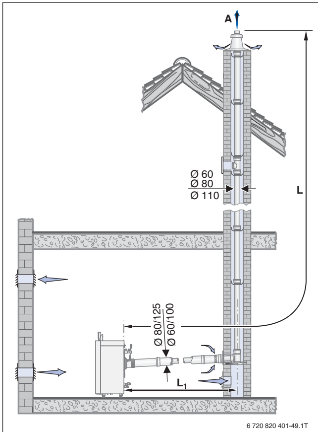
Bild 112 Montagevariante mit dem Bausatz GA-X + GA-K
