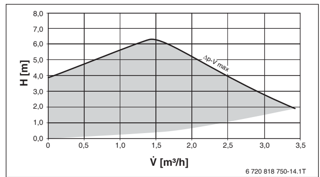
Bild 68 Restförderhöhe HS32 V3: \Delta p -V
