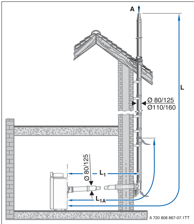
Bild 127 Montagevarianten mit dem Bausatz GAF-K
