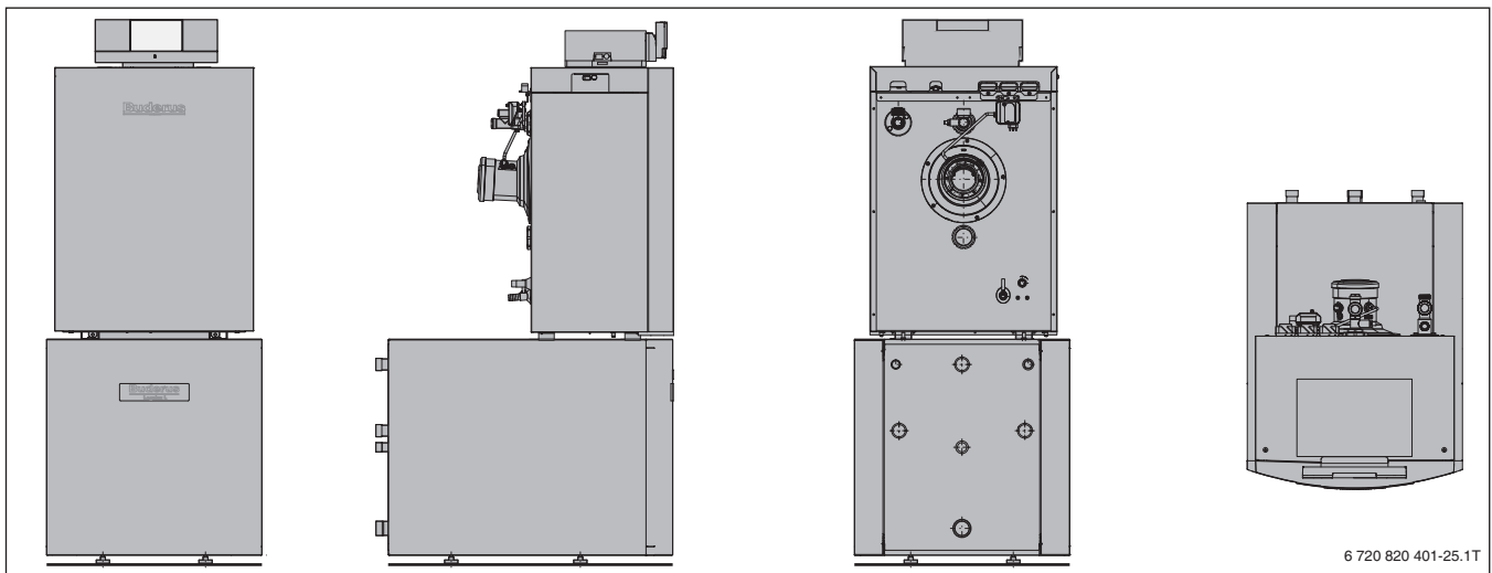
Bild 55 Logano plus GB212 mit Warmwasserspeicher Logalux L/2R
