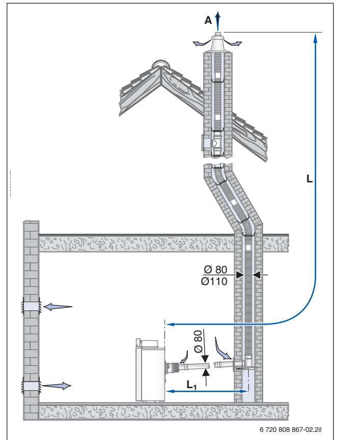
Bild 121 Montagevariante mit dem Bausatz GA + ÜB-flex
