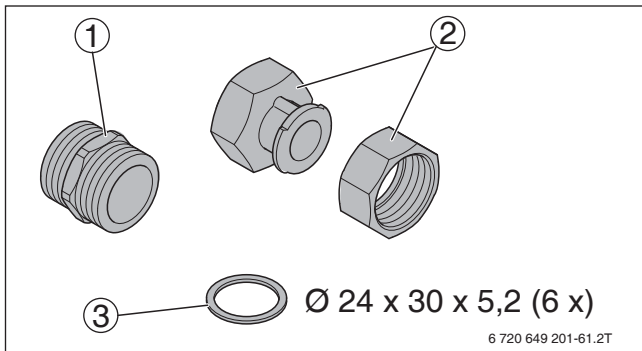
Bild 84 Anschluss-Set Wärmemengenzähler
