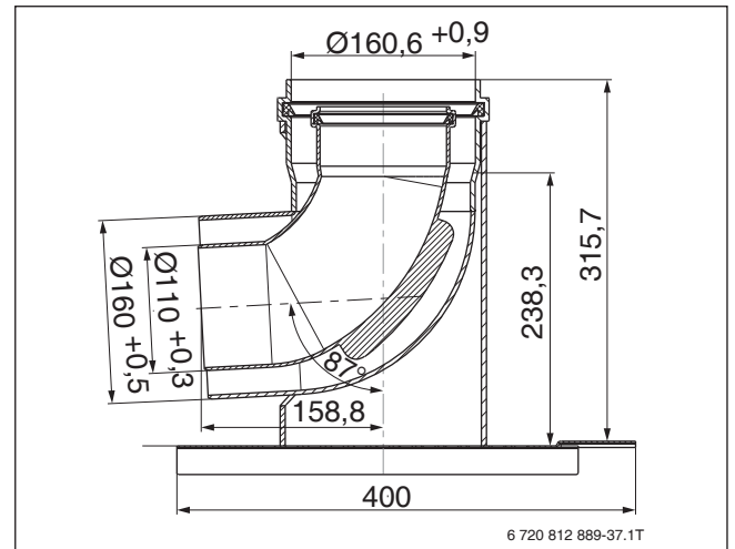
Bild 178 Stützbogen für DO-S in DN 110/160
