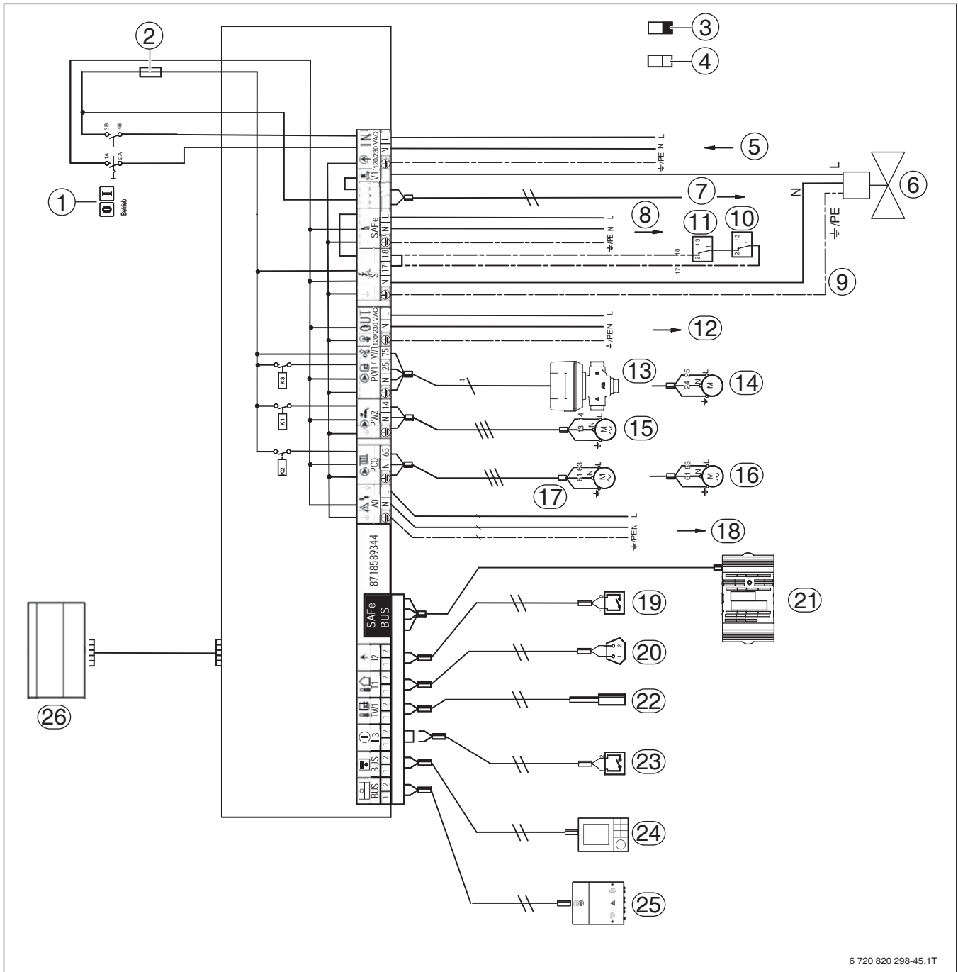
Bild 39 Schaltplan Mastercontroller Logamatic IMC110/MC110
