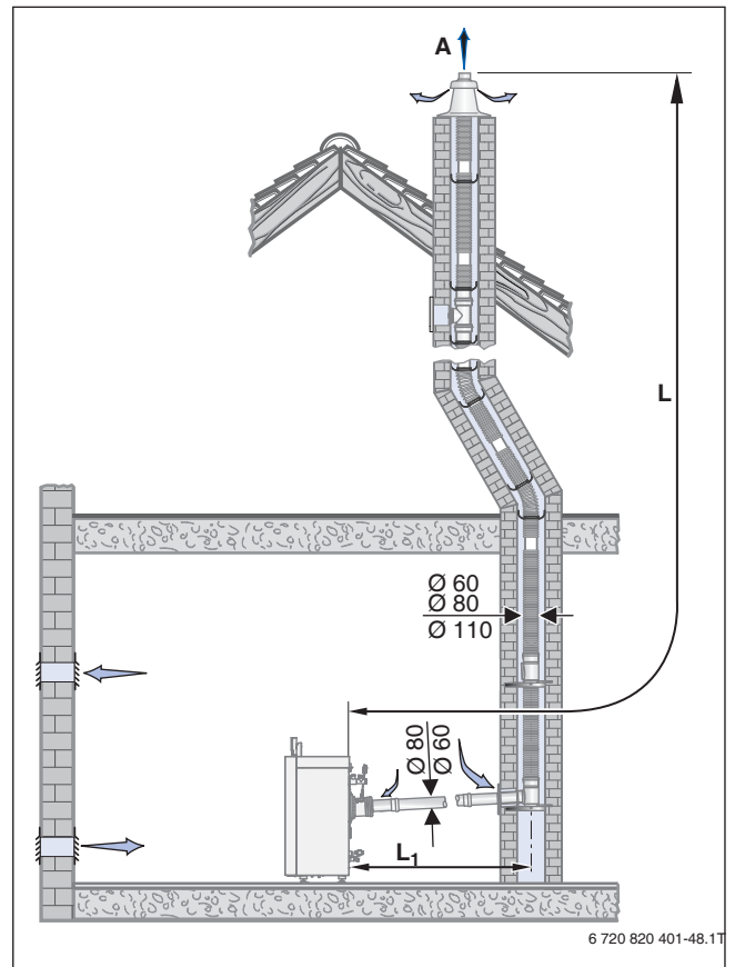
Bild 111 Montagevariante mit dem Bausatz GA + ÜB-Flex
