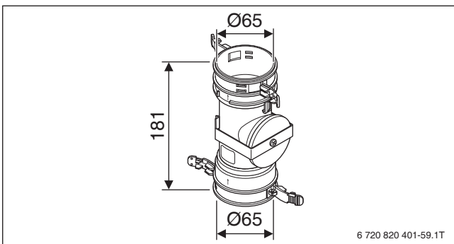
Bild 137 Verbindungsstück Flex mit Prüföffnung Ø 60 mm (Maße in mm)
