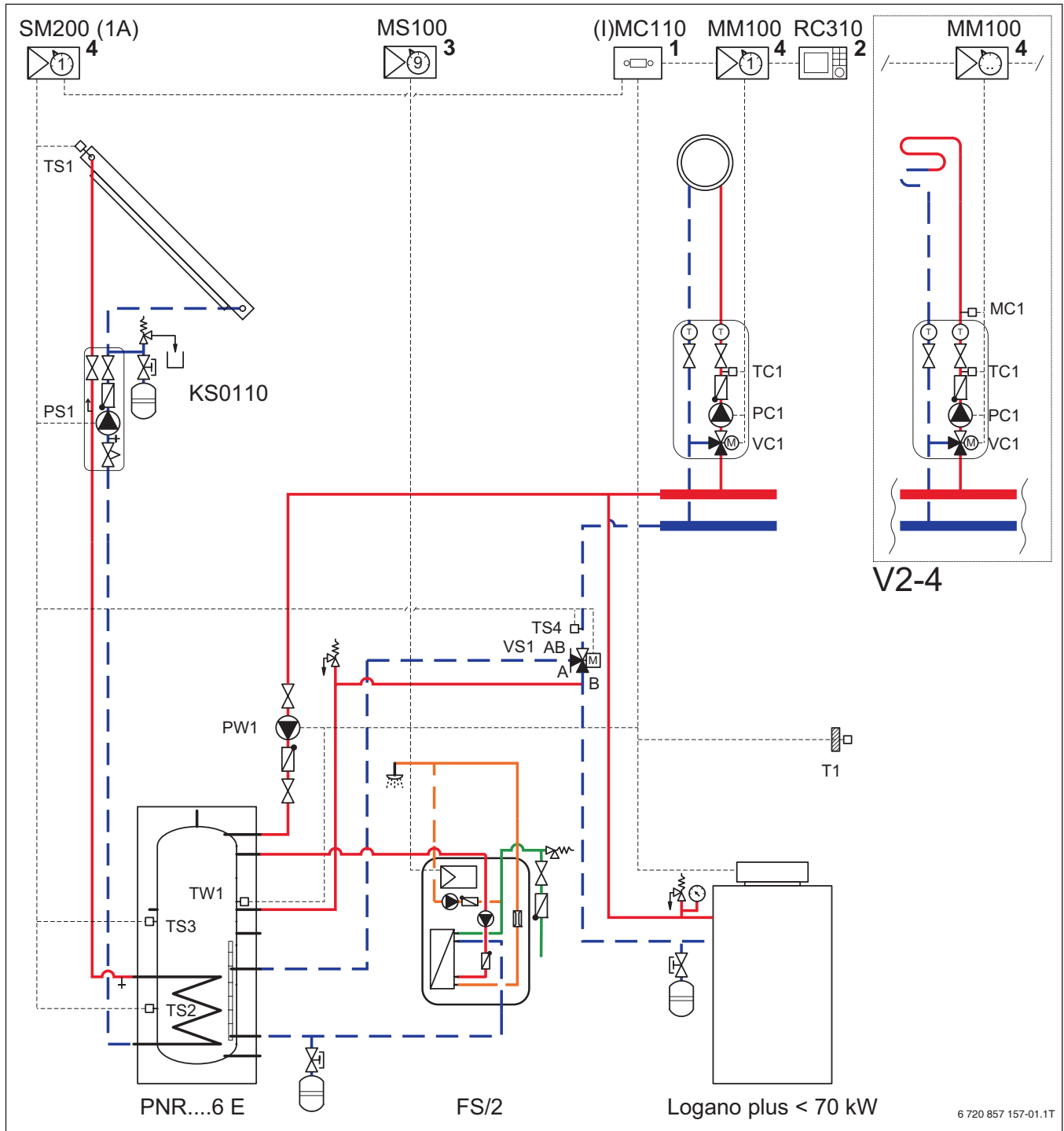
Bild 31 Anlagenbeispiel: Logano plus KB192i/GB212 mit einem gemischten Heizkreis, Frischwasserstation und Pufferspeicher Logalux PNR (Abkürzungsverzeichnis → S. 41)
