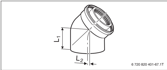
Bild 156 Konzentrischer Bogen Ø 60/100 (Maße → Tabelle 77)
