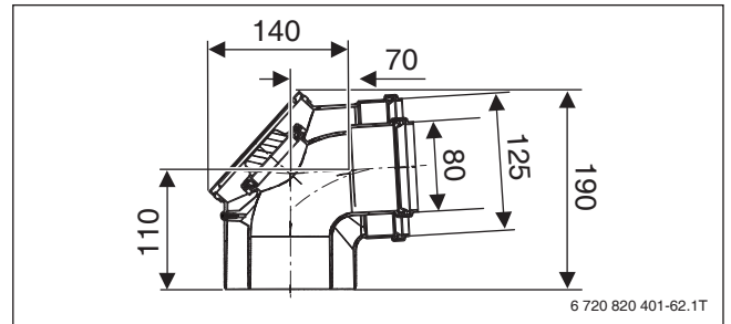
Bild 148 Konzentrischer Bogen mit Prüföffnung Ø 80/125 (Maße in mm)
