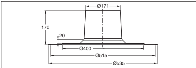
Bild 145 Flachdach-Klebeflansch für DN 110/160 (Maße in mm)
