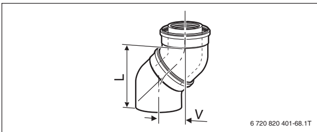
Bild 159 Versatzmaße konzentrischer Bogen Ø 60/100 (Maße → Tabelle 78)
