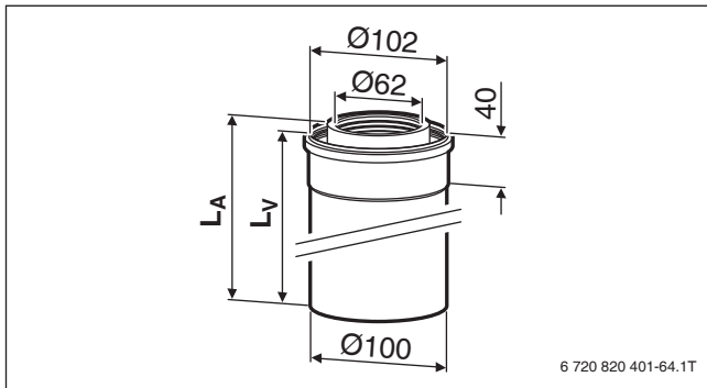
Bild 151 Konzentrisches Rohr \varnothing 60/100 (Maße in mm)
