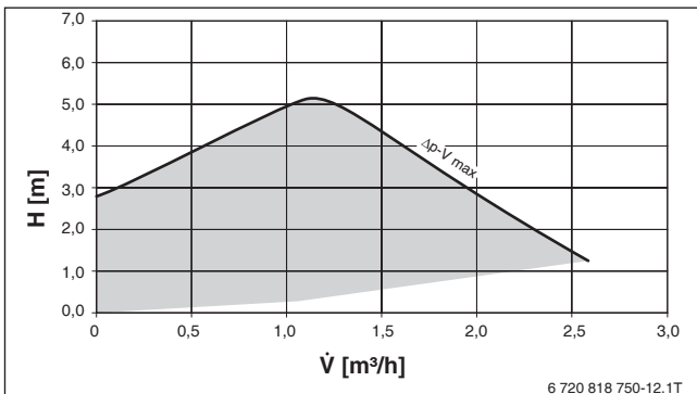
Bild 66 Restförderhöhe HS25/6 V3: \Delta p -V
