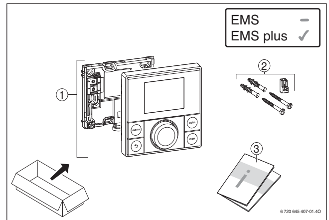
Bild 48 Lieferumfang
