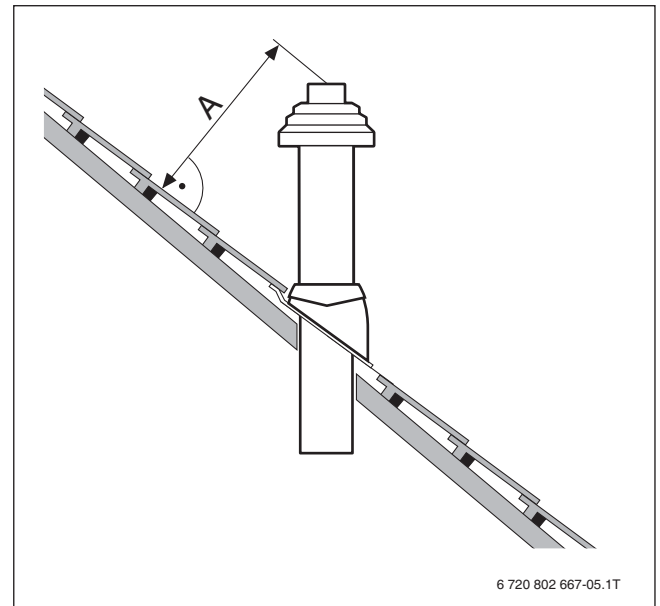
Bild 103 Mindestabstände Schrägdach
