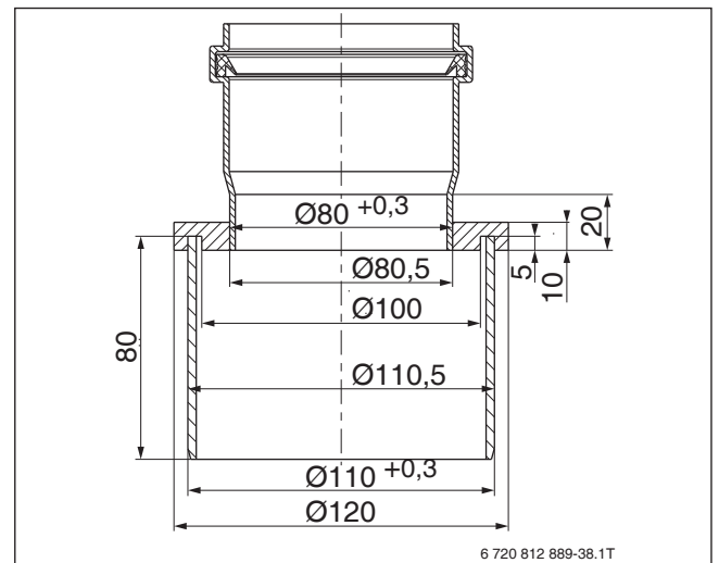
Bild 179 Zentrische Reduktion DN 110 auf DN 80
