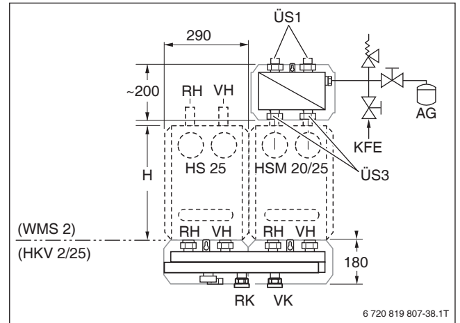
Bild 89 Abmessungen Anschluss-Set Wärmetauscher Systemtrennung mit Heizkreisanschluss-Set (Maße in mm)
