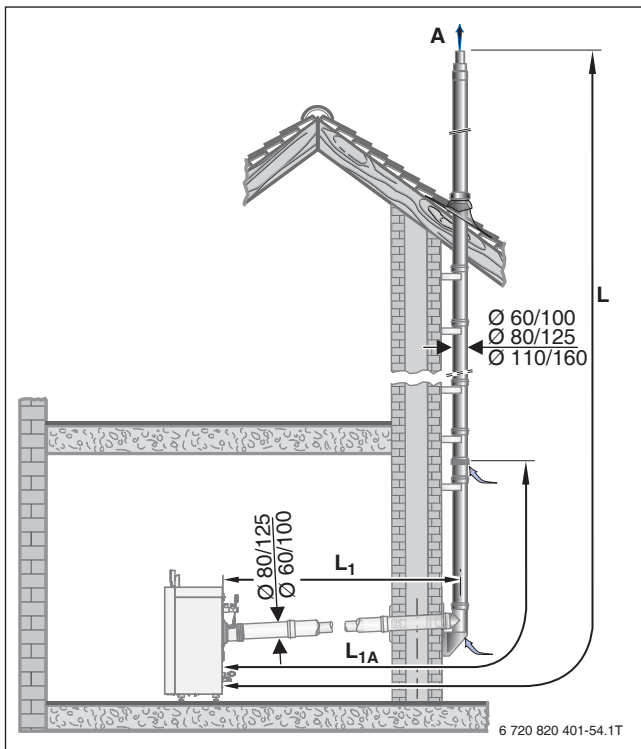
Bild 117 Montagevarianten mit dem Bausatz GAF-K
