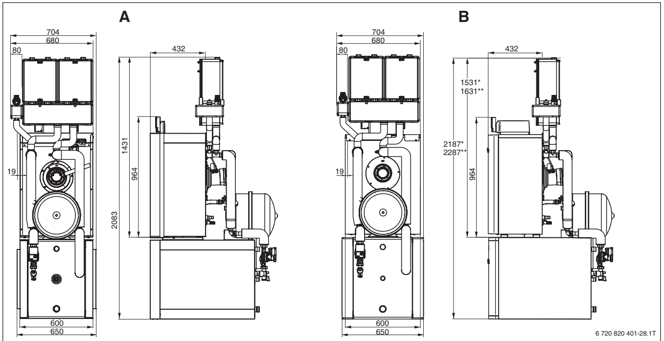
Bild 58 Abmessungen Logano plus KB192i/GB212 mit Logalux L.3RS bzw. Logalux L/2R und Heizkreisverteiler HKV 25 mit 2 Heizkreis-Anschluss-Sets (Maße in mm)
