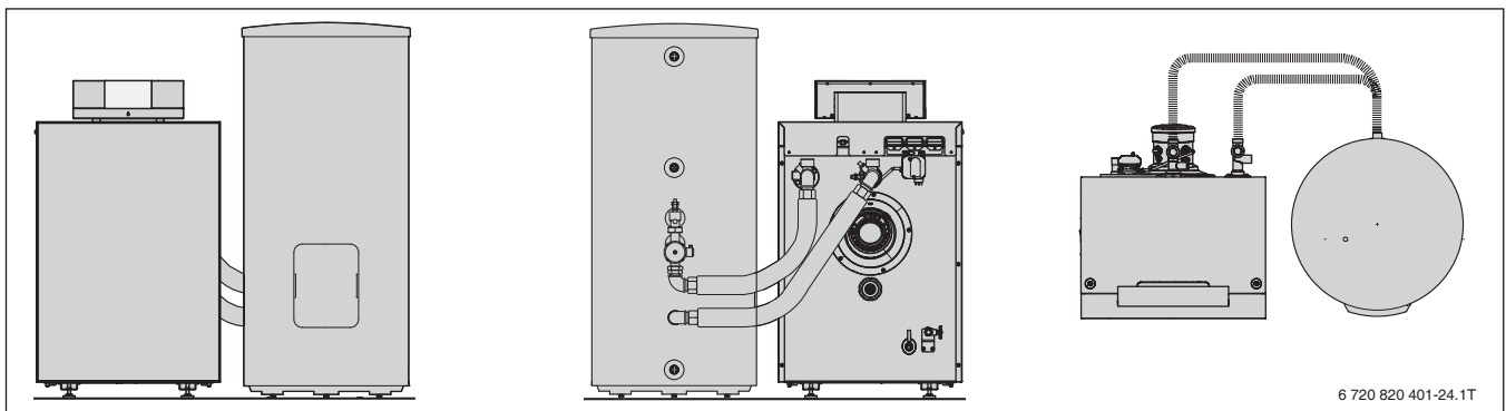
Bild 54 Logano plus KB192i mit Warmwasserspeicher Logalux SU
