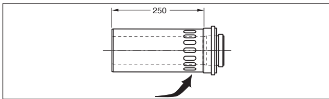
Bild 144 Zuluftgitter (Maße in mm)
