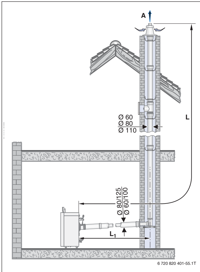
Bild 118 Montagevarianten mit dem Bausatz GA-K
