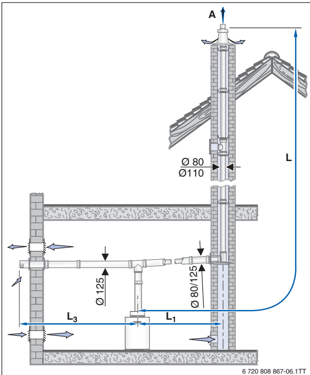
Bild 126 Montagevarianten mit dem Bausatz GA-K + GAL-K
