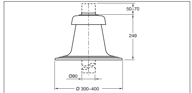
Bild 140 Schachtabdeckung für 80 mm (Maße in mm)
