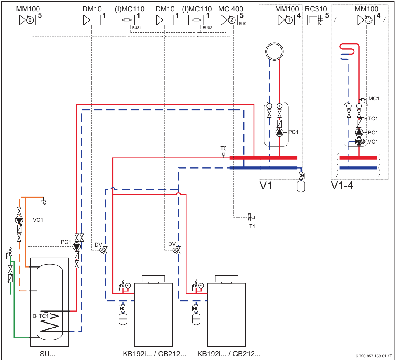
Bild 33 Anlagenbeispiel: 2 Logano plus KB192i/GB212 mit einem gemischten Heizkreis einem ungemischten Heizkreis und Warmwasserspeicher Logalux SU (Abkürzungsverzeichnis → S. 41)
