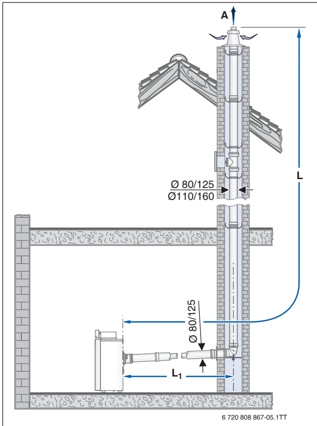
Bild 125 Montagevarianten mit dem Bausatz DO-S
