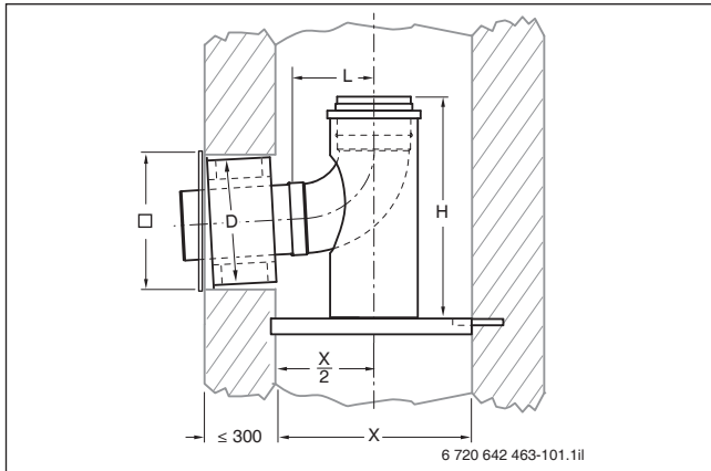
Bild 143 Schornsteinanschluss (Maße in mm)
