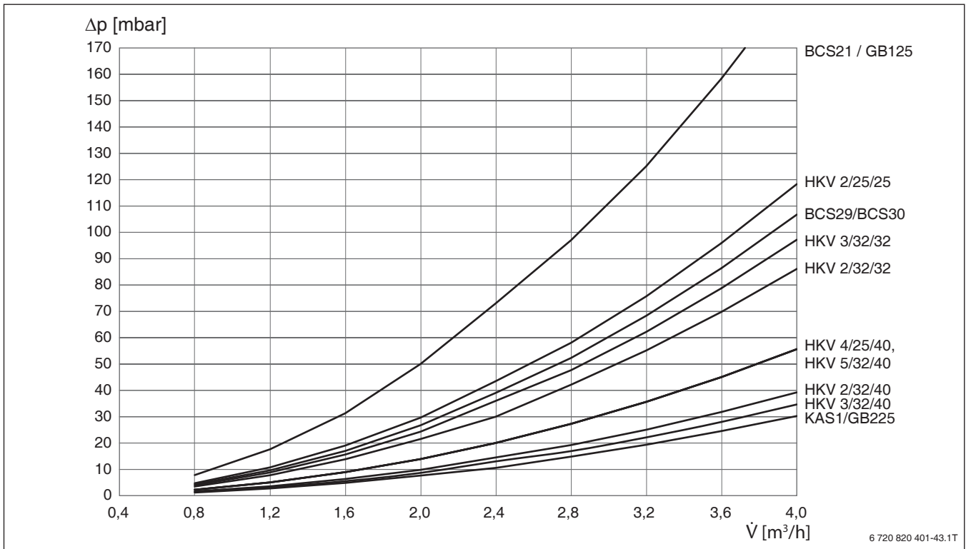
Bild 78 Wasserseitiger Durchflusswiderstand der Kesselanschluss-Sets und Heizkreisverteiler
