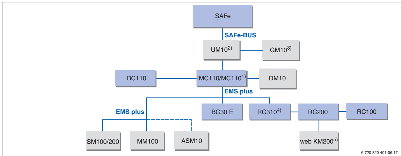
Bild 42 BUS-Aufbau und Prinzipdarstellung mit SAFe für Logano plus KB192i/GB212
