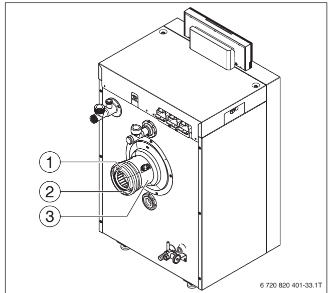
Bild 101 Abgasanschluss montieren Logano plus KB192i
