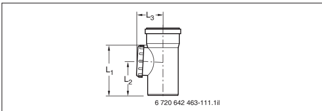
Bild 168 Rohr mit Prüföffnung
