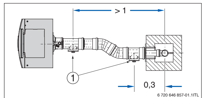
Bild 99 Beispiel zur Anordnung der Prüföffnungen bei einer waagerechten Abgasleitung mit Umlenkung im Aufstellraum – Draufsicht (Maße in m)
