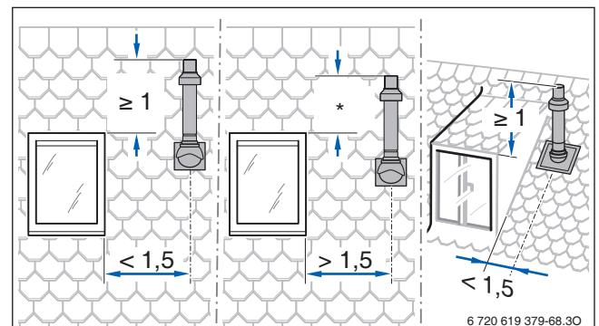
Bild 104 Mindestabstände zu Fenstern beim Bausatz DO (Beispiele nach der MuFeuVO); (Maße in m)
