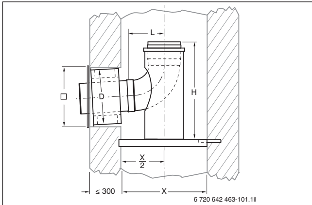
Bild 172 Schornsteinanschluss (Maße in mm)
