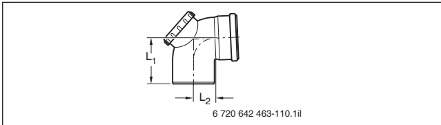
Bild 167 Bogen mit Prüföffnung
