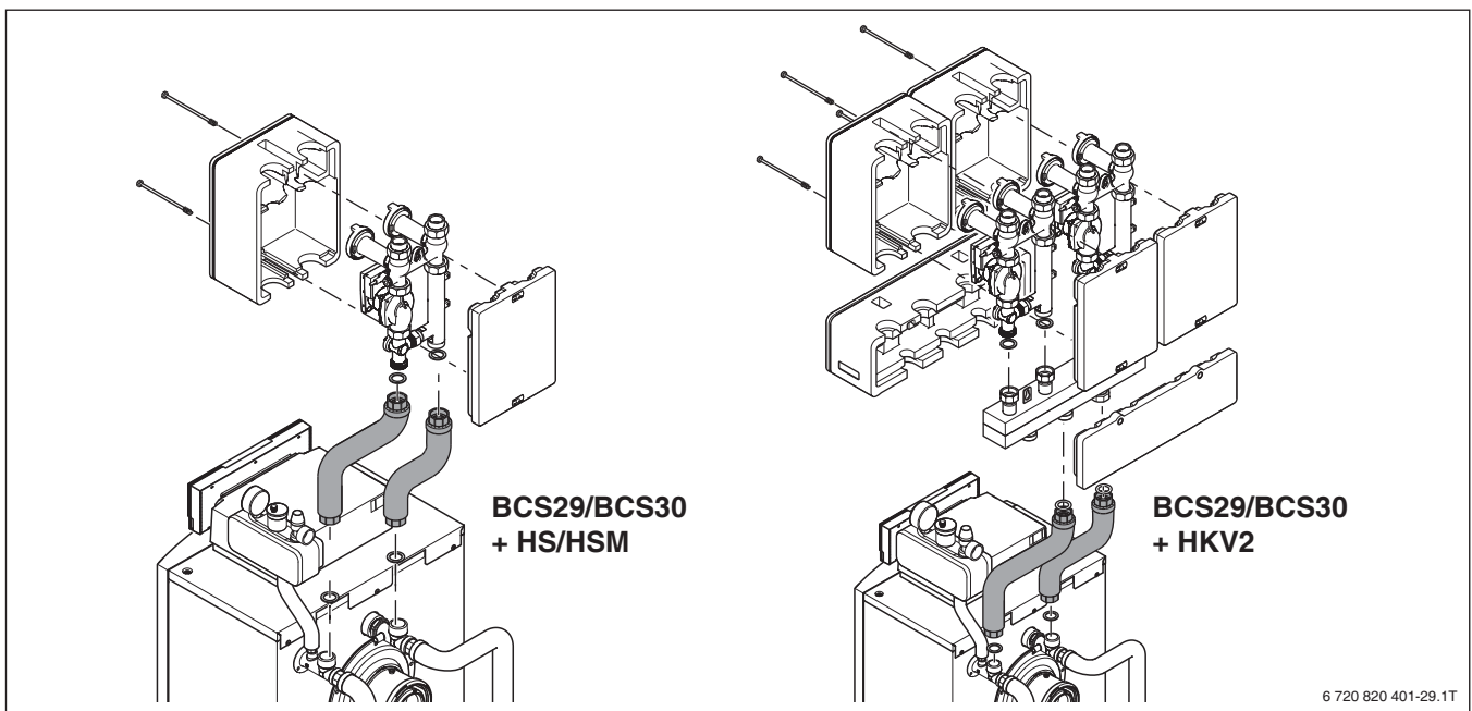
Bild 82 Kesselanschluss-Set BCS29/BCS30 Logano plus GB212 mit MC110
