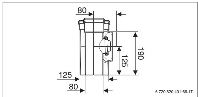
Bild 153 Konzentrisches Rohr mit Prüföffnung \varnothing 80/125 (Maße in mm)
