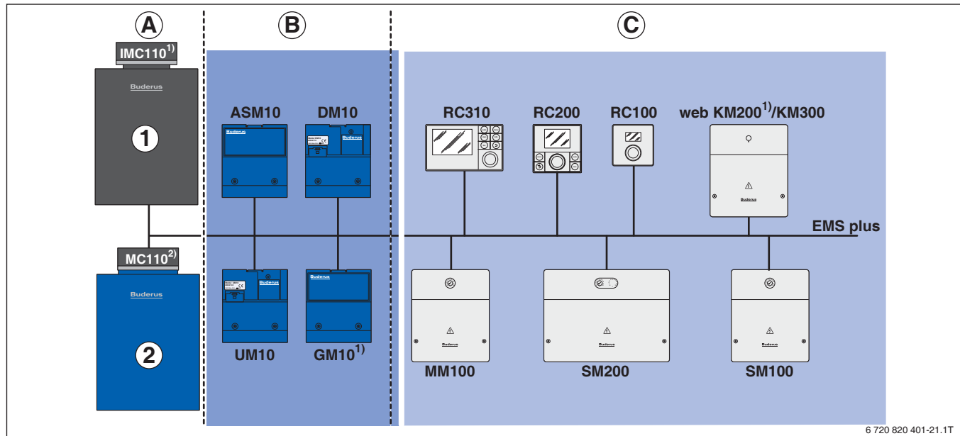
Bild 52 Aufbau modulares Regelsystem Logamatic EMS plus
