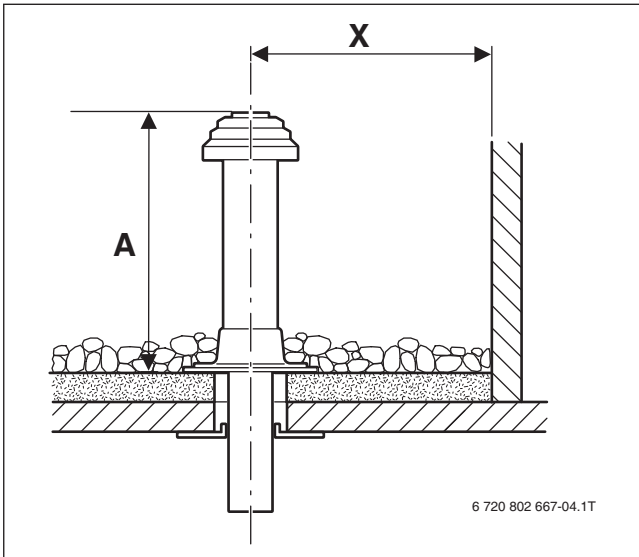
Bild 102 Mindestabstände Flachdach
