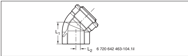
Bild 157 Konzentrischer Bogen Ø 80/125 (Maße → Tabelle 77)
