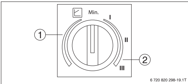
Bild 61 Einstellmöglichkeiten Umwälzpumpe
