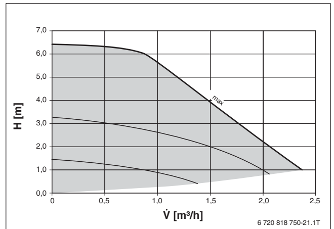
Bild 75 Restförderhöhe HSM25 V3: Konstant
