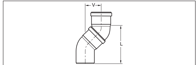
Bild 133 Versatzmaße Bogen
