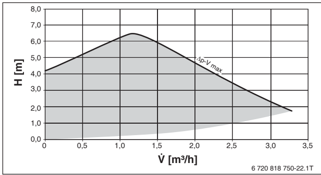
Bild 76 Restförderhöhe HSM32 V3: \Delta p -V
