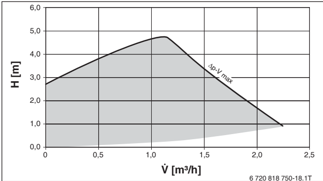
Bild 72 Restförderhöhe HSM20 V3: \Delta p -V
