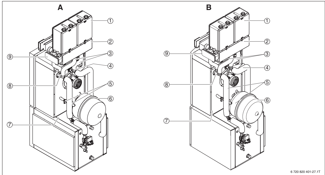
Bild 57 Heizkreis-Schnellmontage-Systeme zur Heizkesselmontage – Logano plus KB192i/GB212
