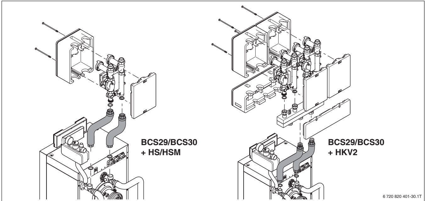
Bild 81 Kesselanschluss-Set BCS29/BCS30 Logano plus KB192i mit IMC110
