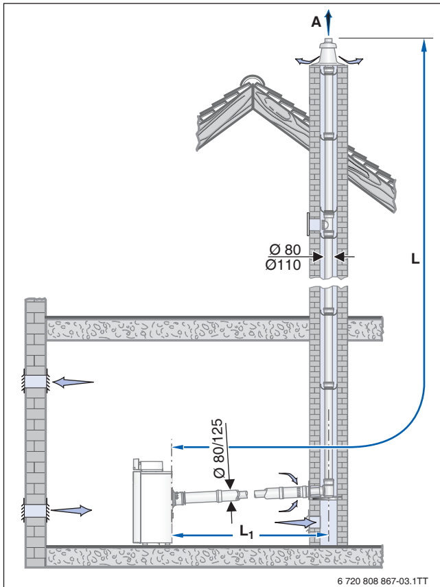
Bild 122 Montagevariante mit dem Bausatz GA-X + GA-K
