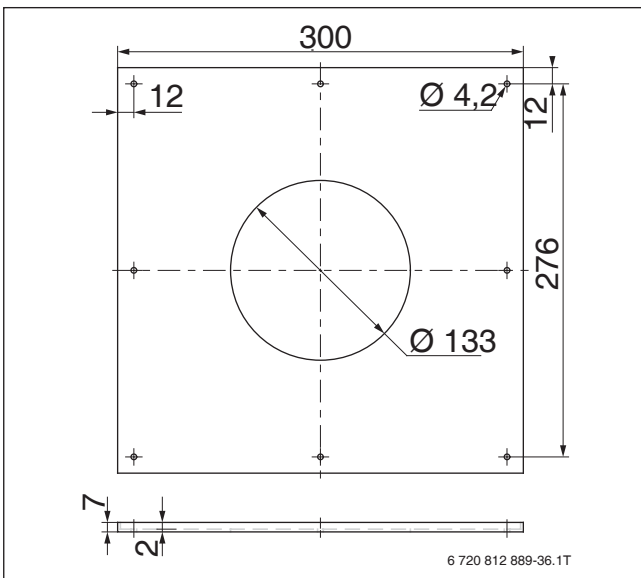
Bild 177 Blende groß; zur Installation als Deckenhalterung
