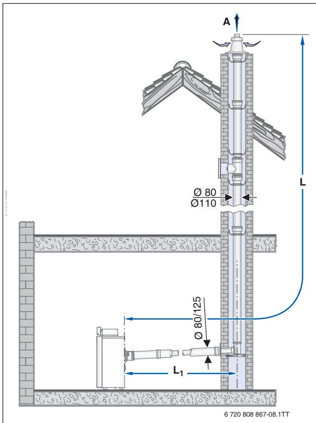
Bild 128 Montagevarianten mit dem Bausatz GA-K
