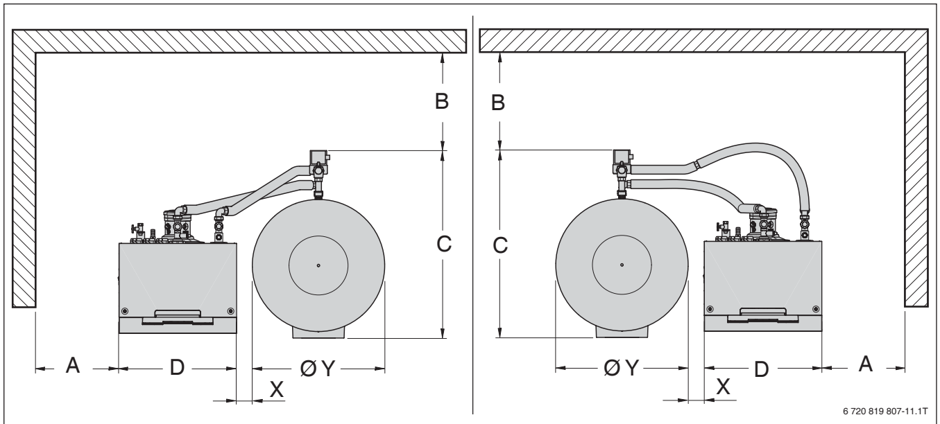
Bild 23 Wandabstände im Aufstellraum
