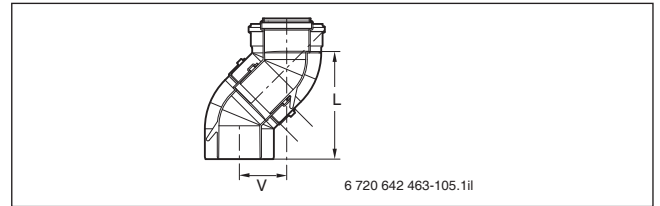
Bild 160 Versatzmaße konzentrischer Bogen Ø 80/125 (Maße → Tabelle 78)
