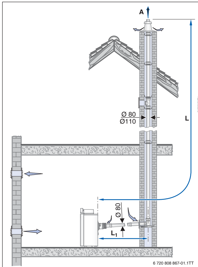
Bild 120 Montagevariante mit dem Bausatz GA
