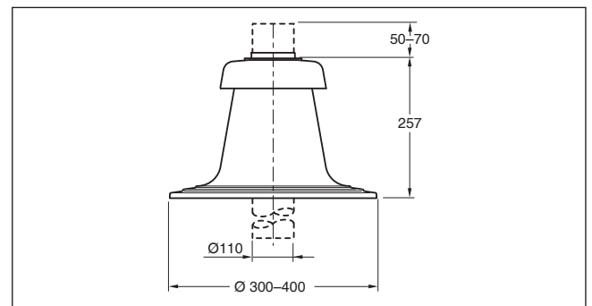
Bild 141 Schachtabdeckung für 110 mm (Maße in mm)
