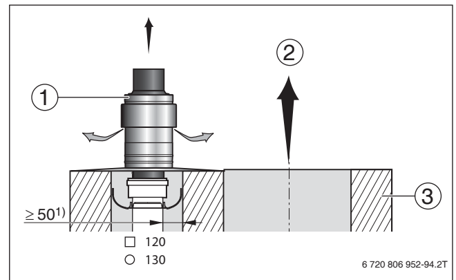
Bild 108 Mindestmaße des Schachtquerschnitts und der Schachtmündung in Verbindung mit Feuerstätten für feste Brennstoffe (Maße in mm)
