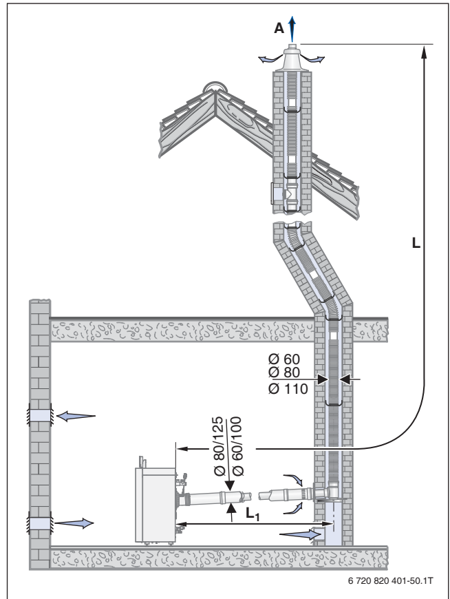
Bild 113 Montagevariante mit dem Bausatz GA-X + GA-K + ÜB-Flex
