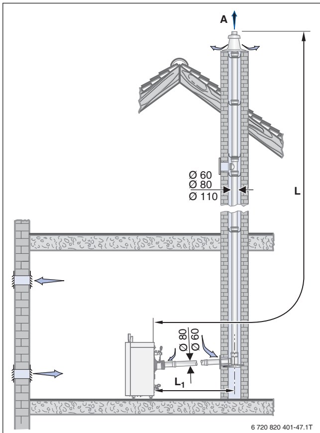
Bild 110 Montagevariante mit dem Bausatz GA
