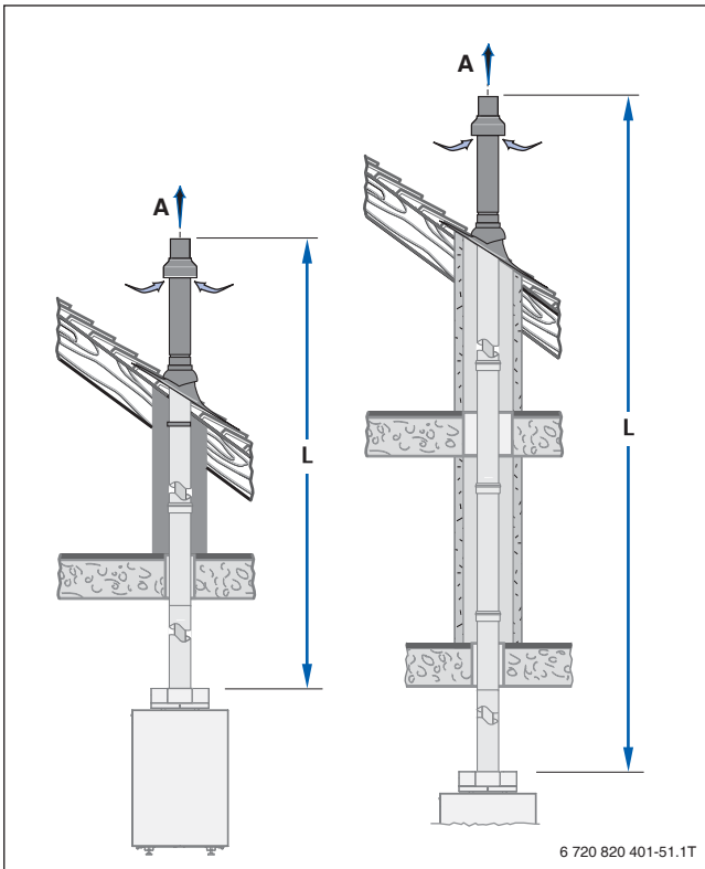
Bild 114 Montagevarianten mit dem Bausatz DO
