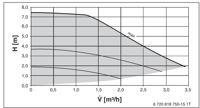
Bild 69 Restförderhöhe HS32 V3: Konstant
