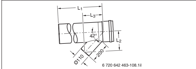
Bild 173 Abgassammler (Maße in mm)
