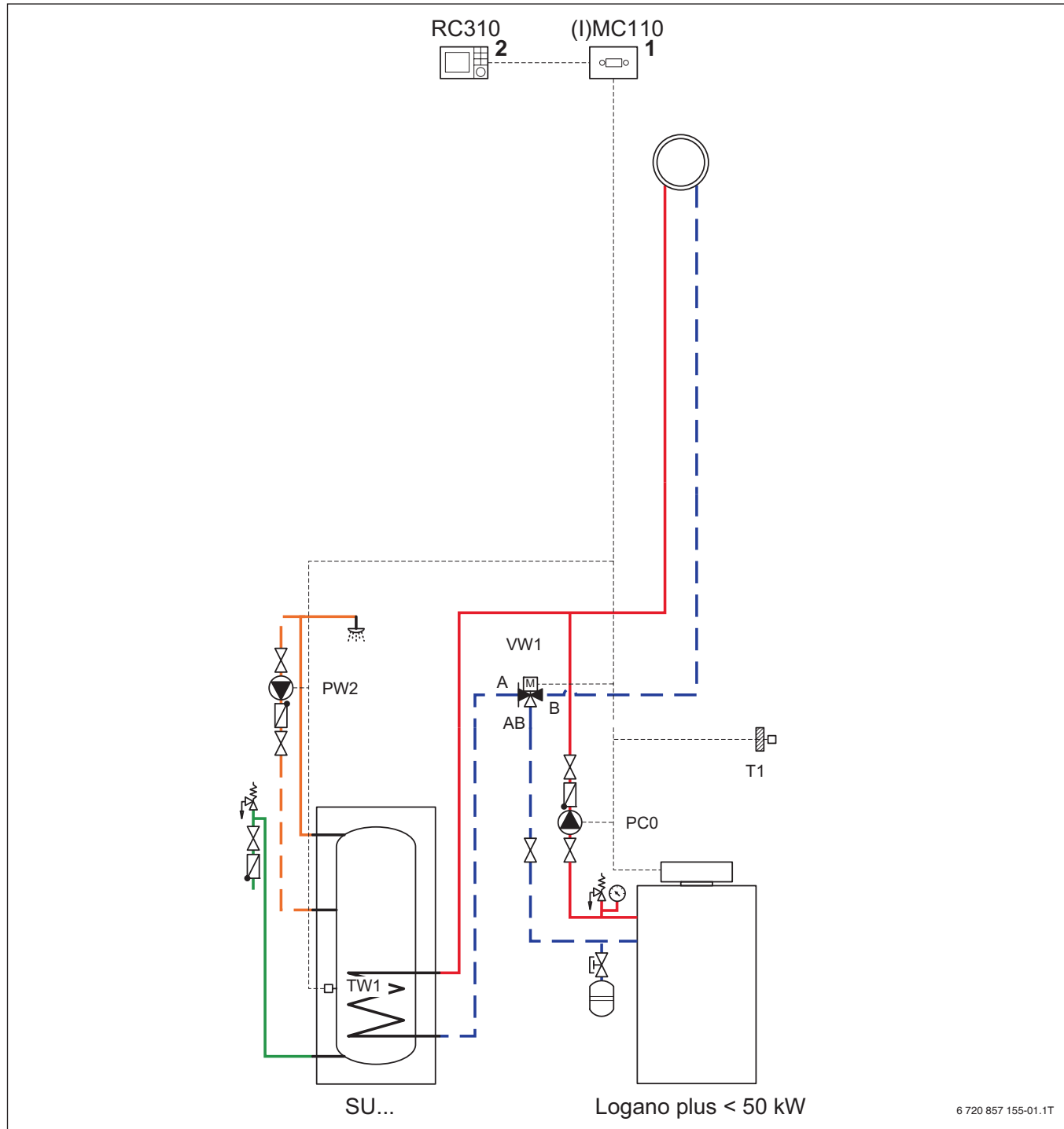
Bild 27 Anlagenbeispiel: Logano plus KB192i/GB212 mit einem ungemischten Heizkreis und Warmwasserspeicher Logalux SU (Abkürzungsverzeichnis → S. 41)
