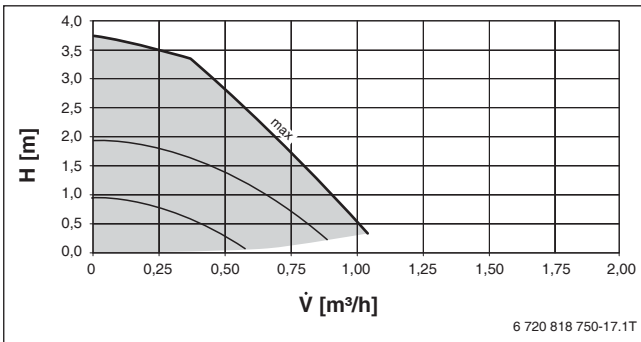
Bild 71 Restförderhöhe HSM15 V3: Konstant
