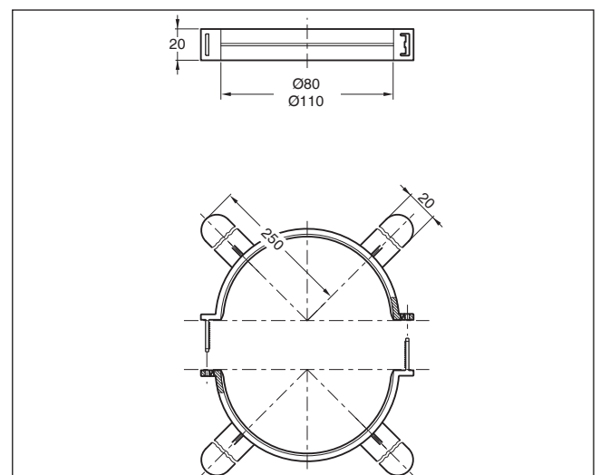
Bild 142 Abstandshalter für Abgasleitung im Schacht (Maße in mm)
