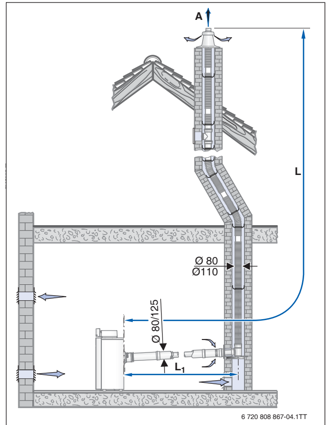
Bild 123 Montagevariante mit dem Bausatz GA-X + GA-K + ÜB-Flex
