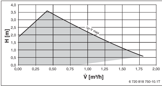
Bild 64 Restförderhöhe HS25/4 V3: \Delta p -V
