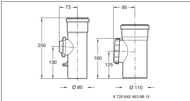
Bild 131 Rohr mit Prüföffnung (Maße in mm)
