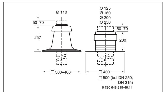
Bild 170 Schachtabdeckung (Maße in mm)
