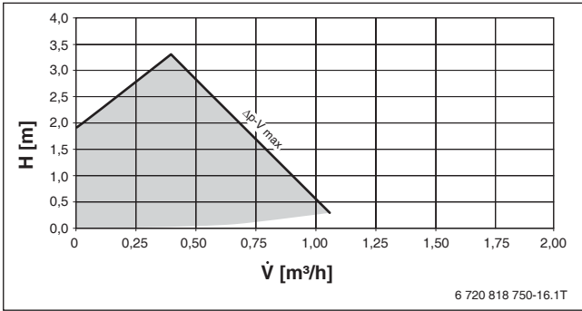
Bild 70 Restförderhöhe HSM15 V3: \Delta p -V
