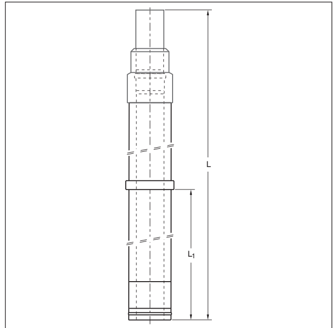
Bild 165 Dachdurchführung mit Mündungsabschluss
