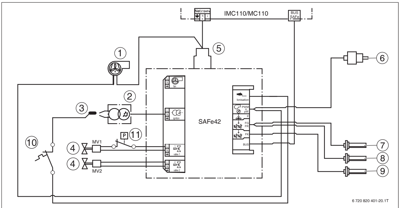
Bild 37 Anschlussplan Feuerungsautomat (50 kW)
