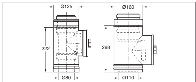
Bild 155 Konzentrisches Rohr mit Prüföffnung aus Edelstahl (Maße in mm)
