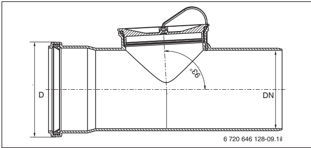
Bild 176 Muffenmaße Abgasrohre
