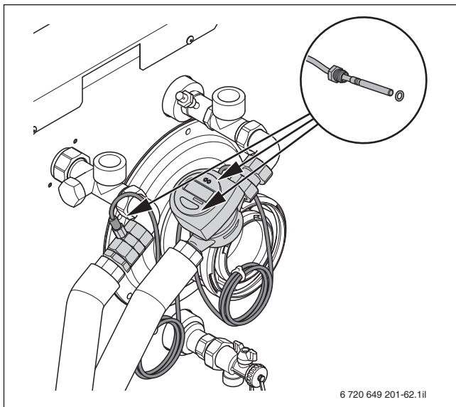
Bild 85 Einbauposition Anschluss-Set Wärmemengenzähler
