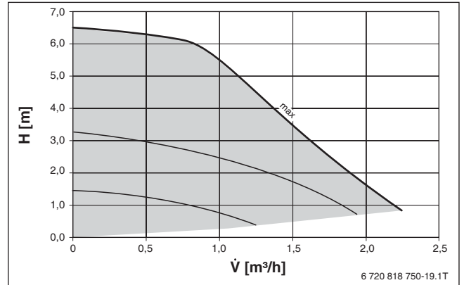
Bild 73 Restförderhöhe HSM20 V3: Konstant
