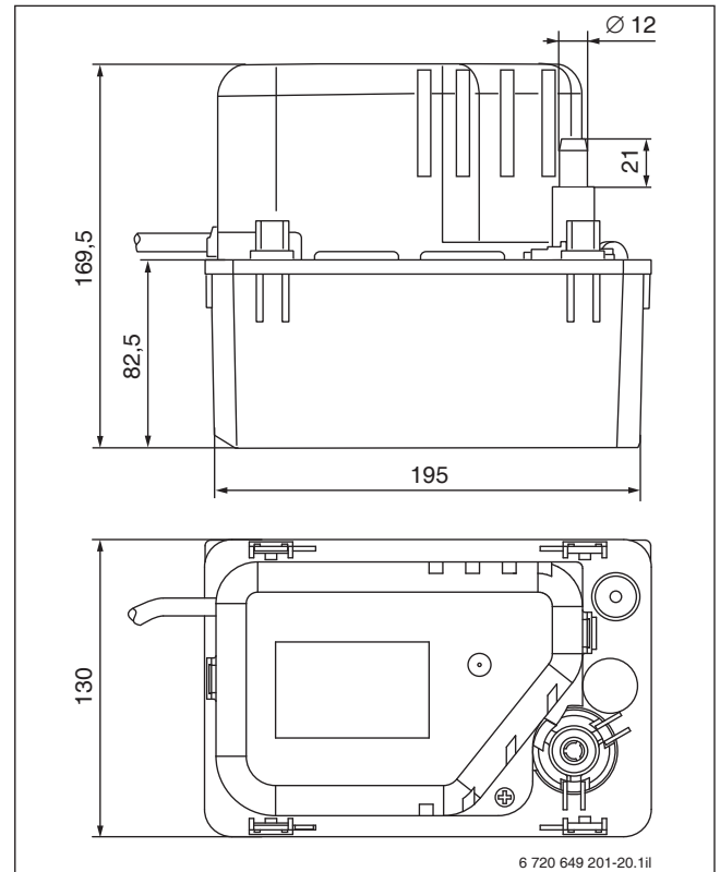
Bild 93 Abmessungen Kondensathebeanlage Wilo-DrainLift Con (Maße in mm)
