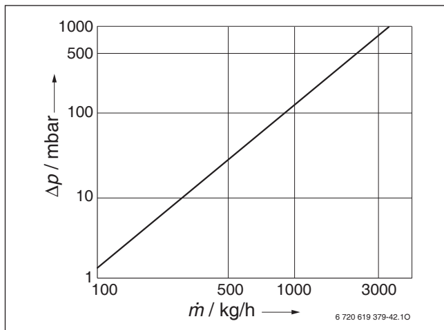
Bild 90 Druckverlust des Anschluss-Sets Wärmetauscher Systemtrennung
