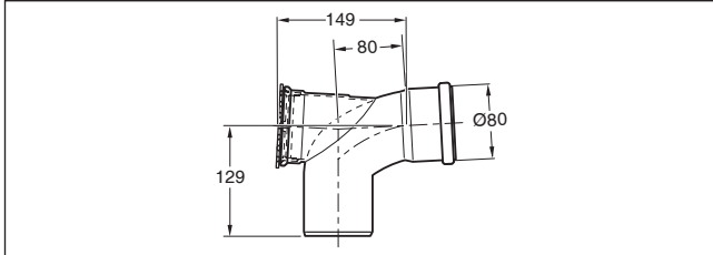
Bild 130 Bogen mit Prüföffnung lang (Maße in mm)
