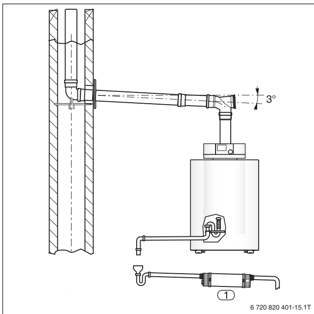
Bild 91 Kondensatableitung aus dem Gas-Brennwertkessel und einer Abgasleitung über den Neutralisator
