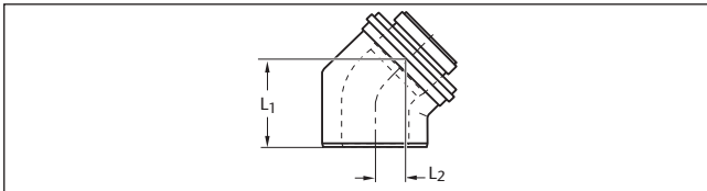
Bild 158 Konzentrischer Bogen Ø 110/160 (Maße → Tabelle 77)
