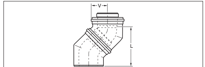
Bild 161 Versatzmaße konzentrischer Bogen Ø 110/160 (Maße → Tabelle 78)
