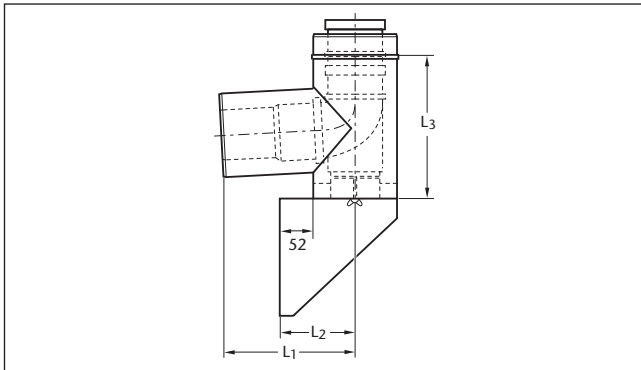
Bild 163 Konzentrisches Zuluft-T-Stück (Maße → Tabelle 80)
