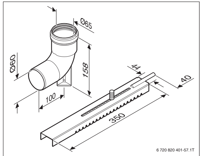
Bild 134 Stützbogen mit Auflageschiene für Ø 60 mm (Maße in mm)
