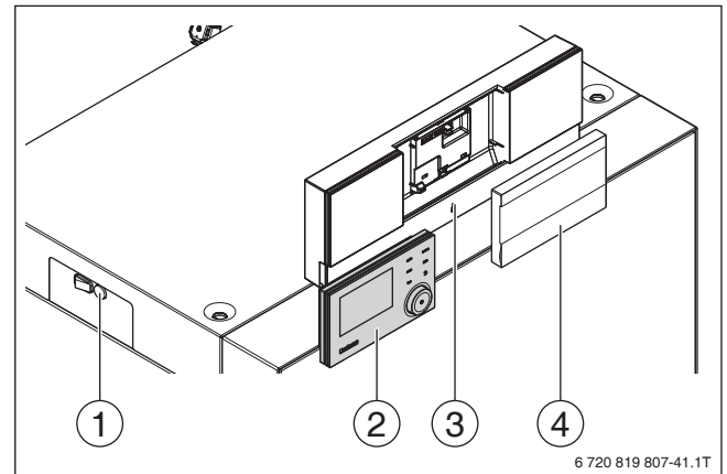
Bild 41 Logamatic IMC110/MC110
