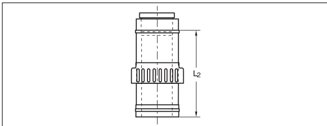
Bild 164 Konzentrischer Zuluftstutzen
