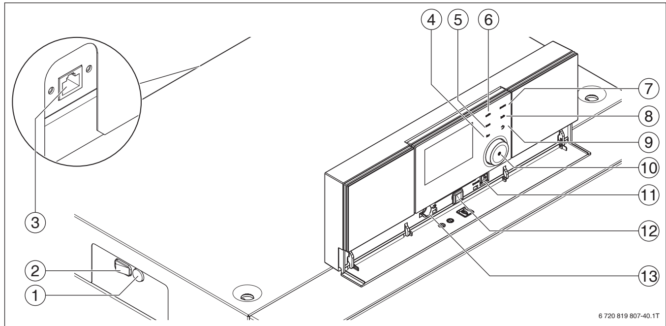
Bild 38 Mastercontroller IMC110 mit Basiscontroller Logamatic BC110 mit eingeklippter Bedieneinheit RC310 – Bedienelemente
