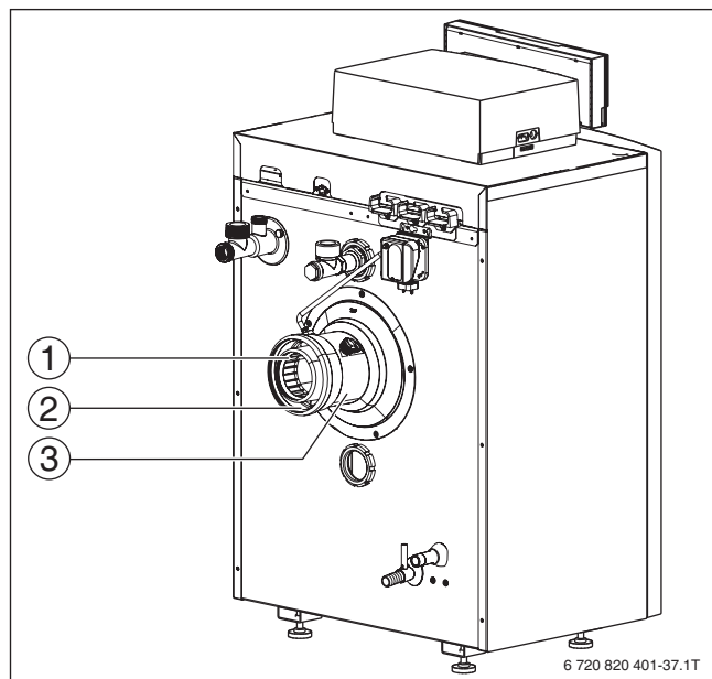
Bild 100 Abgasanschluss montieren Logano plus GB212
