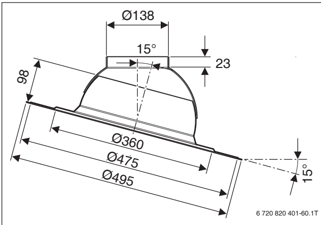
Bild 146 Flachdach-Klebeflansch für DN 80/125 (Maße in mm)
