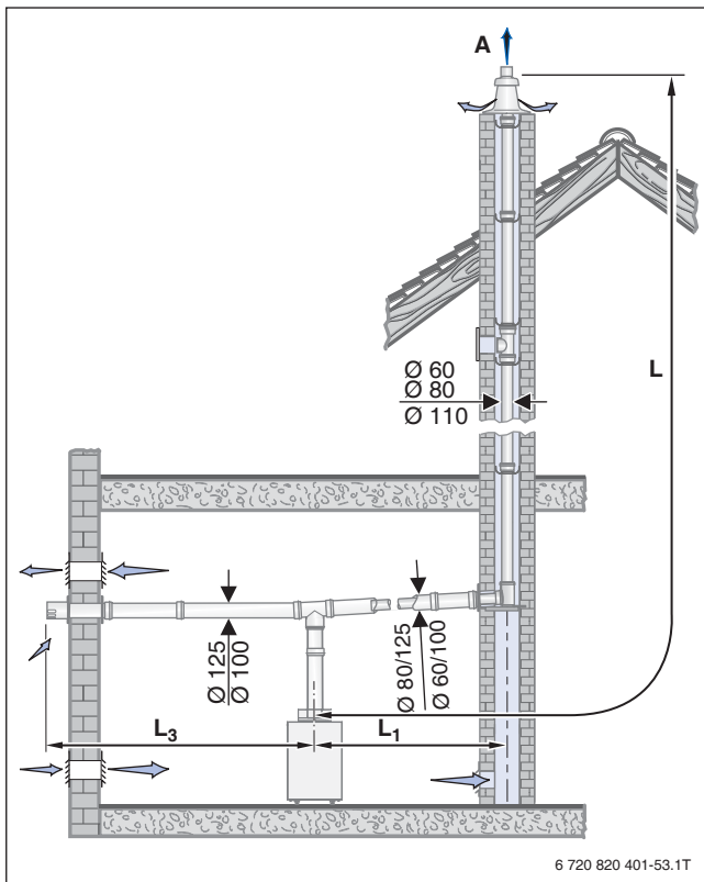
Bild 116 Montagevarianten mit dem Bausatz GA-K + GAL-K
