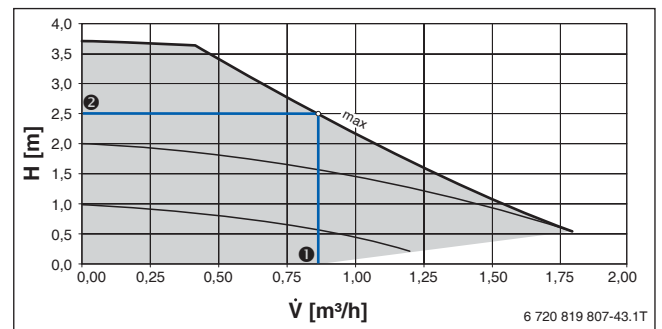
Bild 63 Restförderhöhe HS25/4 V3: Konstant
