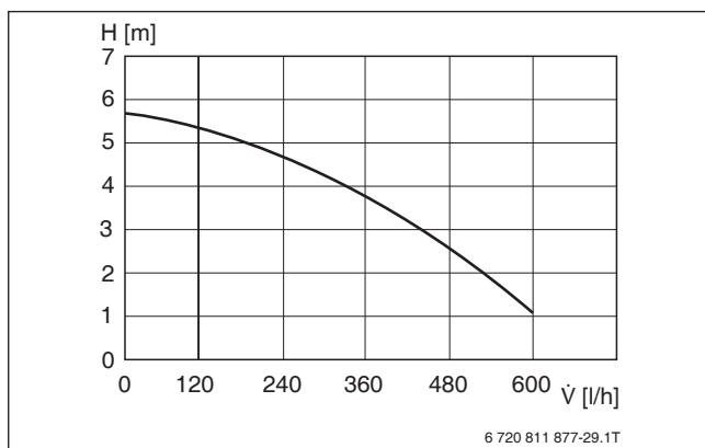
Bild 92 Leistungsdiagramm Wilo-DrainLift Con
