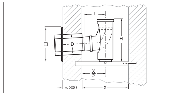
Bild 162 Konzentrischer Schornsteinanschluss (Maße in mm)
