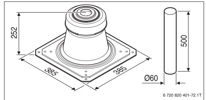
Bild 139 Schachtabdeckung für 60 mm, Kunststoff (Maße in mm)
