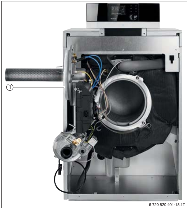
Bild 34 Gas-Vormischbrenner Logano plus KB192i
