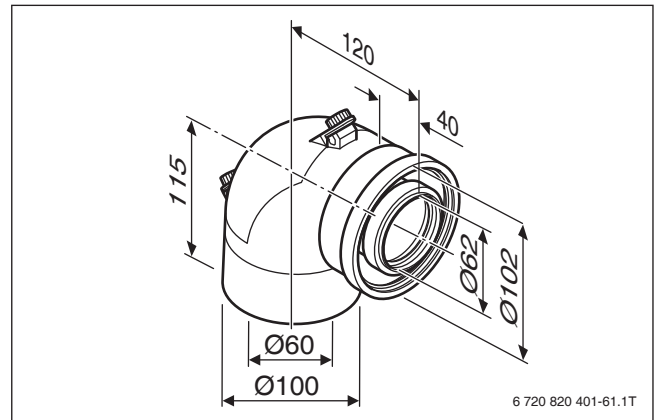
Bild 147 Konzentrischer Bogen mit Prüföffnung Ø 60/100 (Maße in mm)
