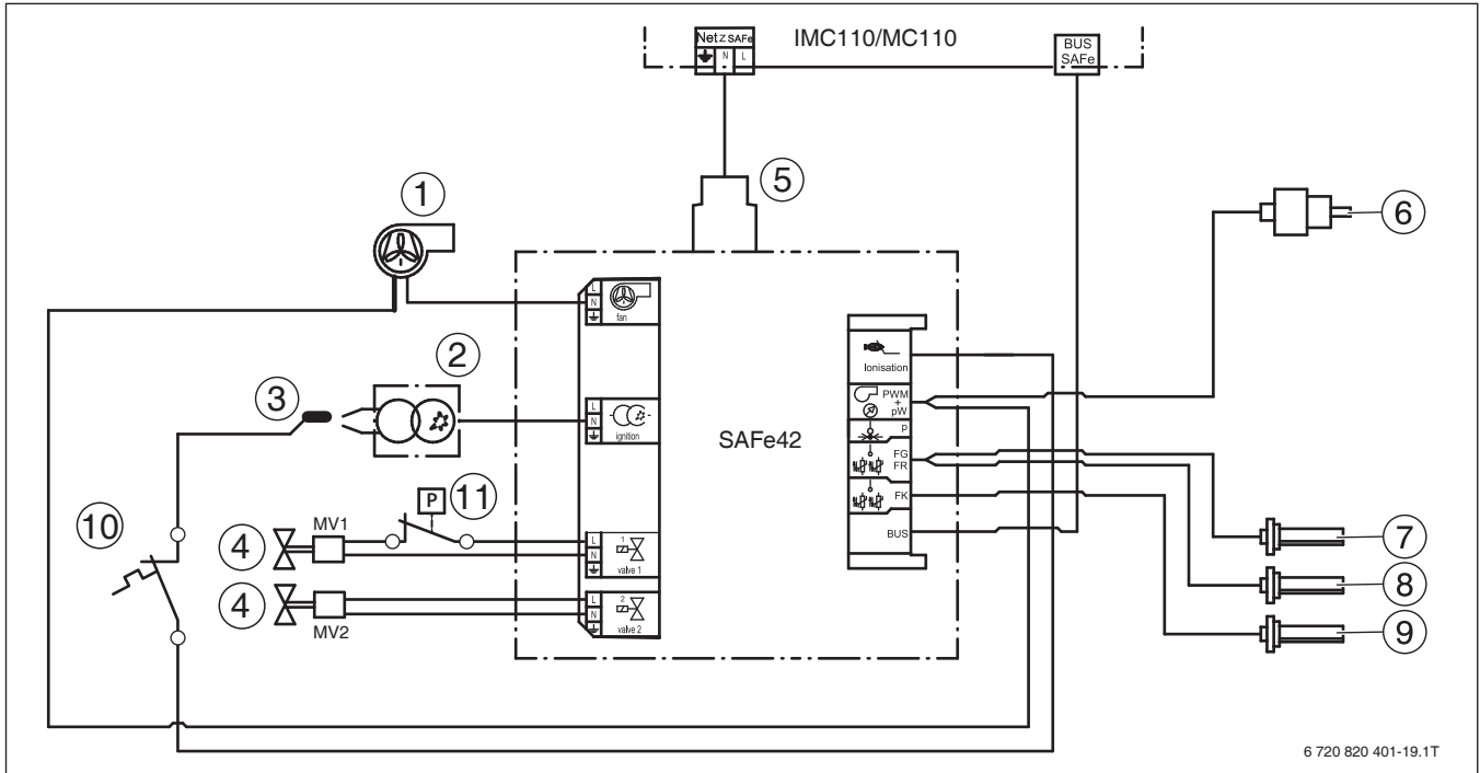
Bild 36 Anschlussplan Feuerungsautomat (15 ... 40 kW)
