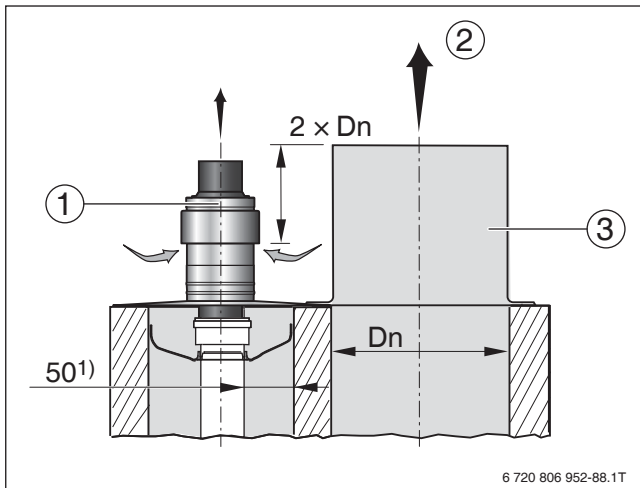
Bild 107 Schachtmündung für die Abgasleitung des Bausatzes GA-K in Verbindung mit Feuerstätten für feste Brennstoffe (Maße in mm)
