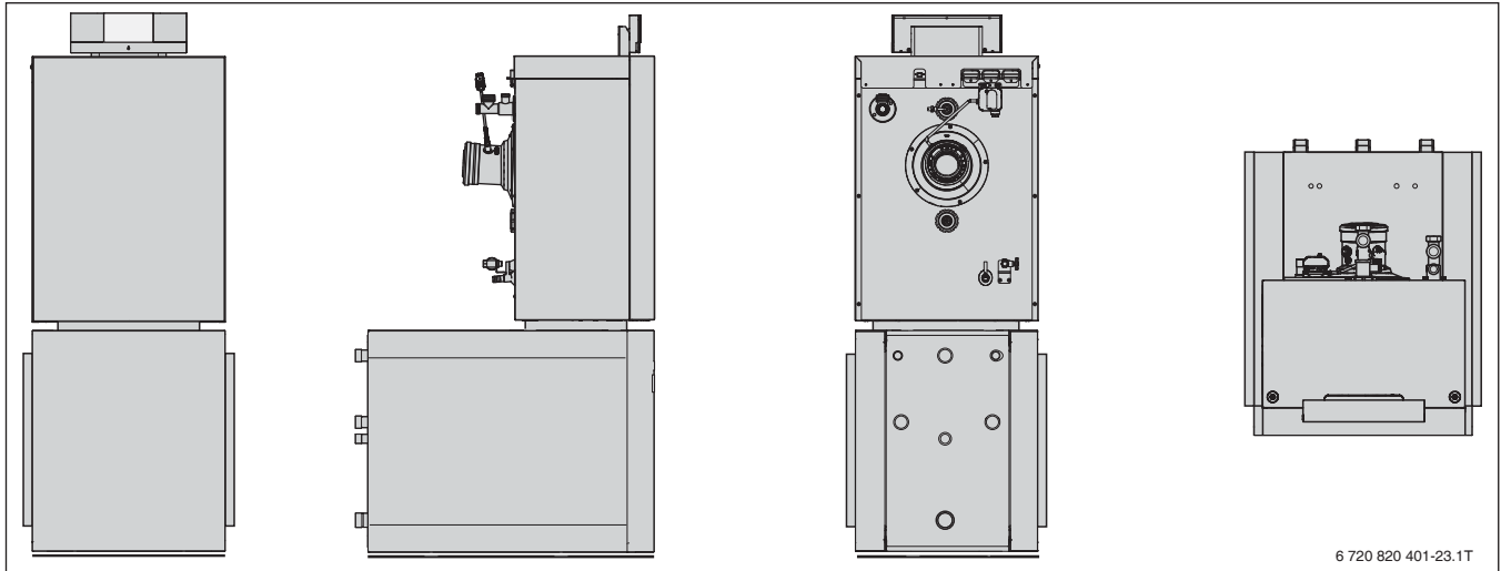
Bild 53 Logano plus KB192i mit Warmwasserspeicher Logalux L.3RS
