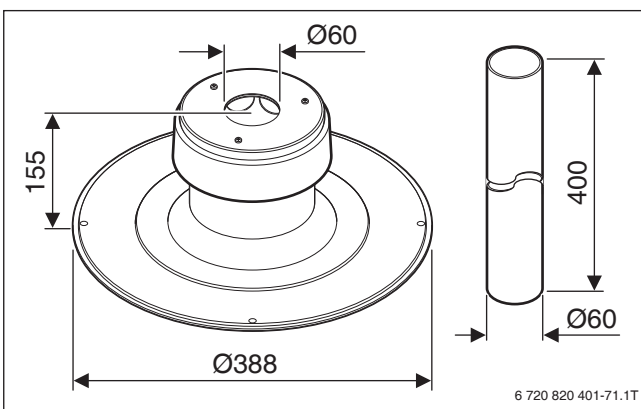
Bild 138 Schachtabdeckung für 60 mm, Aluminium (Maße in mm)
