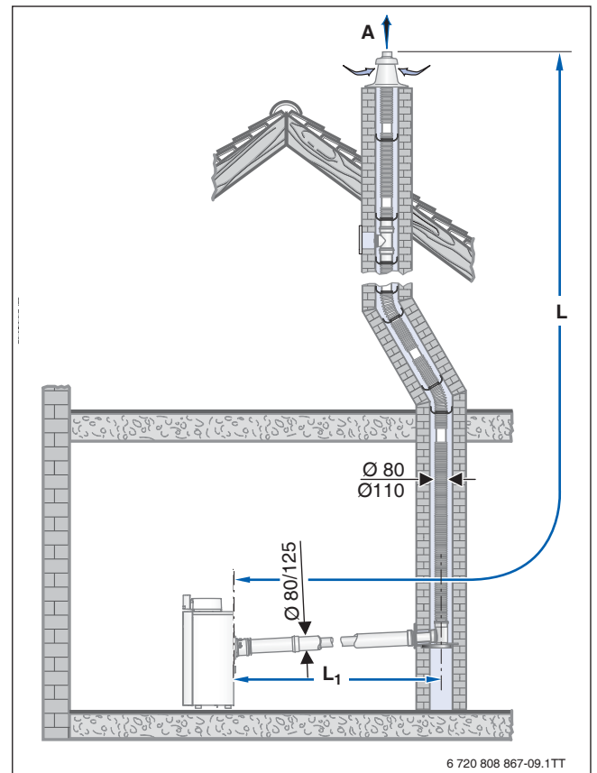
Bild 129 Montagevarianten mit dem Bausatz GA-K + ÜB-Flex
