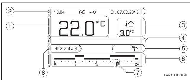
Bild 45 Beispiel für die Standardanzeige System-Bedieneinheit RC310
