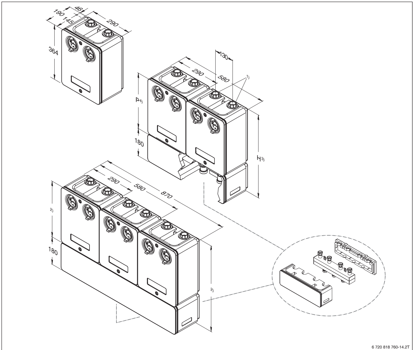
Bild 59 Heizkreis-Schnellmontage-Systeme zur Wandinstallation
