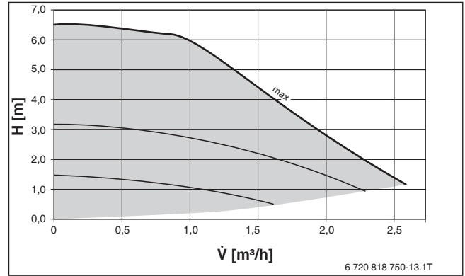
Bild 67 Restförderhöhe HS25/6 V3: Konstant
