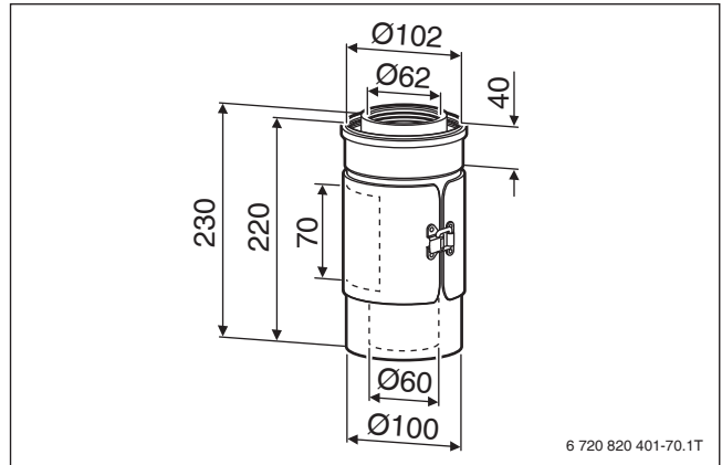
Bild 152 Konzentrisches Rohr mit Prüföffnung \varnothing 60/100 (Maße in mm)
