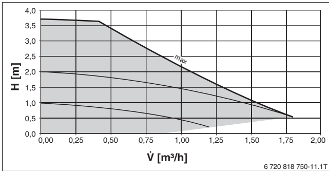
Bild 65 Restförderhöhe HS25/4 V3: Konstant
