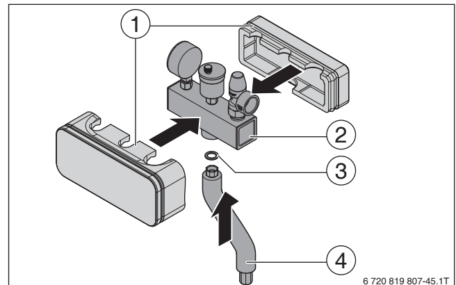
Bild 86 Kesselsicherheits-Set
