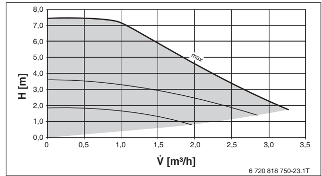
Bild 77 Restförderhöhe HSM32 V3: Konstant
