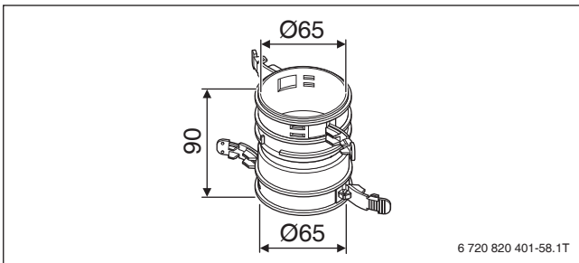
Bild 136 Verbindungsstück Flex Ø 60 mm (Maße in mm)
