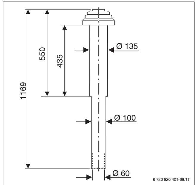
Bild 166 Dachdurchführung Ø 60/100 (Maße in mm)
