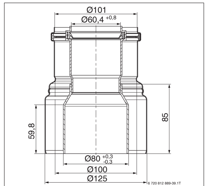
Bild 180 Konzentrische Reduktion DN 80/125 auf DN 60/100
