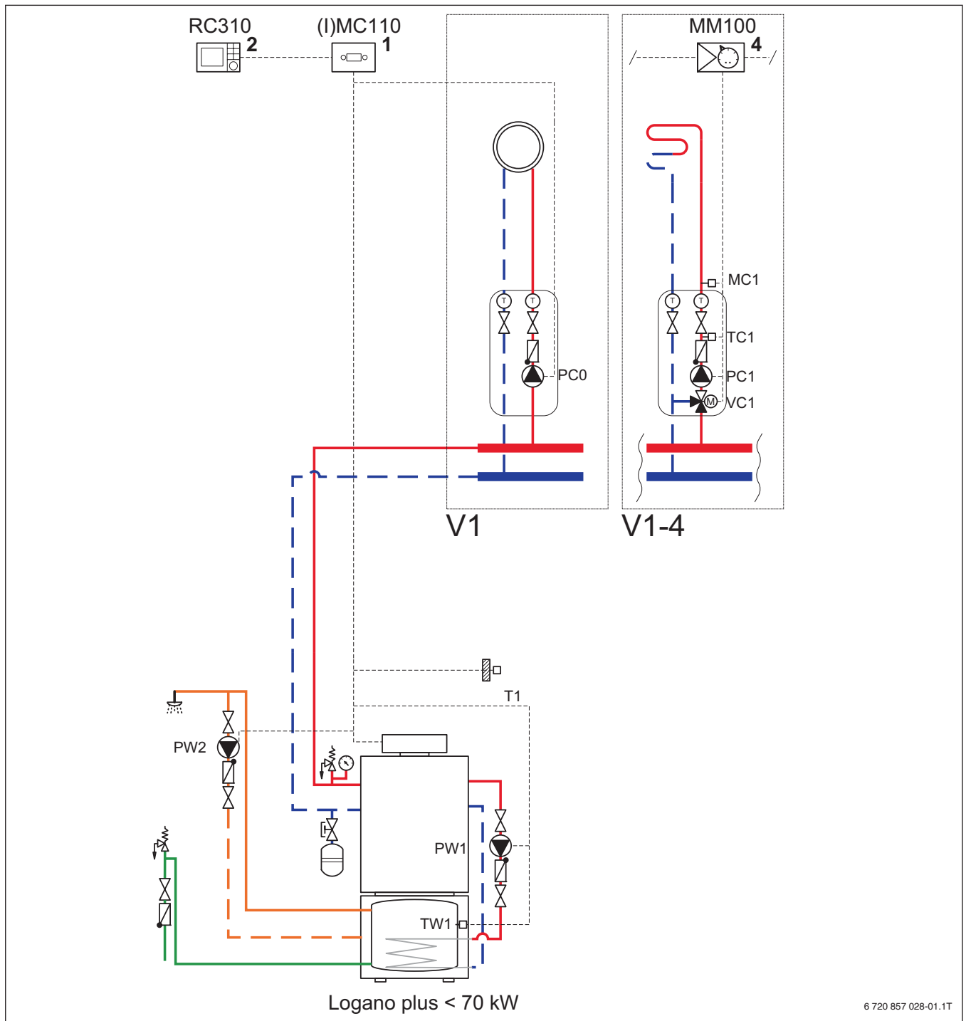
Bild 28 Anlagenbeispiel: Logano plus KB192i/GB212 mit Warmwasserspeicher Logalux L.3RS, L/2R und einem gemischten Heizkreis (Abkürzungsverzeichnis → S. 41)
