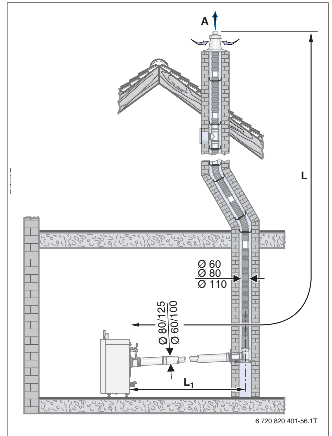
Bild 119 Montagevarianten mit dem Bausatz GA-K + ÜB-Flex
