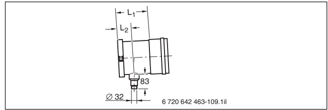
Bild 174 Endstück mit Kondensatablauf (Maße in mm)
