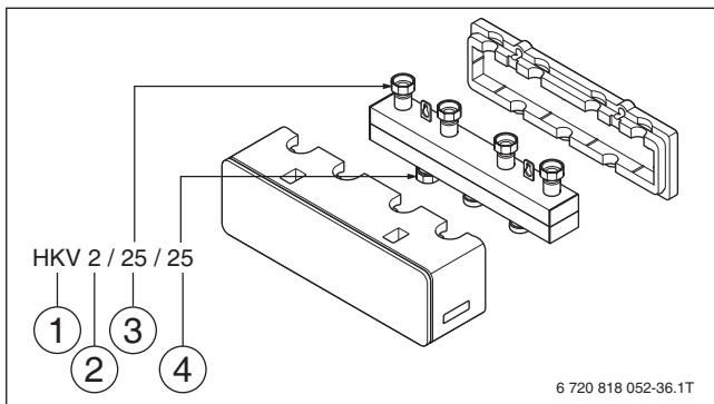
Bild 83 Heizkreisverteiler HKV
