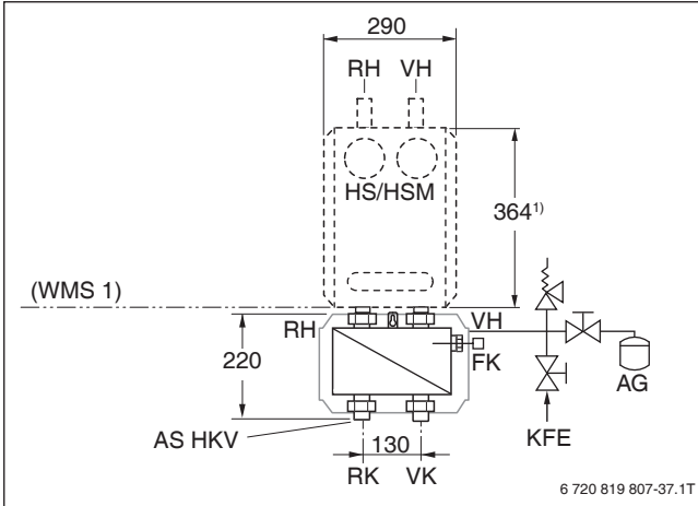
Bild 88 Abmessungen Anschluss-Set Wärmetauscher Systemtrennung mit Heizkreisanschluss-Set (Maße in mm)
