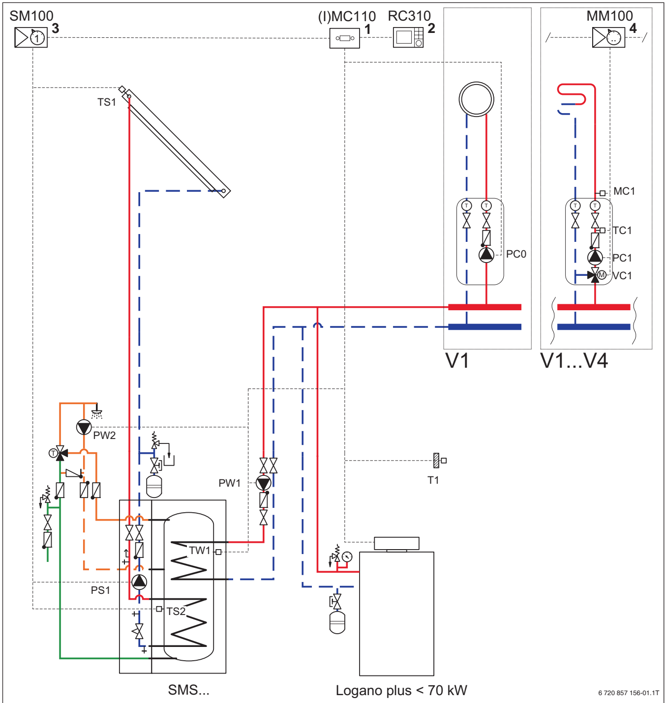
Bild 29 Anlagenbeispiel: Logano plus KB192i/GB212 mit einem ungemischten Heizkreis und Solarspeicher Logalux SMS (Abkürzungsverzeichnis → S. 41)
