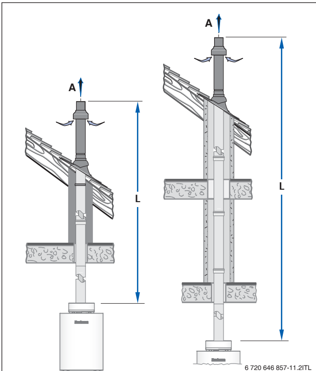
Bild 124 Montagevarianten mit dem Bausatz DO
