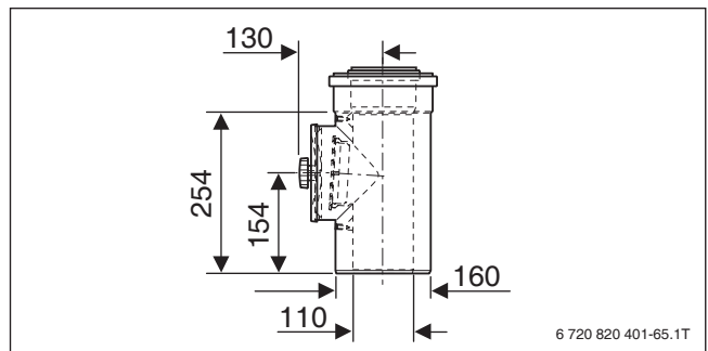
Bild 154 Konzentrisches Rohr mit Prüföffnung \varnothing 110/160 (Maße in mm)
