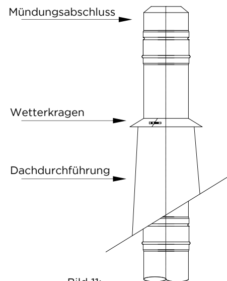
Bild 11: Dachdurchführung
