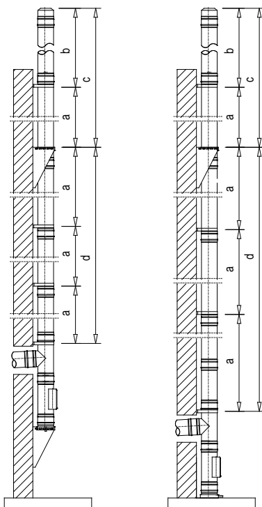
Bild 1: Aufbauhöhen
