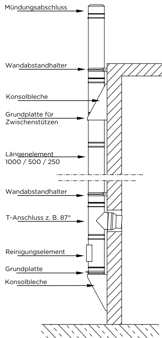
Bild 10: Aufbau mit Zwischenstütze
