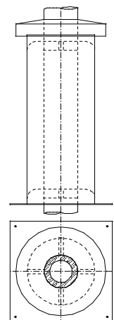
Bild 13: Aufbau Stulprohr mit integrierter Abluftführung
