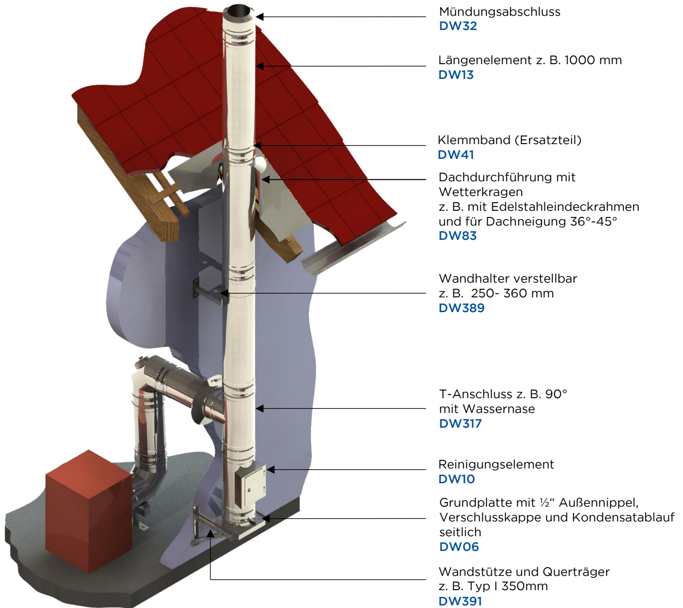
Bild 15: Ausführungsbeispiel
