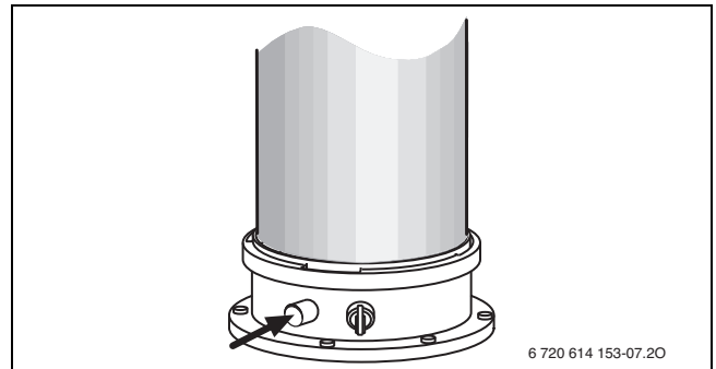
Bild 59 Abgasmessstutzen
