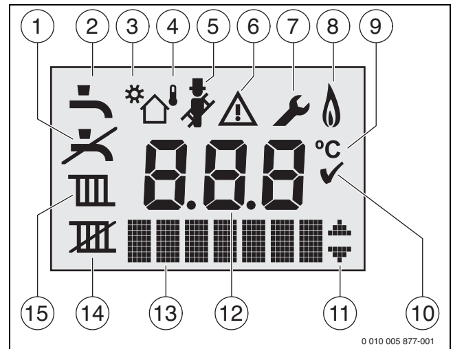
Bild 46 Displayanzeigen
