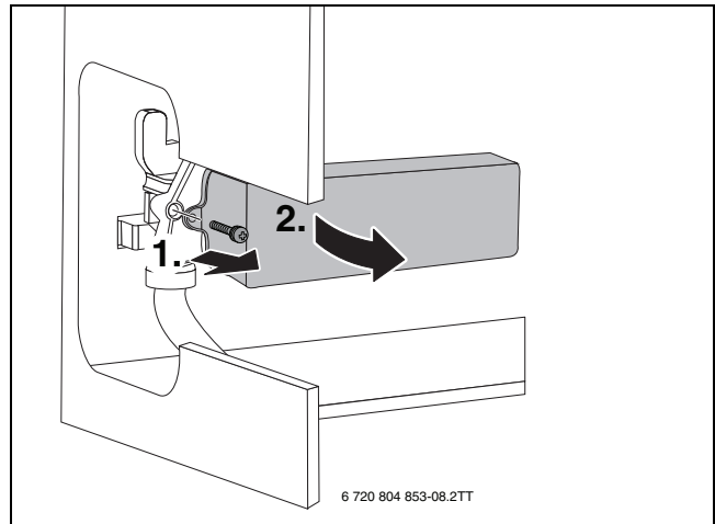
Bild 75 Plattenwärmetauscher ausbauen
