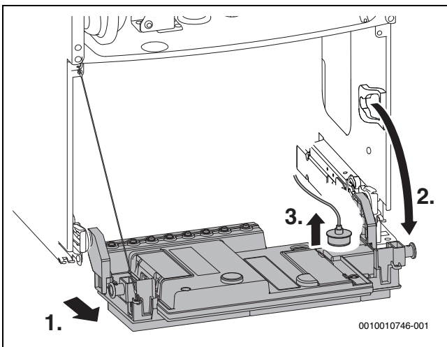
Bild 85 Steuergerät nach unten klappen
