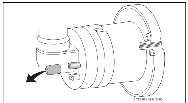
Bild 64 Messstutzen an der Mischeinrichtung
