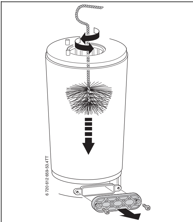
Bild 70 Wärmeblock reinigen
