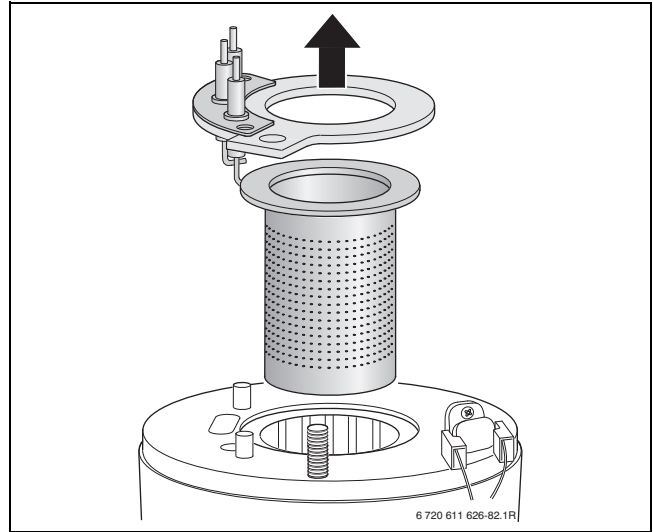
Bild 67 Brenner herausnehmen
