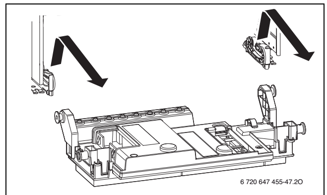
Bild 87 Steuergerät aushängen
