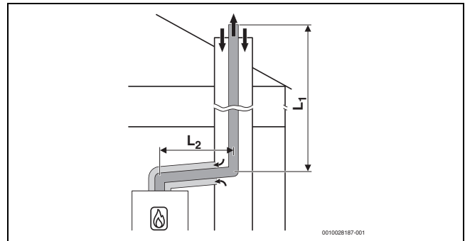
Bild 20 Starre Abgasführung nach C 93x im Schacht und konzentrische Luft-Abgas-Führung im Aufstellraum
