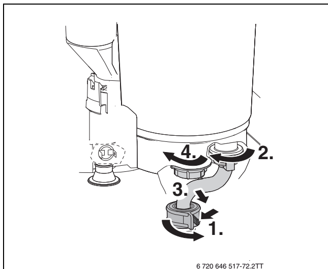
Bild 89 Mutter entfernen und Rücklaufrohr lösen
