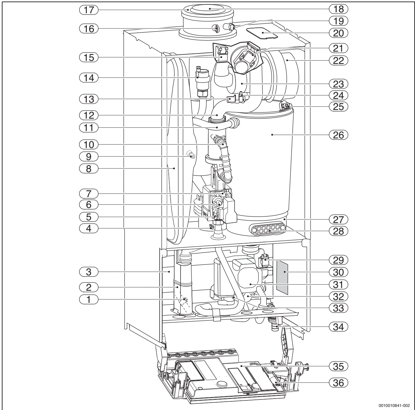
Bild 3 Produktübersicht GB182i... KD
