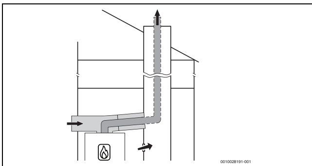
Bild 19 Luft-Abgas-Führung nach C 83(x) bis zum Schacht mit separater Luftzufuhr und konzentrischer Abgasableitung
