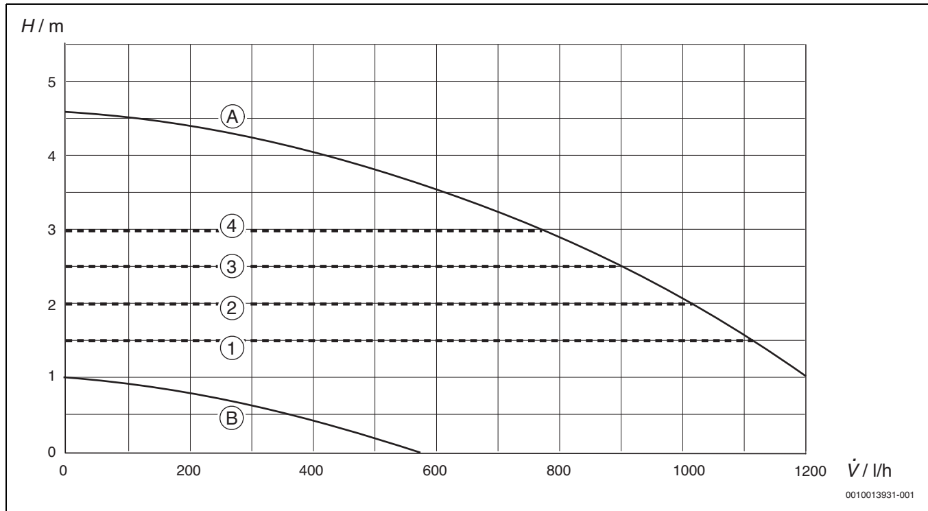
Bild 94 Pumpenkennfelder und Pumpenkennlinien
