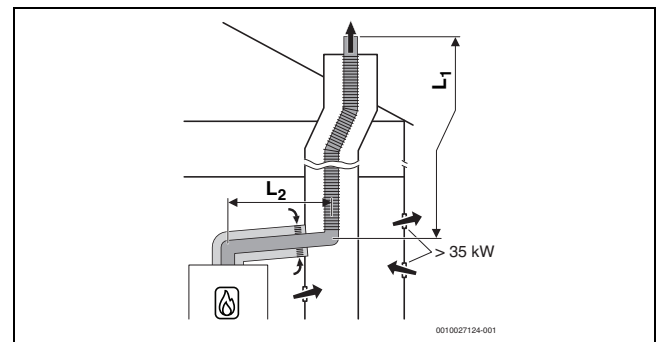
Bild 25 Flexible Abgasführung im Schacht nach B 33 mit raumluftabhängiger Luftzufuhr über die konzentrische Luft-Abgas-Führung im Aufstellraum
