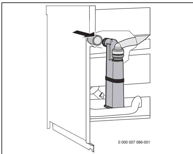
Bild 38 Schlauch am Kondensatsiphon montieren
