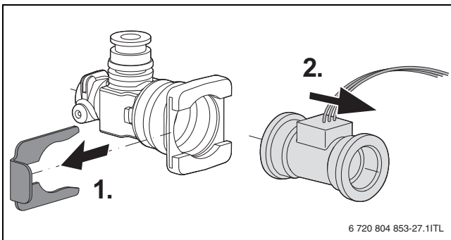
Bild 77 Turbine am Kaltwasserrohr ausbauen
