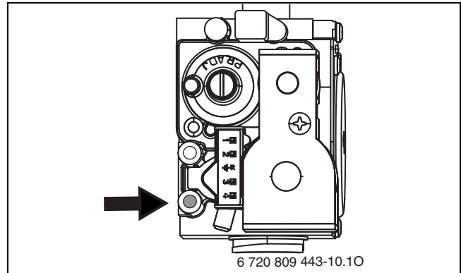
Bild 61 Messstutzen für Gas-Anschlussdruck
