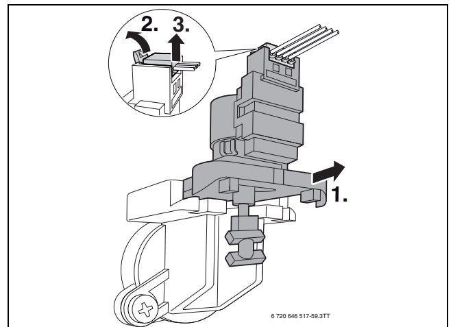
Bild 79 Motor des 3-Wege-Ventils ausbauen
