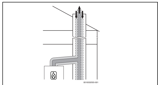
Bild 14 Konzentrische Luft-Abgas-Führung nach C (10)3x im Aufstellraum
