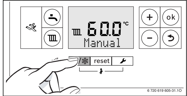
Bild 57 Manuellen Betrieb einstellen
