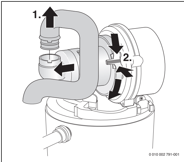
Bild 65 Saugrohr und Mischeinrichtung ausbauen
