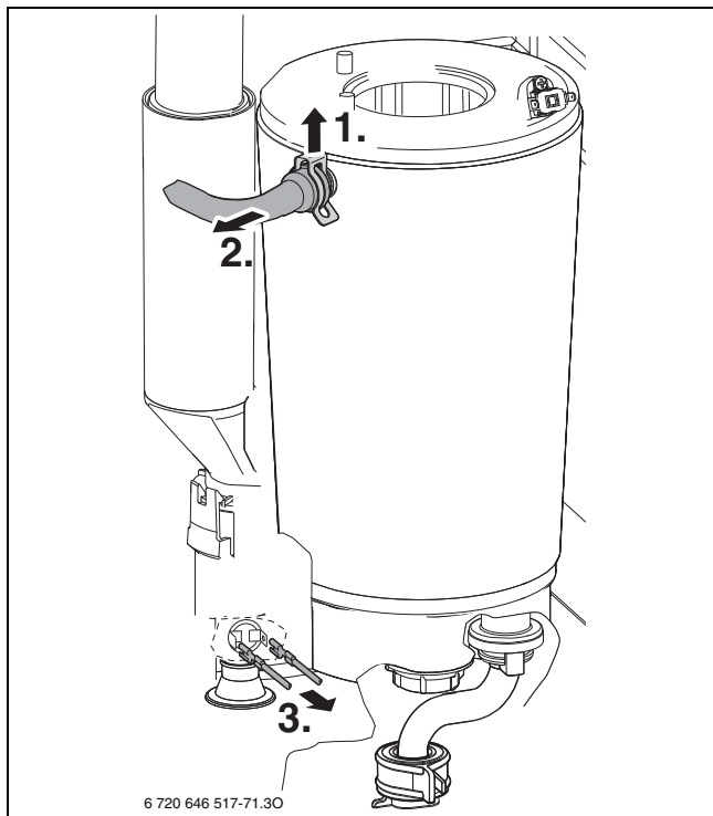
Bild 88 Vorlaufrohr lösen und Kabel abziehen
