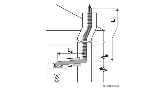
Bild 23 Flexible Abgasführung im Schacht nach B 23p /B 53p mit raumluftabhängiger Luftzufuhr am Gerät und konzentrischem Verbindungsstück zwischen Aufstellraum und Schacht
