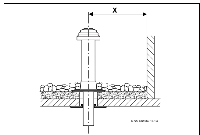
Bild 8 Abstandsmasse bei Flachdach
