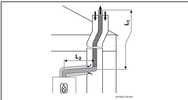
Bild 21 Flexible Abgasführung nach C 93x im Schacht und konzentrische Luft-Abgas-Führung im Aufstellraum
