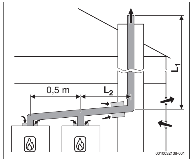
Bild 31 Kaskade mit 2 Geräten: Starre Abgasführung im Schacht nach B 23p /B 53p mit raumluftabhängiger Luftzufuhr am Gerät
