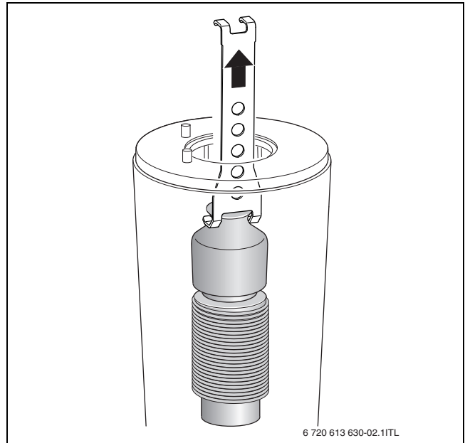
Bild 68 Oberen Verdrängungskörper herausnehmen
