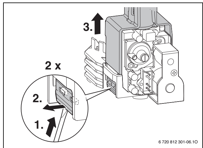
Bild 83 Gasarmatur ausbauen
