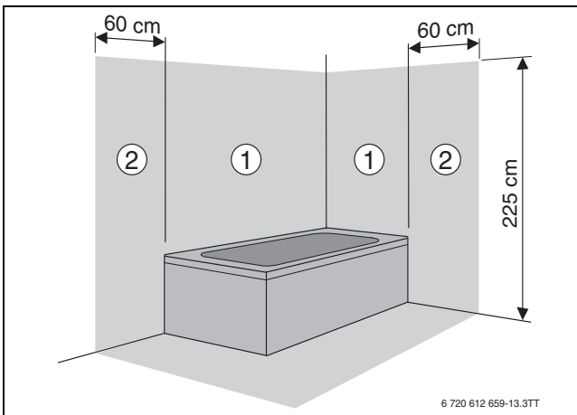
Bild 41 Schutzbereiche
