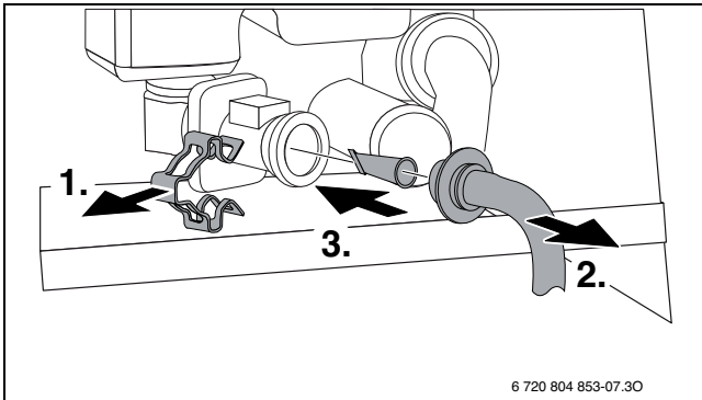
Bild 76 Sieb aus Kaltwasserrohr ausbauen
