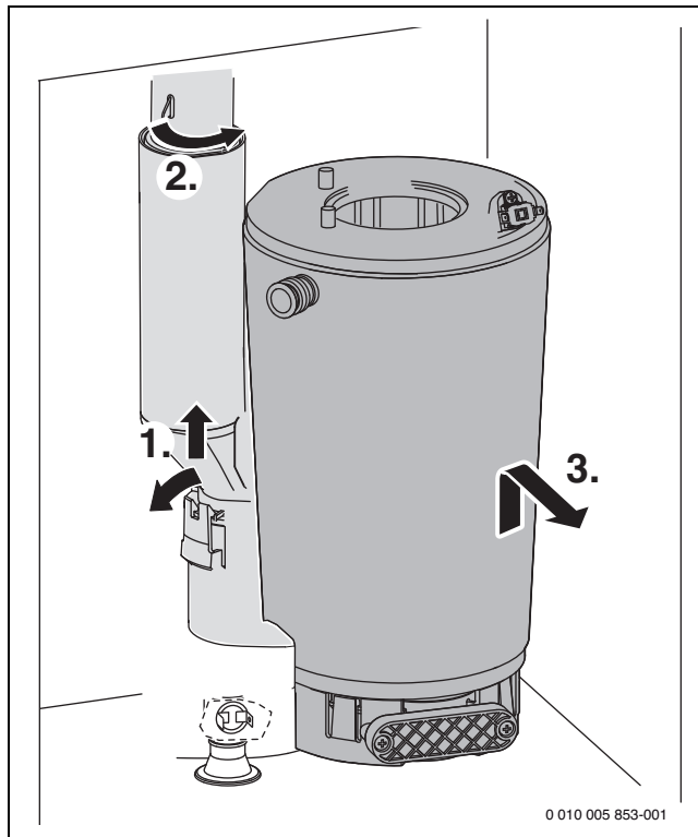
Bild 90 Wärmeblock ausbauen
