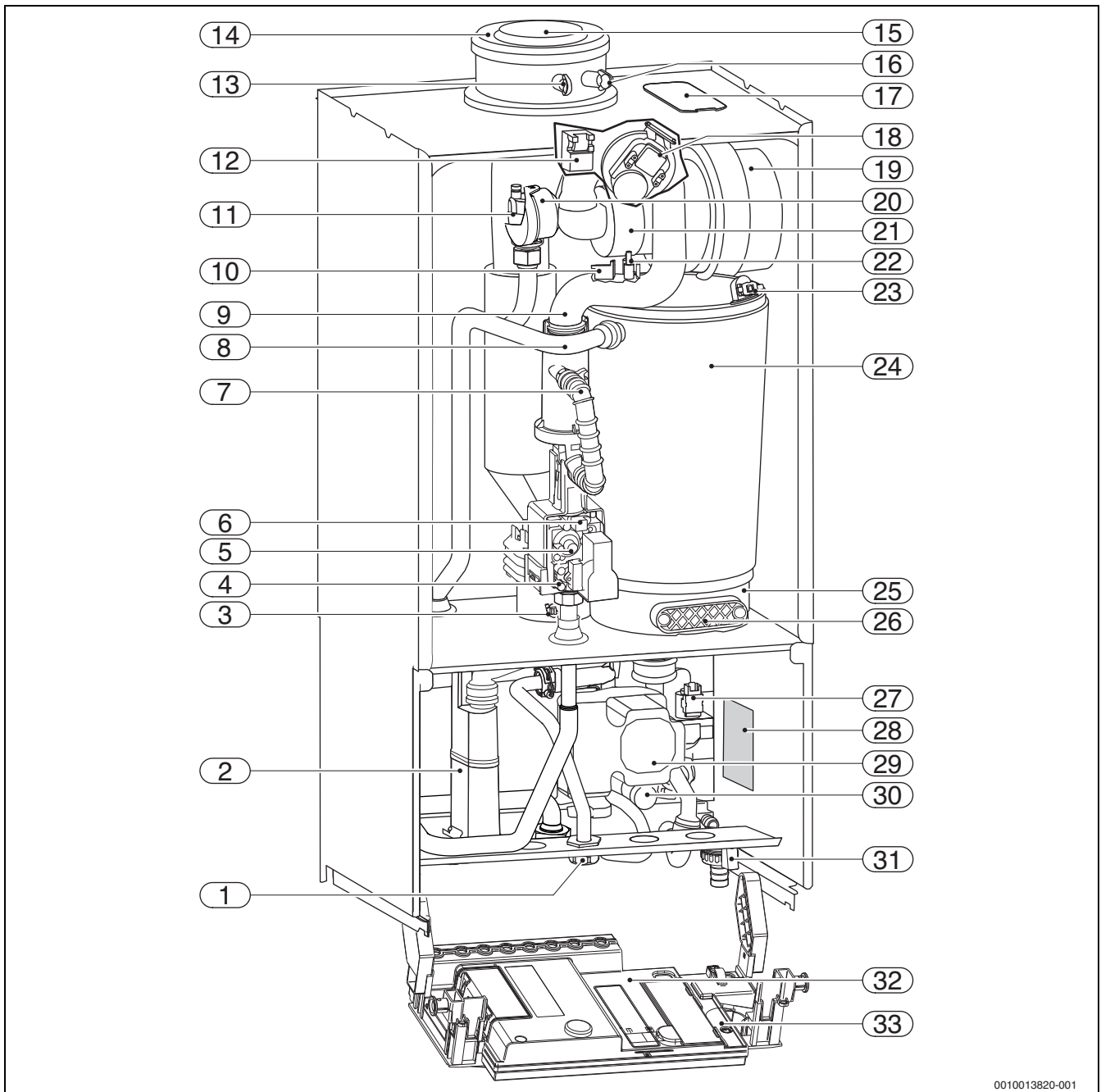
Bild 4 Produktübersicht GB182i-..
