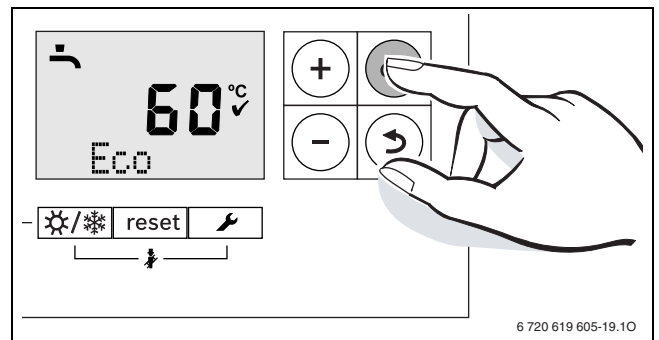
Bild 54 Anzeige Warmwassertemperatur bestätigen
