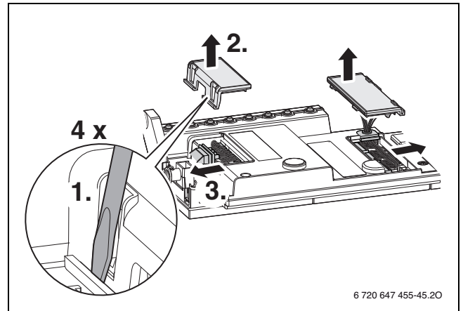
Bild 86 Abdeckung entfernen
