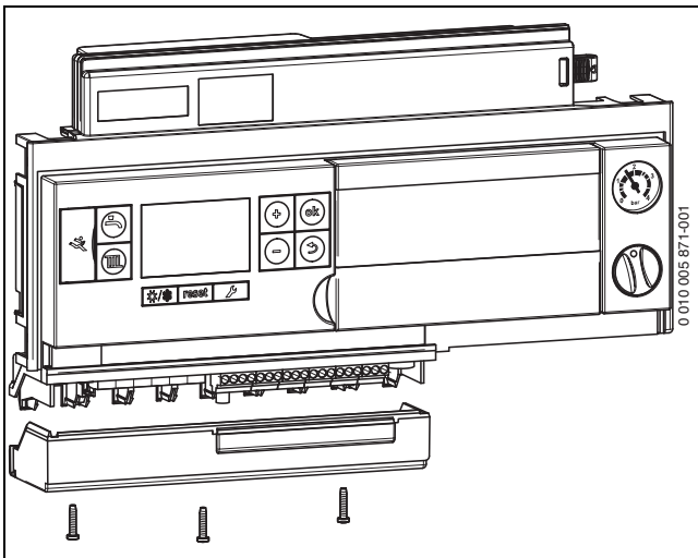
Bild 84 Abdeckung entfernen
