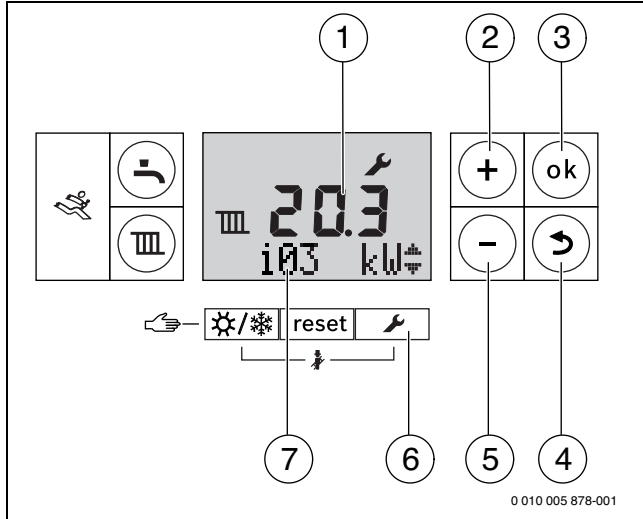
Bild 58 Übersicht der Bedienelemente
