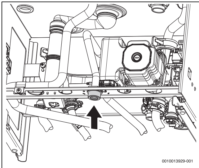
Bild 34 Anschluss externes Ausdehnungsgefäß
