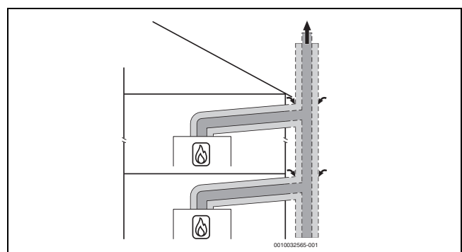
Bild 27 Mehrfachbelegung nach C (12)3x mit konzentrischer Luft-Abgas-Führung im Aufstellraum
