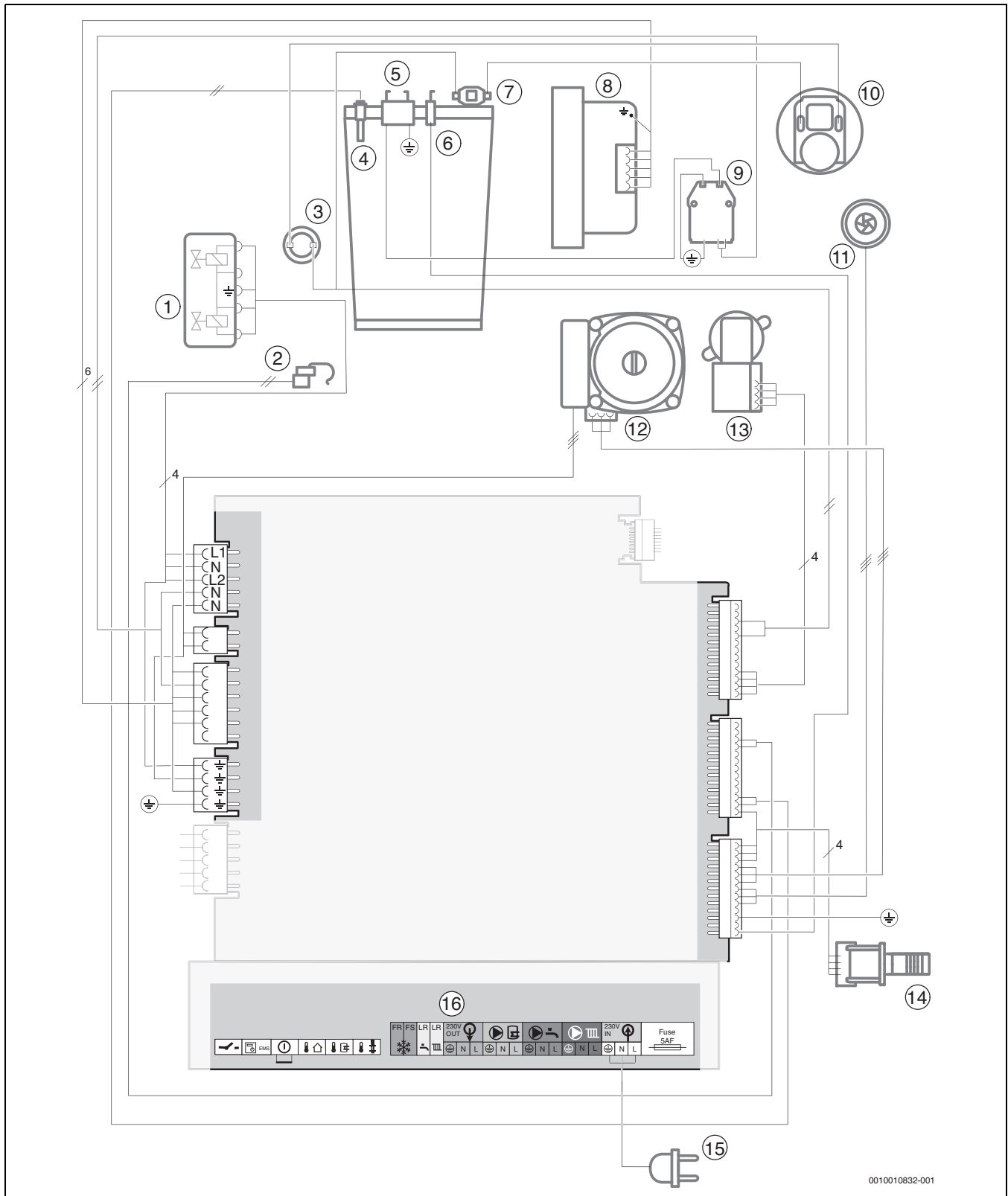
Bild 93 Elektrische Verdrahtung
