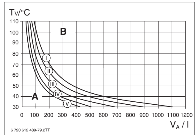
Bild 35 Kennlinien des Ausdehnungsgefäßes
