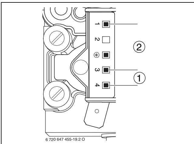
Bild 81 Messstellen an der Gasarmatur
