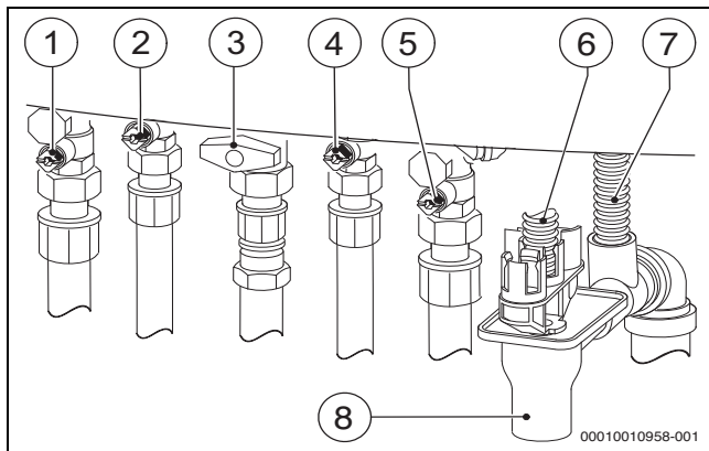
Bild 40 Gas- und wasserseitige Anschlüsse (Zubehör)
