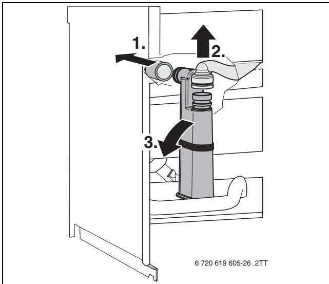
Bild 73 Kondensatsiphon ausbauen
