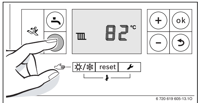
Bild 49 Anzeige Vorlauftemperatur
