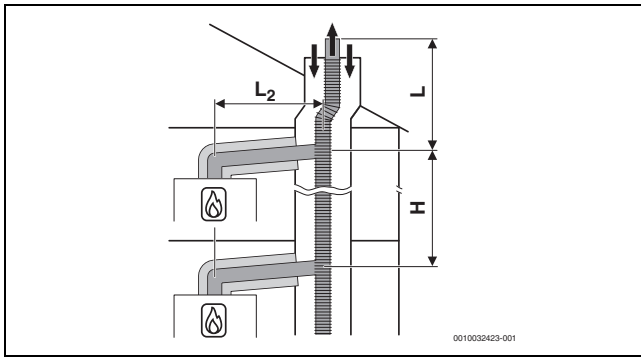
Bild 30 Mehrfachbelegung nach C_{(14)3x} mit kollektiver flexibler Abgasableitung und konzentrischer Luft-Abgas-Führung im Aufstellraum
