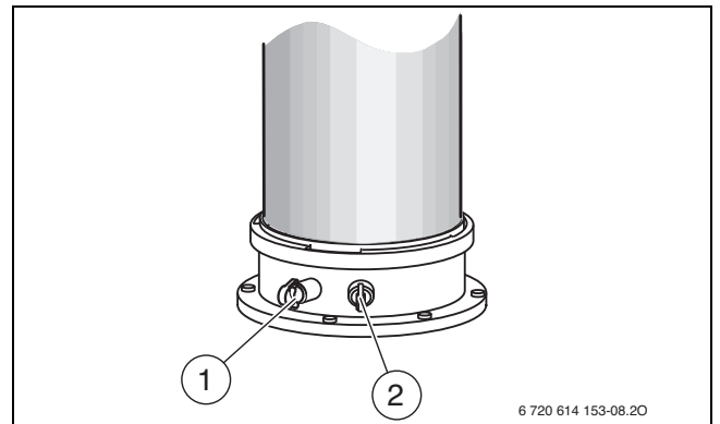
Bild 63 Abgassmessstutzen und Verbrennungsluft-Messstutzen
