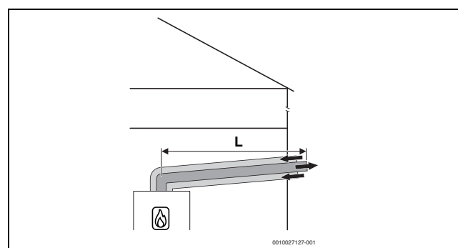
Bild 11 Horizontale konzentrische Luft-Abgas-Führung nach C 13x durch die Außenwand
