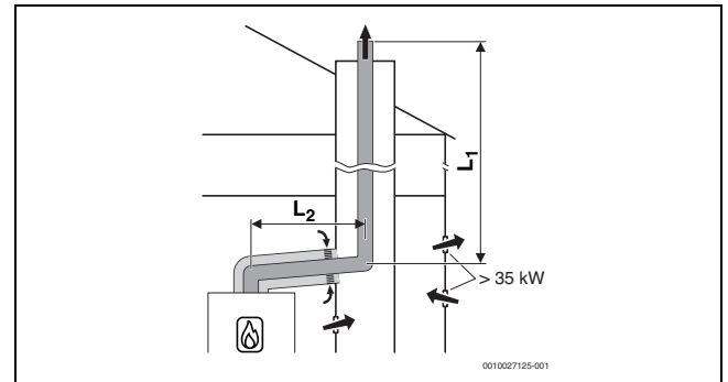
Bild 24 Starre Abgasführung im Schacht nach B 33 mit raumluftabhängiger Luftzufuhr über die konzentrische Luft-Abgas-Führung im Aufstellraum
