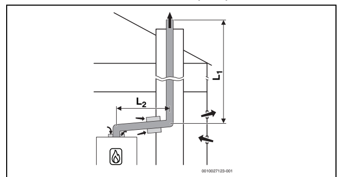
Bild 22 Starre Abgasführung im Schacht nach B 23p /B 53p mit raumluftabhängiger Luftzufuhr am Gerät und konzentrischem Verbindungsstück zwischen Aufstellraum und Schacht
