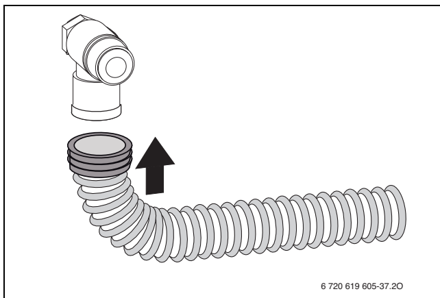
Bild 37 Schlauch am Sicherheitsventil montieren
