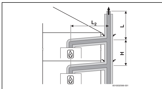
Bild 28 Mehrfachbelegung nach C (13)3x mit konzentrischer Luft-Abgas-Führung an der Außenwand und im Aufstellraum
