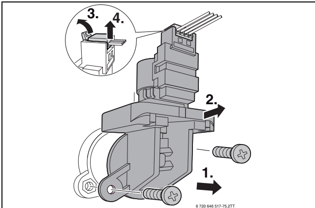
Bild 80 3-Wege-Ventil ausbauen
