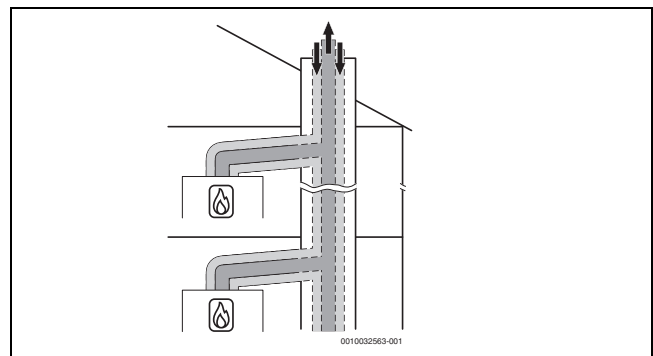
Bild 26 Mehrfachbelegung nach C (10)3x mit konzentrischer Luft-Abgas-Führung im Aufstellraum
