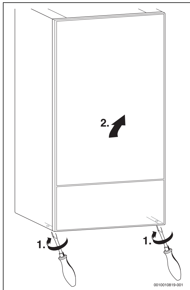
Bild 36 Verkleidung abnehmen
