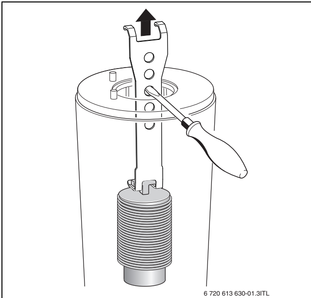
Bild 69 Unteren Verdrängungskörper herausnehmen
