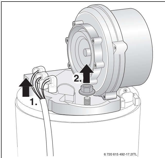
Bild 66 Gebläse herausnehmen
