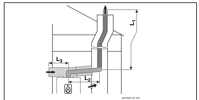
Bild 17 Flexible Abgasführung nach C 53(x) im Schacht und Luft-Abgas-Führung mit separater Luftzufuhr und konzentrischer Abgasableitung im Aufstellraum
