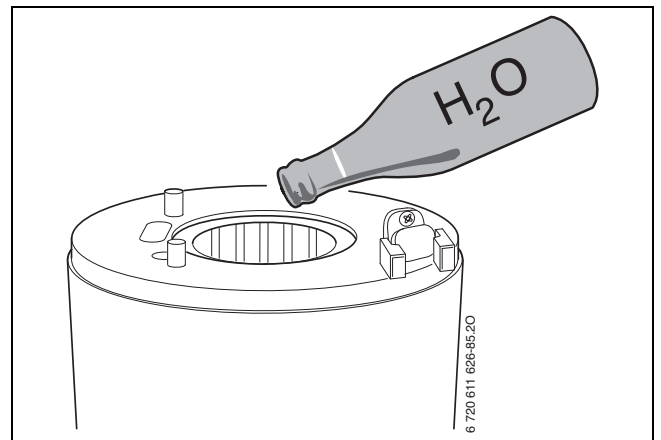
Bild 72 Wärmeblock mit Wasser spülen
