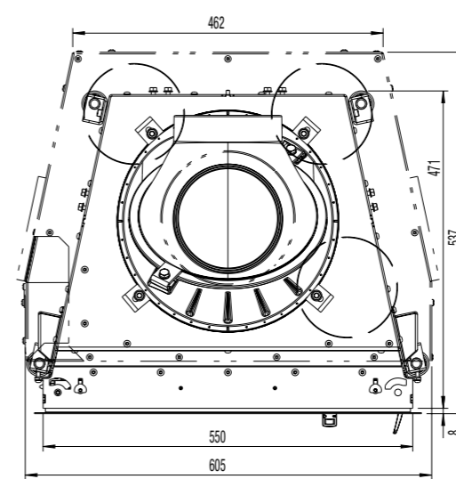
Maßstab 1:10
