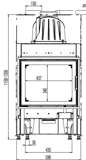
Maßstab 1:20
