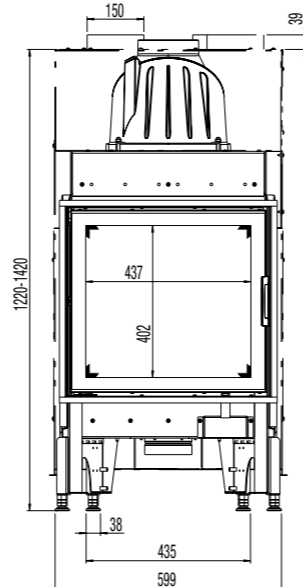
Maßstab 1:20
