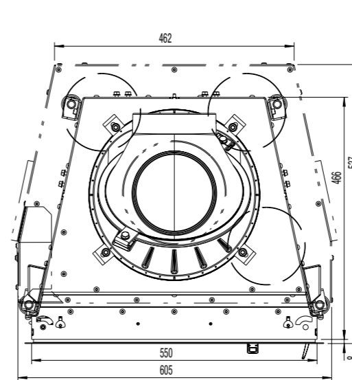
Maßstab 1:10
