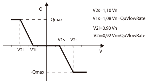
Blindleistungssteuerung, Blindleistung Standardkennlinie Q= f(V)
