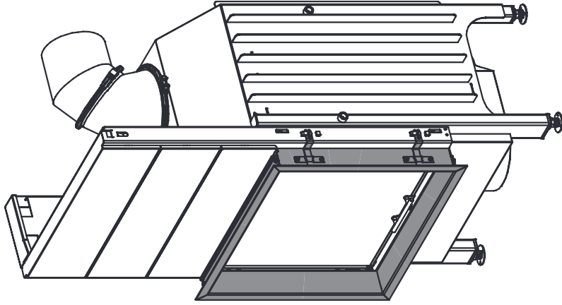
Steckblende (nur 1V-Brennzellen)
