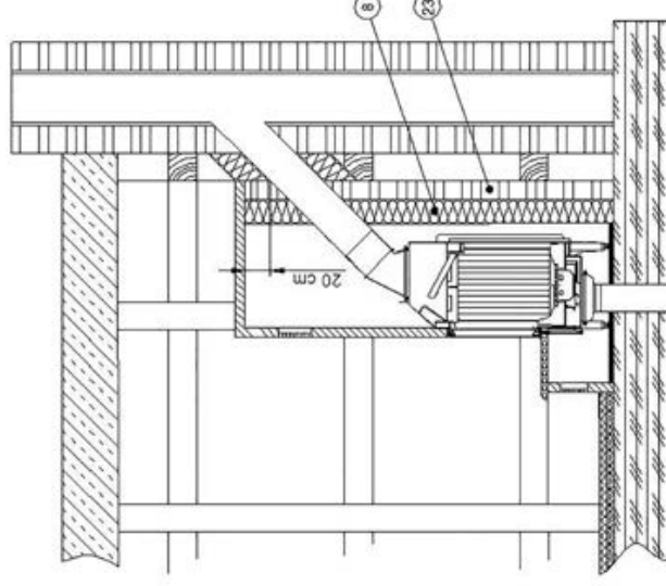
8. Dämmung der Heizkammer gemäß den Wärmedämmstoffdicken der technischen Daten 23 Vormauerung, 10 cm stark*
