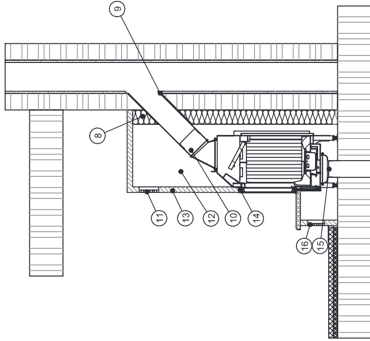
Die Abbildung zeigt eine beispielhafte Aufbausituation eines Varia 1V-51-4S und gilt exemplarisch für jede Brennzelle.
