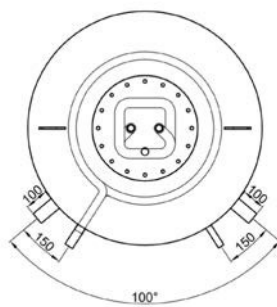
Hygiene-Kombispeicher Typ KER (mit einem Wärmetauscher)
