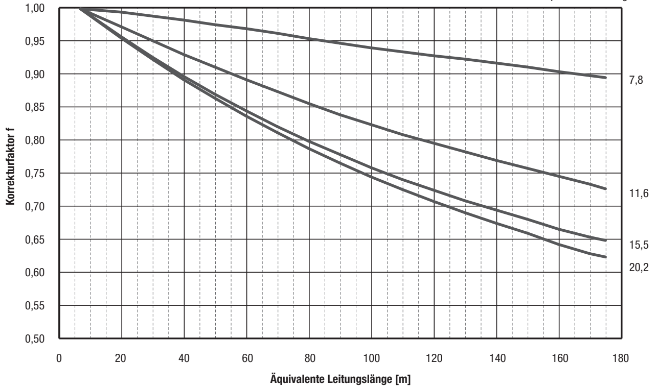
PUMY-P112VKM, PUMY-P112YKM: Heizbetrieb PUMY-P125VKM, PUMY-P125YKM: Heizbetrieb PUMY-P140VKM, PUMY-P140YKM: Heizbetrieb
