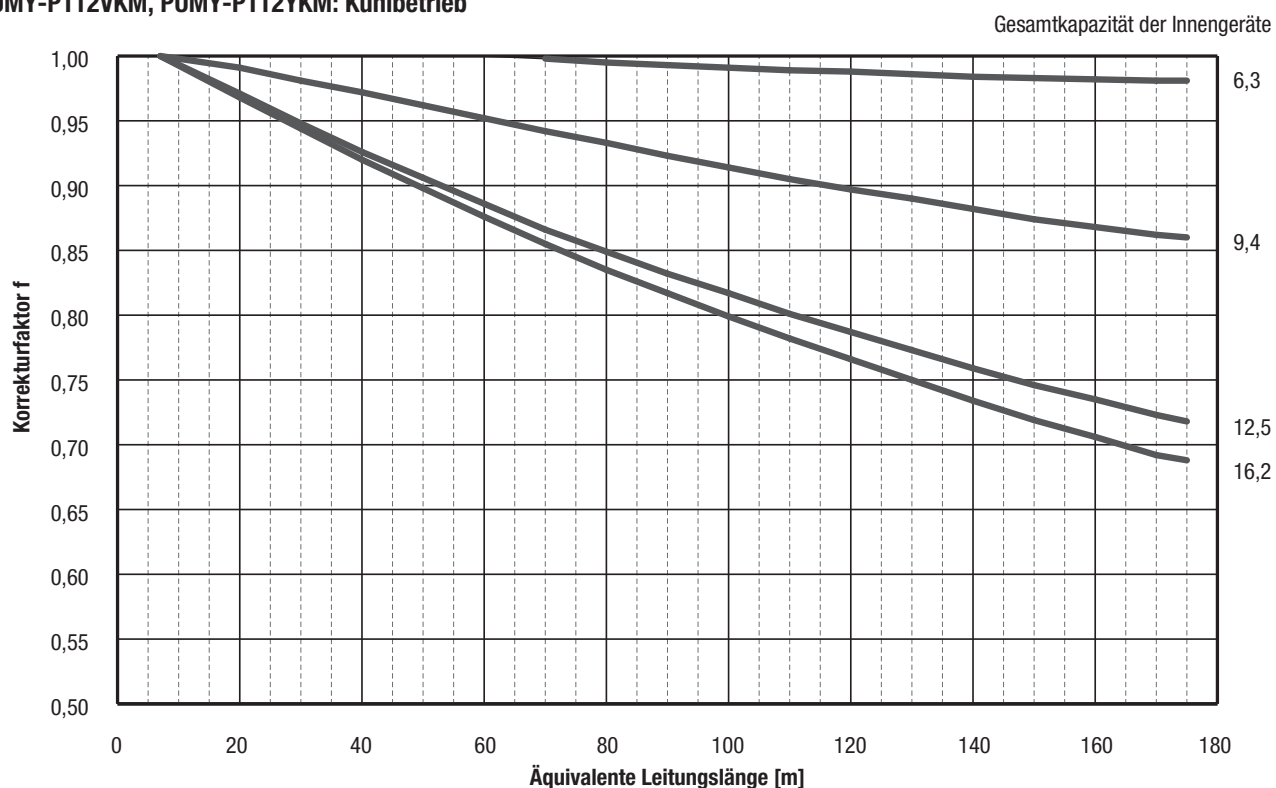
PUMY-P112VKM, PUMY-P112YKM: Kühlbetrieb
