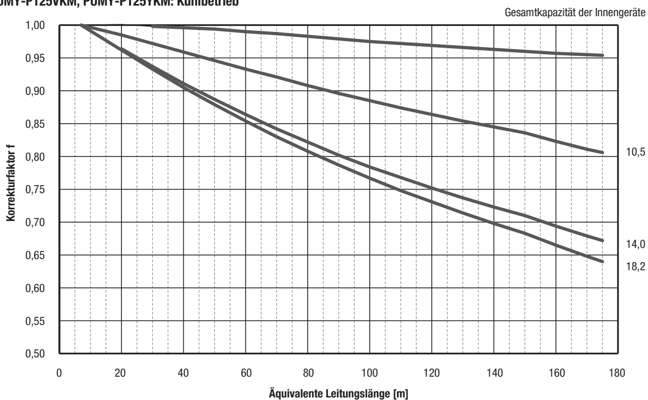
PUMY-P125VKM, PUMY-P125YKM: Kühlbetrieb
