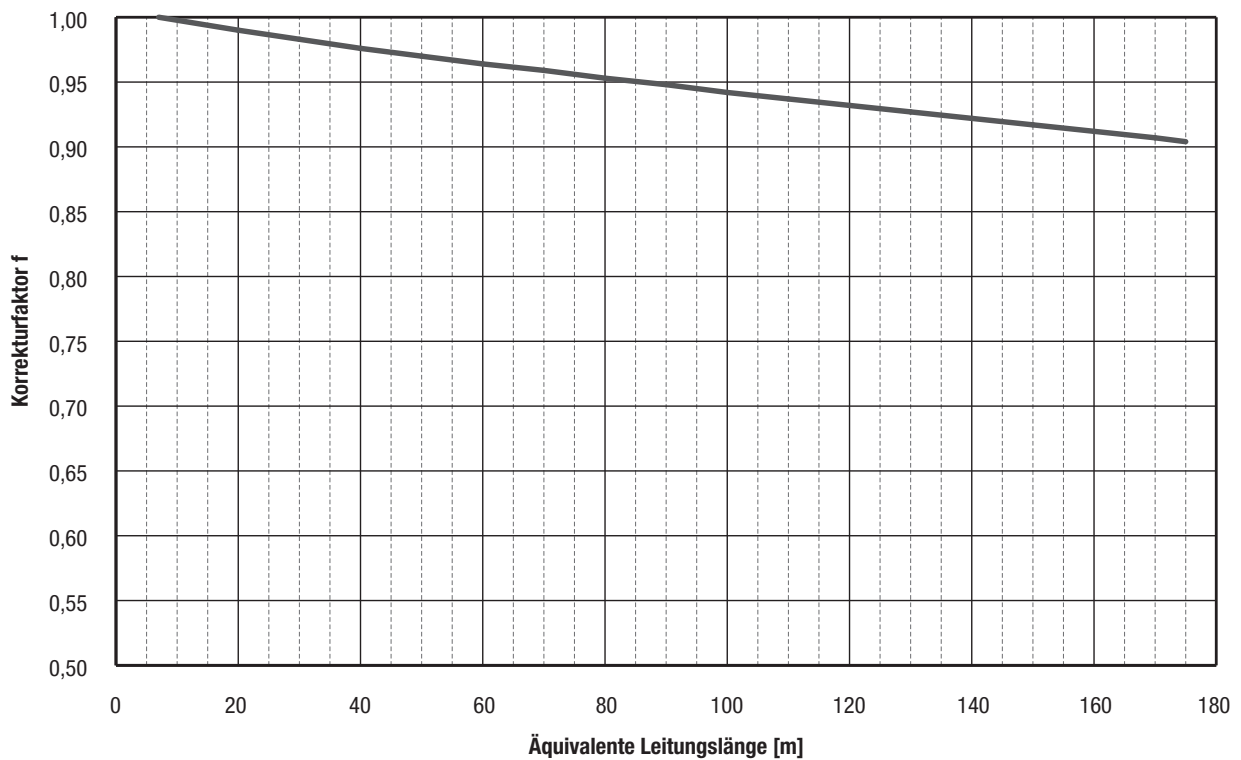
PUMY-P112VKM, PUMY-P112YKM: Heizbetrieb PUMY-P125VKM, PUMY-P125YKM: Heizbetrieb PUMY-P140VKM, PUMY-P140YKM: Heizbetrieb
