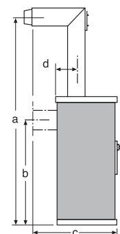
Maß a und c: mit Original-Winkelrohr dimension a and c: with original angle pipe Cotes a et c : avec conduit coude d'origine Wymiary a i c : z oryginalną rurą pod kątem 90°
