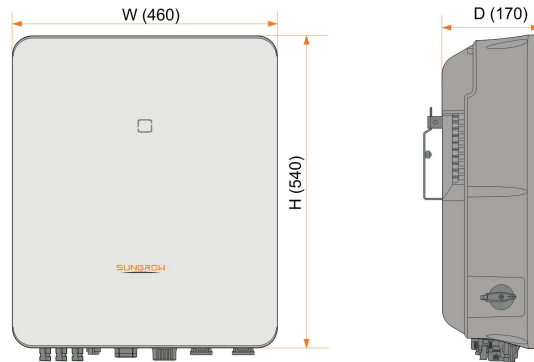
Abbildung 2-2 Abmessungen des Wechselrichters (in mm)
