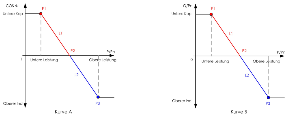
Abbildung 8-2 Q(P)-Kurve
