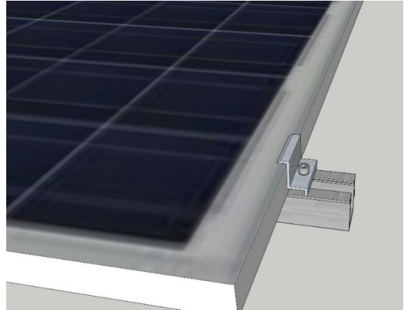
Abbildung 12/Modulendklemme anbringen
