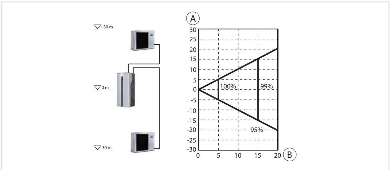
Abb. 46: Heizleistungsverluste bei WKF/WKF-compact 100
