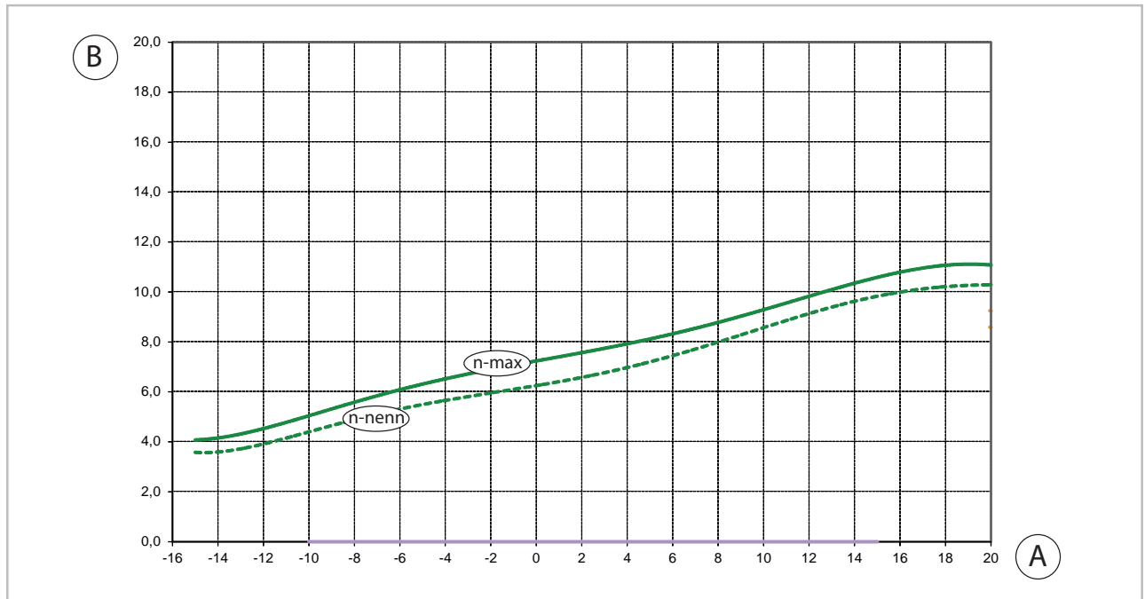
Abb. 26: Heizleistung WKF/WKF-compact 100 bei Vorlauftemperatur 55 °C
