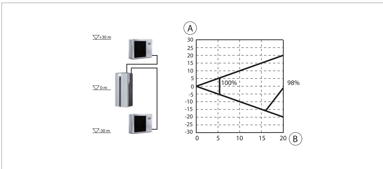
Abb. 49: Kühlleistungsverluste bei WKF/WKF-compact 130/WKF 130 Duo
