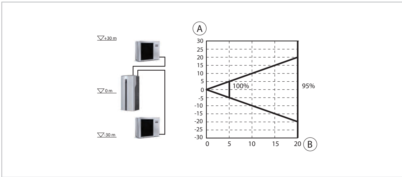
Abb. 48: Heizleistungsverluste bei WKF/WKF-compact 130/WKF 130 Duo
