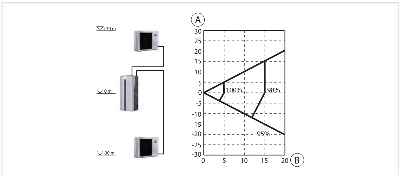
Abb. 47: Kühlleistungsverluste bei WKF/WKF-compact 100
