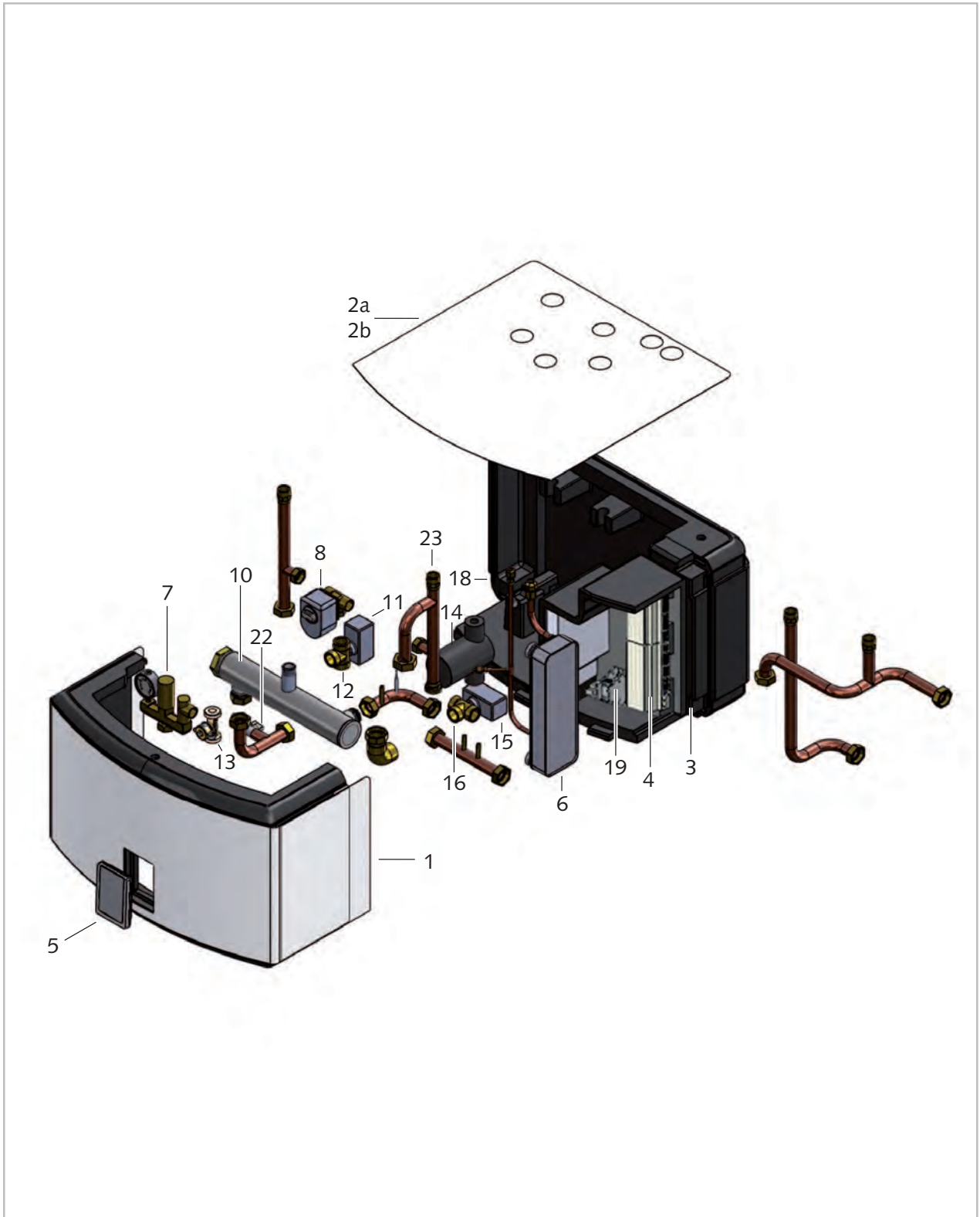
Abb. 84: Explosionszeichnung
