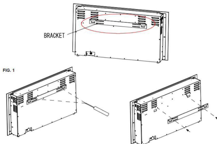
AV-WM42-50-60-65-72-100ROY Muurbeugel geïllustreerd
