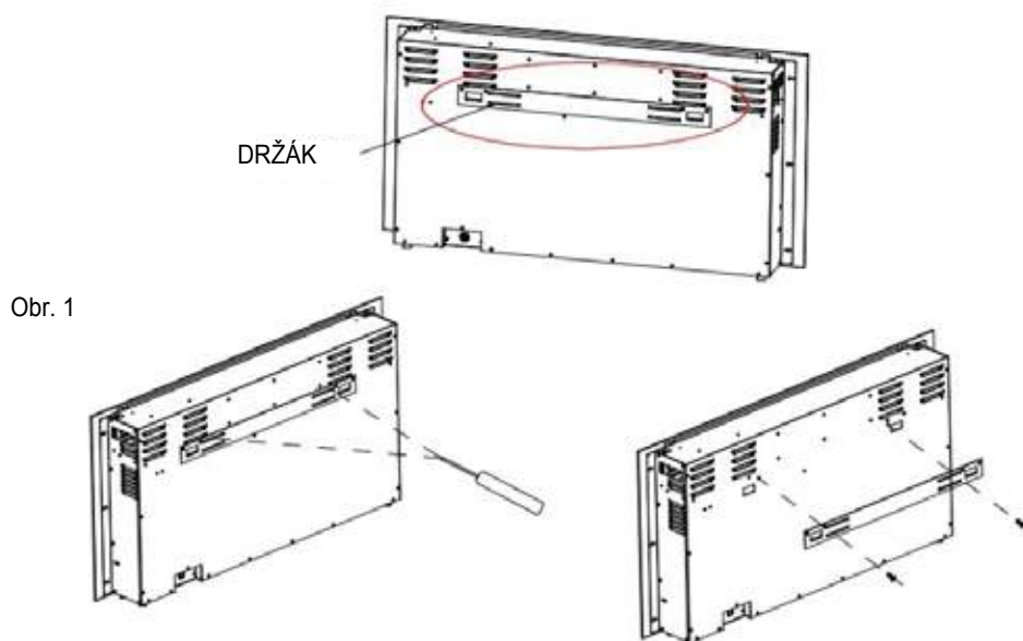
Ilustrace představující nástěnnou vzpěru pro modely AV-WM42-50-60-65-72-100ROY
