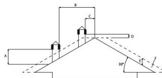
30° TOIT
