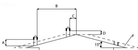
TELHADO A 15°
