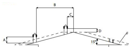
15° TOIT
