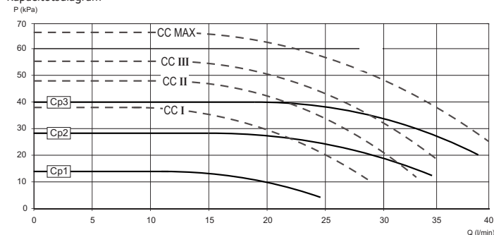
Kapazitätsdiagramm
