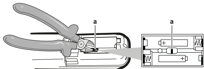
a Adressierungs-Jumper
