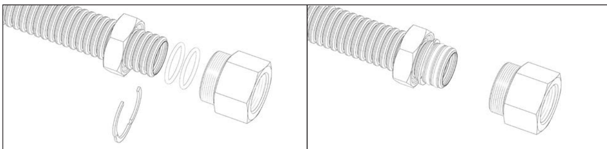
Abb. 6.5.2 Rohranschluss C-Clip
