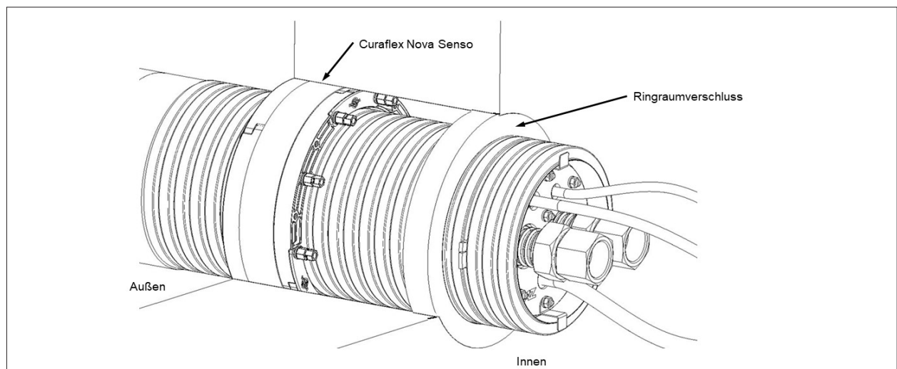
Abb. 6.3.2 Ringraumverschlüsse Typ Kellerdurchführung
