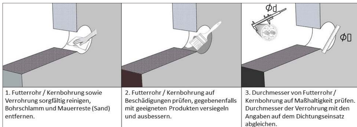
Abb. 4.3 Wanddurchdringung
