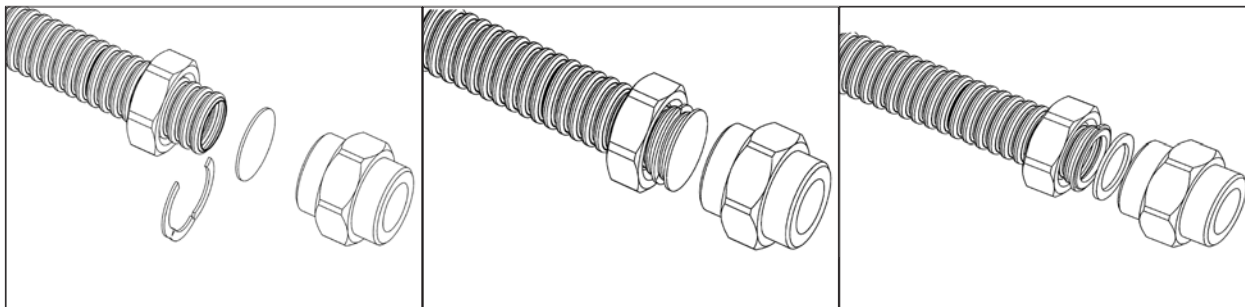
Abb. 6.5.1 Stauchanschluss
