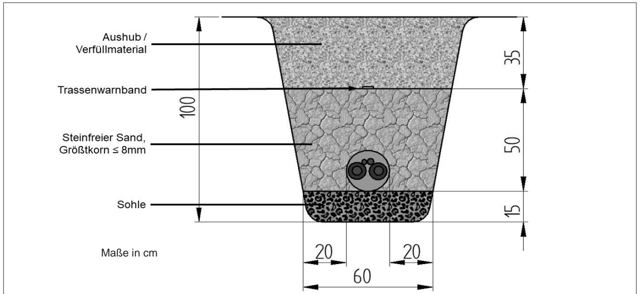
Abb. 4.4 Einbettung des Mantelrohres
