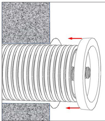
Abb. 6.3.1 Ringraumverschluss bei Typ Wanddurchführung
