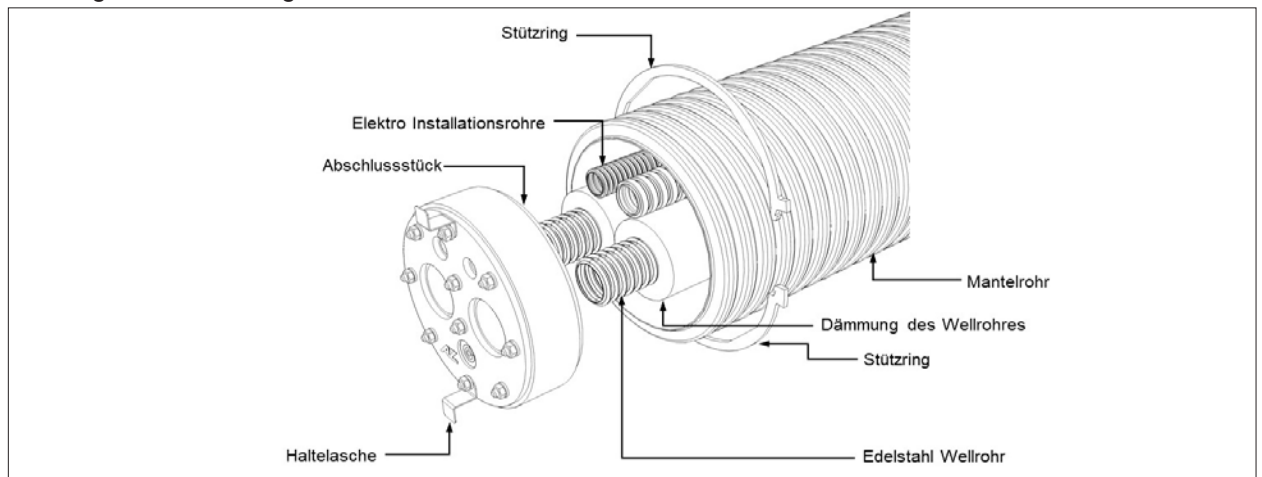
Abb. 6.4-1 Abschlussstück Mantelrohr
