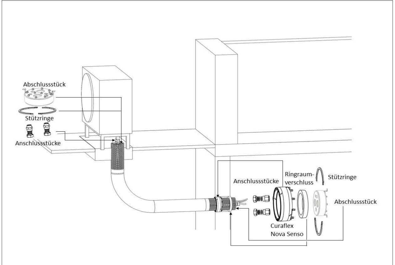
Abb. 3.2 Kellereinführung
