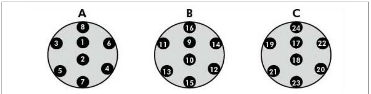
Abb. 6.4-3 Verspannen des Abschlussstückes
