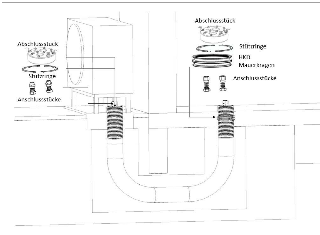
Abb. 3.3 Typ Bodenplatteneinführung
