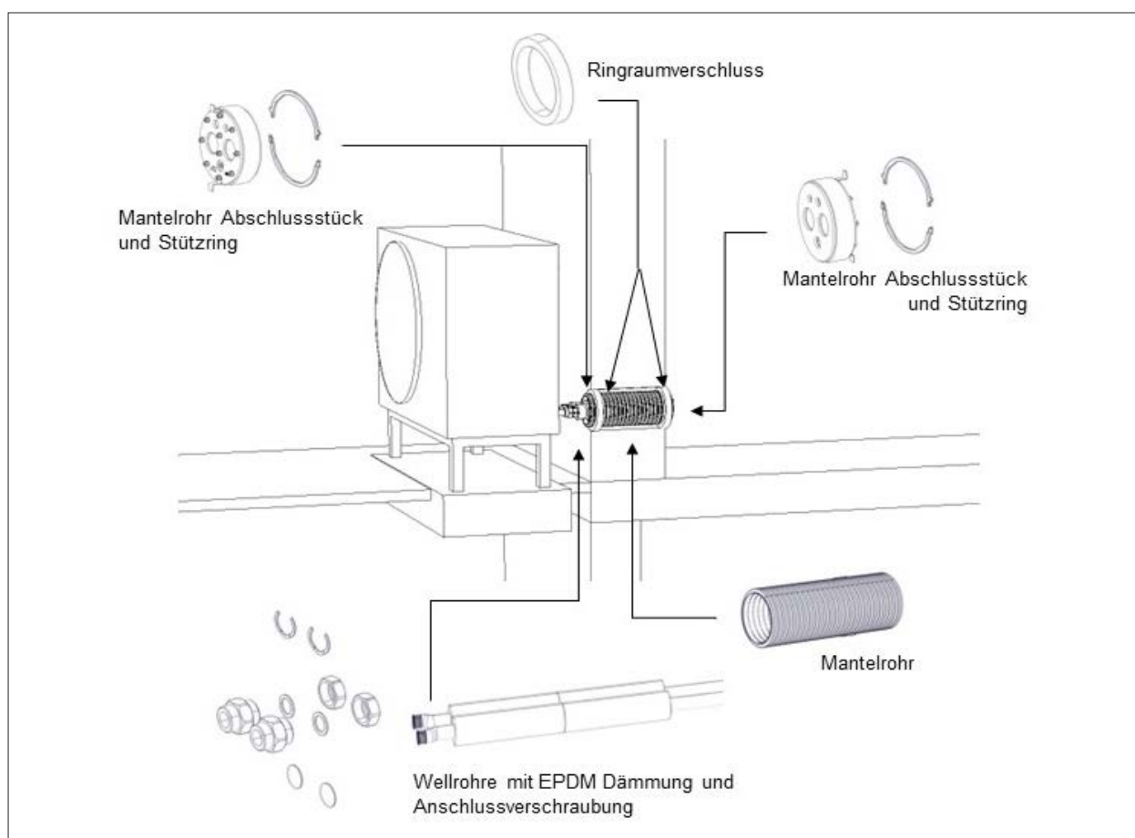
Abb. 3.1 Typ Wanddurchführung
