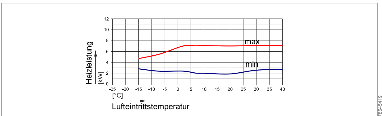
Abb. 10: Heizleistung CHA-07 bei einem Vorlauf von 65 °C
