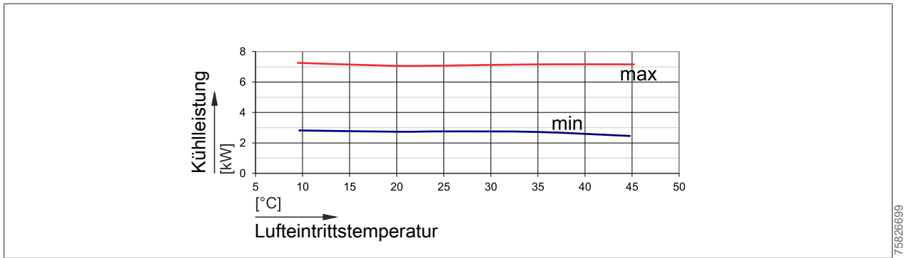
Abb. 16: Kühlleistung CHA-07 bei einem Vorlauf von 18 °C
