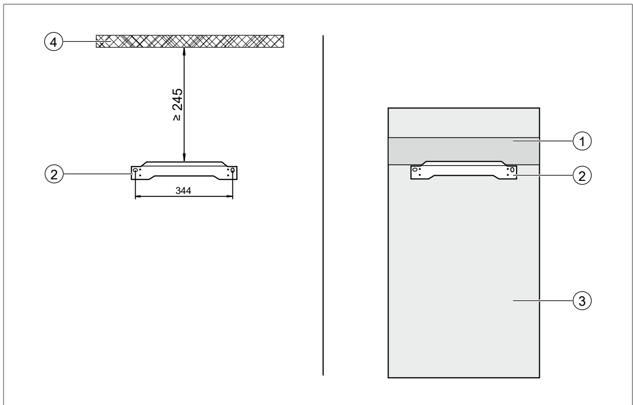
Abb. 5: Gerätebefestigung mit Einhängewinkel
