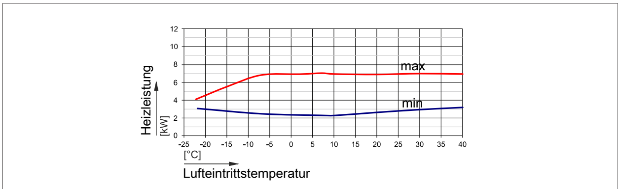
Abb. 7: Heizleistung CHA-07 bei einem Vorlauf von 35 °C
