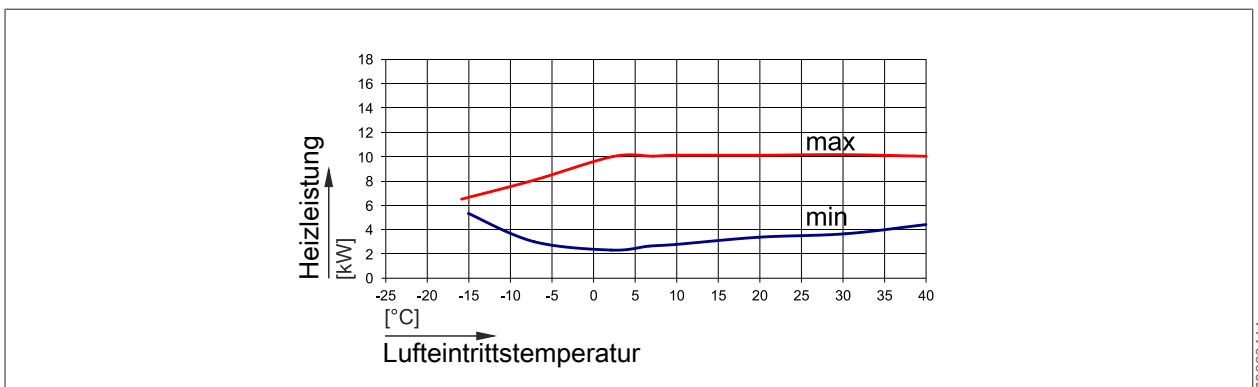
Abb. 15: Heizleistung CHA-10 bei einem Vorlauf von 65 °C
