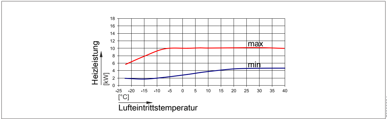
Abb. 12: Heizleistung CHA-10 bei einem Vorlauf von 35 °C
