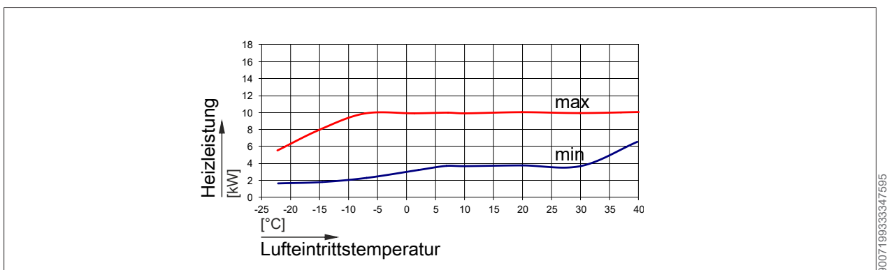
Abb. 11: Heizleistung CHA-10 bei einem Vorlauf von 25 °C
