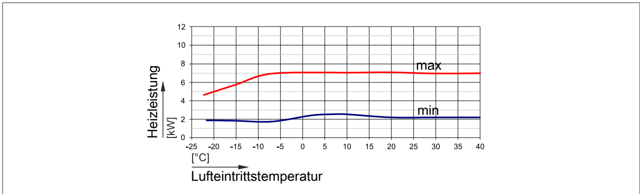
Abb. 6: Heizleistung CHA-07 bei einem Vorlauf von 25 °C
