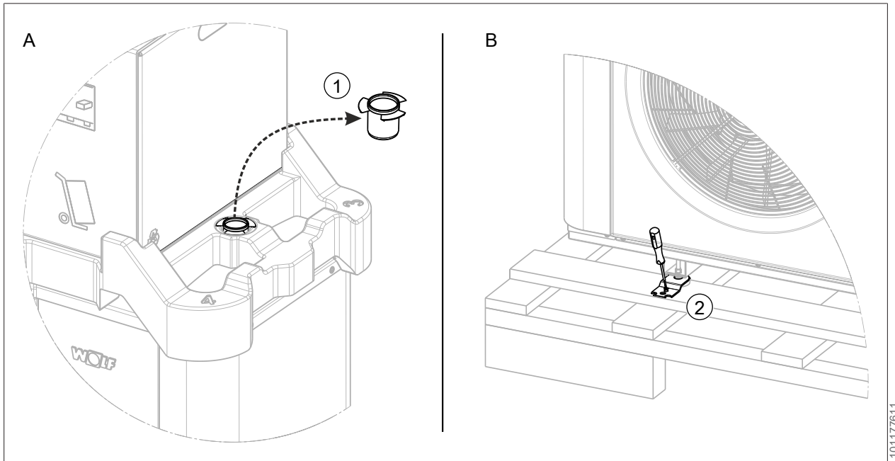
1 Kondensatstutzen
