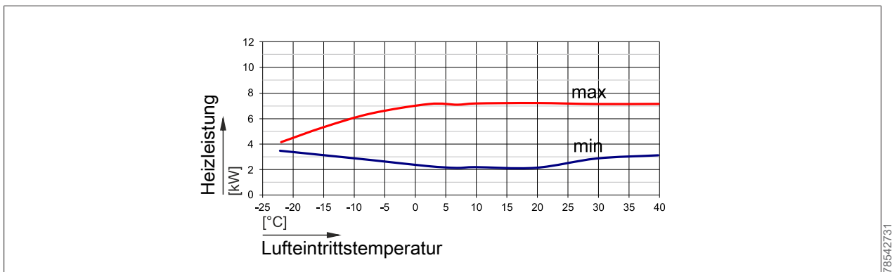
Abb. 9: Heizleistung CHA-07 bei einem Vorlauf von 55 °C
