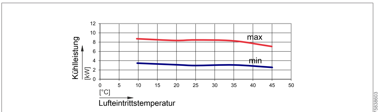
Abb. 19: Kühlleistung CHA-10 bei einem Vorlauf von 7 °C
