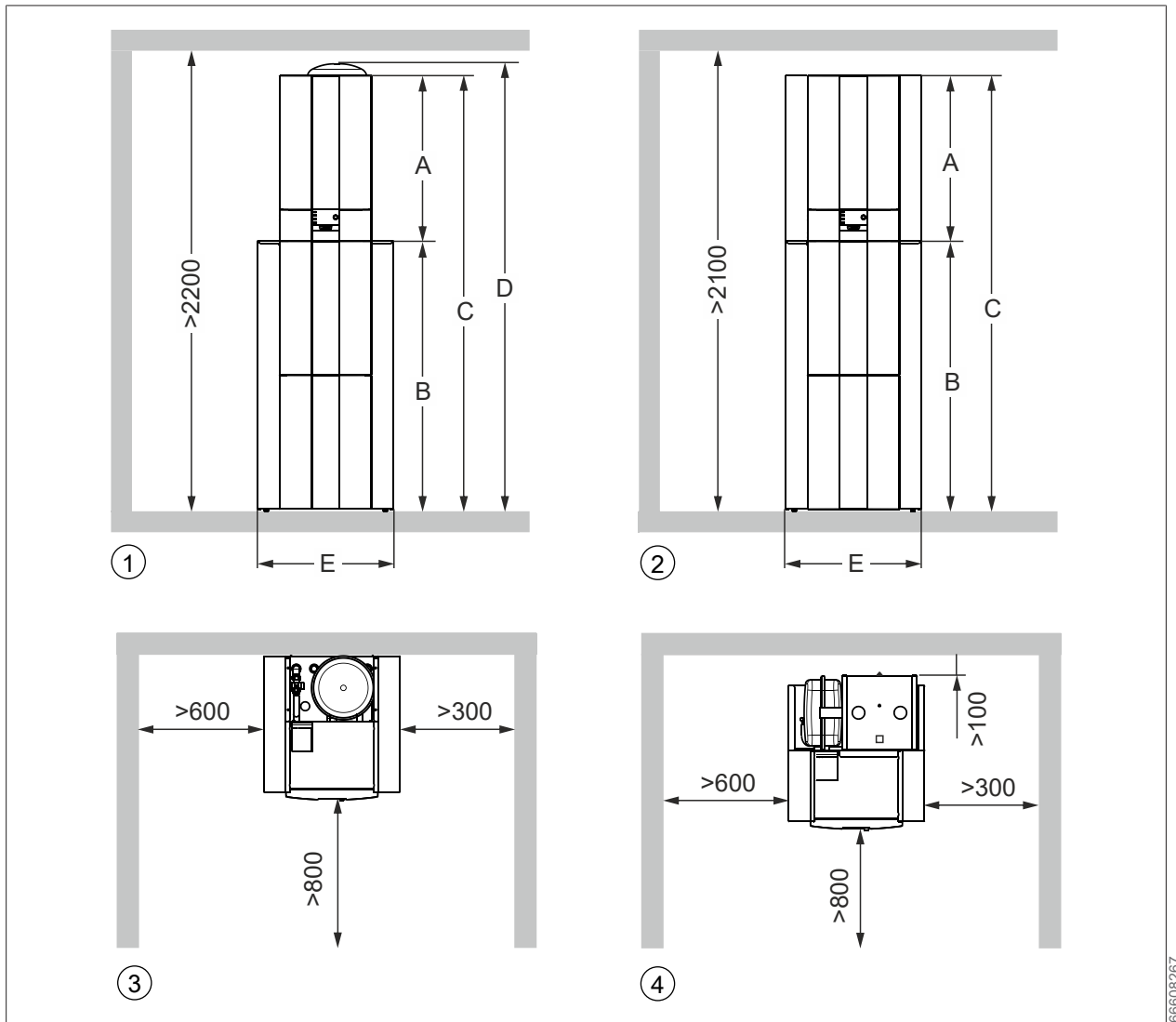
1 Vorderansicht CHC-Monoblock / 200
