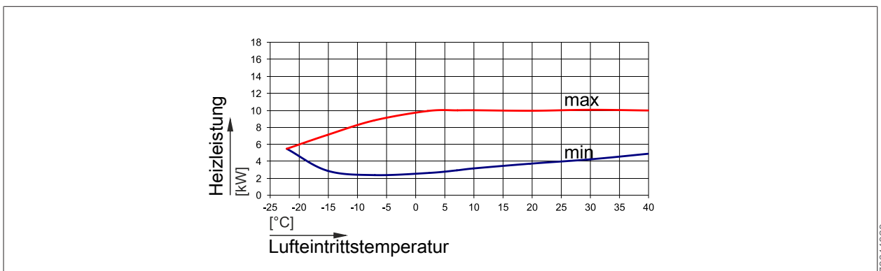
Abb. 14: Heizleistung CHA-10 bei einem Vorlauf von 55 °C
