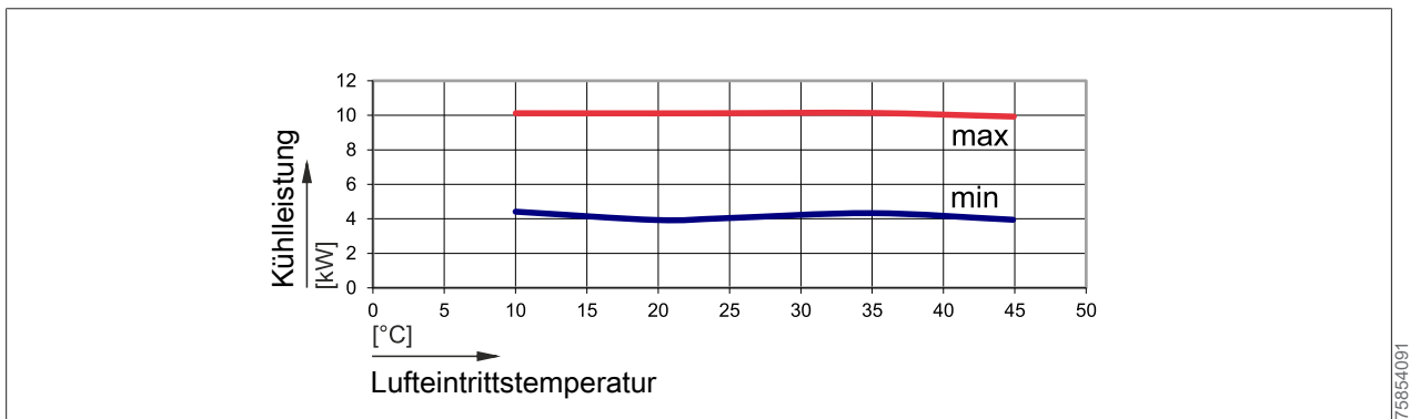
Abb. 18: Kühlleistung CHA-10 bei einem Vorlauf von 18 °C
