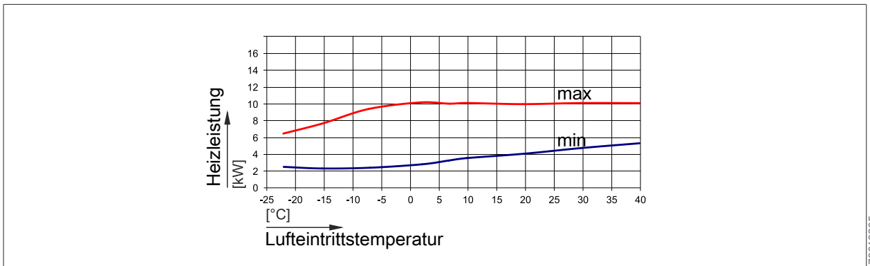
Abb. 13: Heizleistung CHA-10 bei einem Vorlauf von 45 °C
