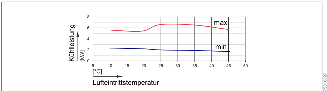
Abb. 17: Kühlleistung CHA-07 bei einem Vorlauf von 7 °C
