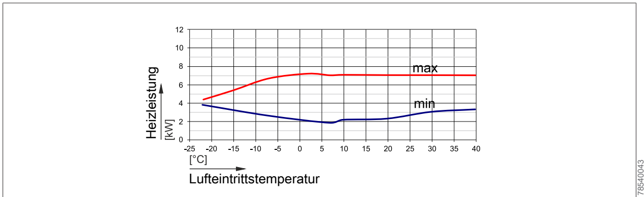
Abb. 8: Heizleistung CHA-07 bei einem Vorlauf von 45 °C
