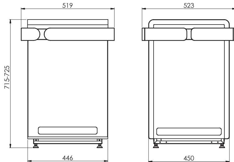
Abb.5 Abmessungen Concept R 9 kW und 10,5 kW (CP-RB-090 / CP-RB-105) Maße in mm
