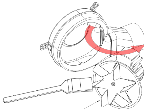
KROK 2. Oczyszczyć łopatki wirnika wentylatora.
