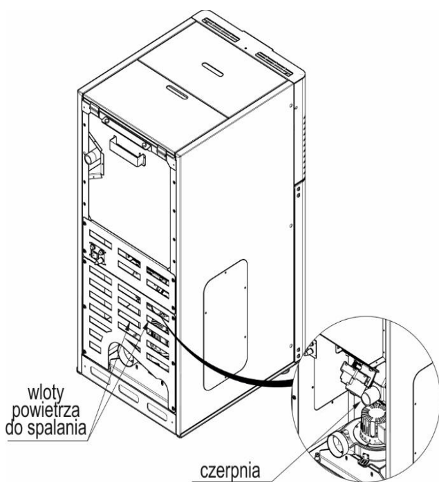
Rysunek 10. Czepnia powietrza - otwór dolotowy powietrza.
