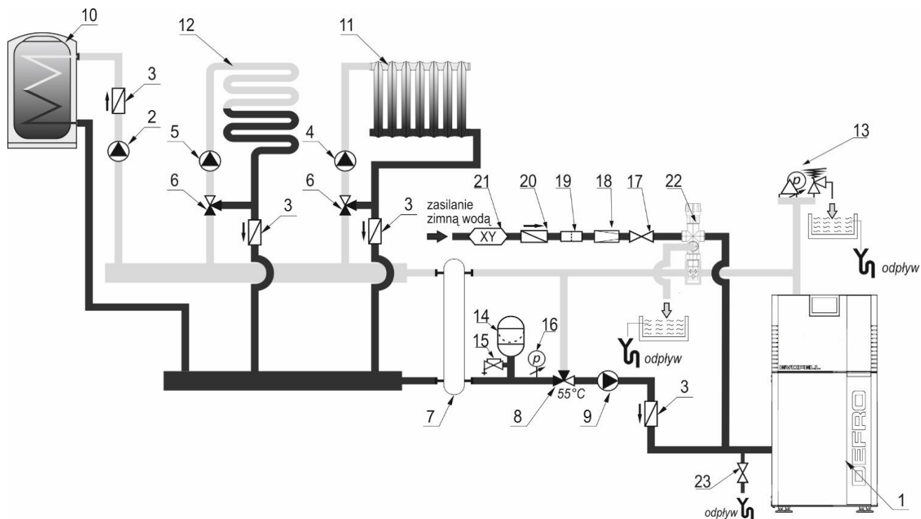
Rysunek 8. Uproszczony schemat instalacji grzewczej systemu zamkniętego.
