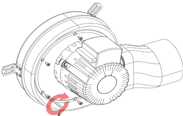
KROK 1. Odkręcić śruby mocujące wirnik wentylatora.
