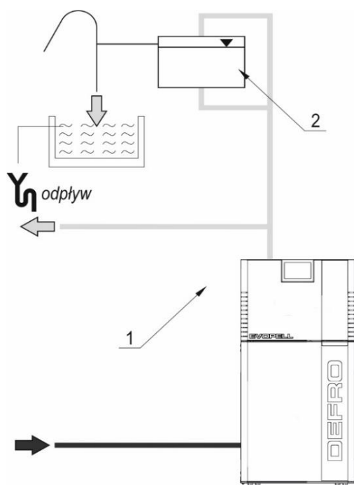
Rysunek 4. Przykładowy schemat zabezpieczeń kotła EVOPELL w układzie otwartym 1-kocioł; 2-otwarte naczynie zbiorcze.
