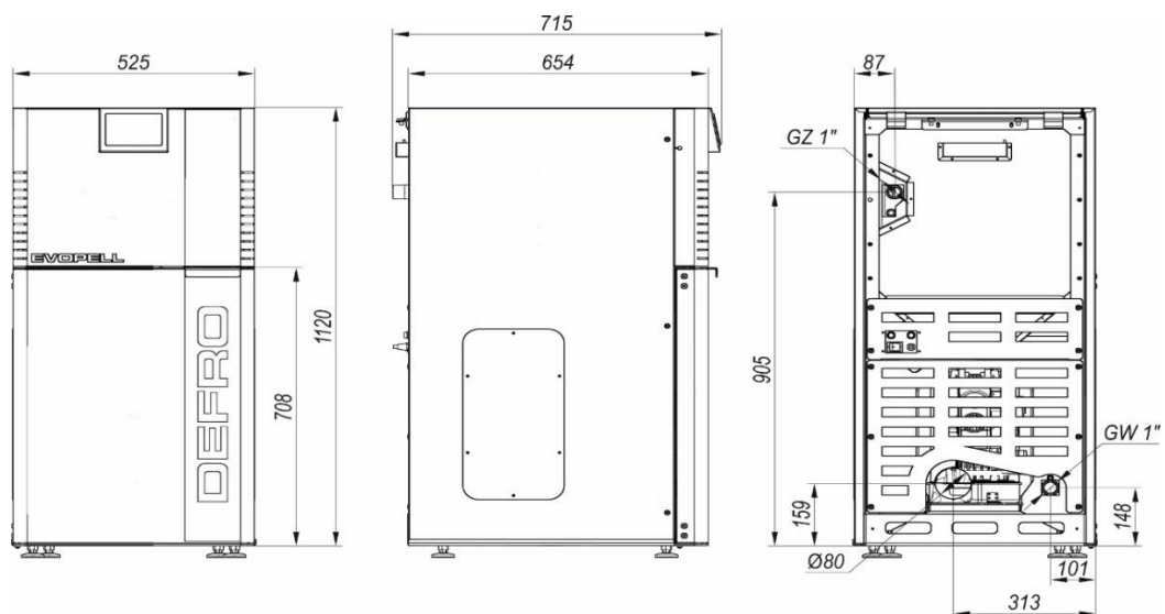
Rysunek 1. Podstawowe wymiary kotła.
