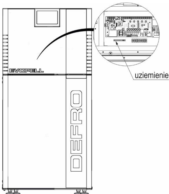
Rysunek 9 Uziemienie kotła.
