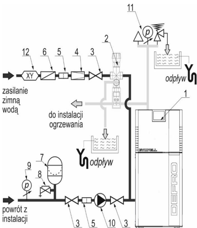
Rysunek 5. Przykładowy schemat zabezpieczeń kotła w układzie zamkniętym:
