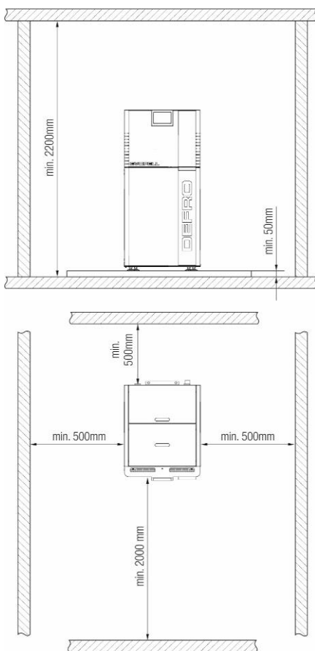
Rysunek 3. Ustawienie kotła w pomieszczeniu kotłowni.
