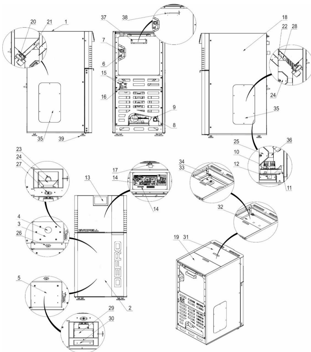
Rysunek 2. Podstawowe elementy kotła.
