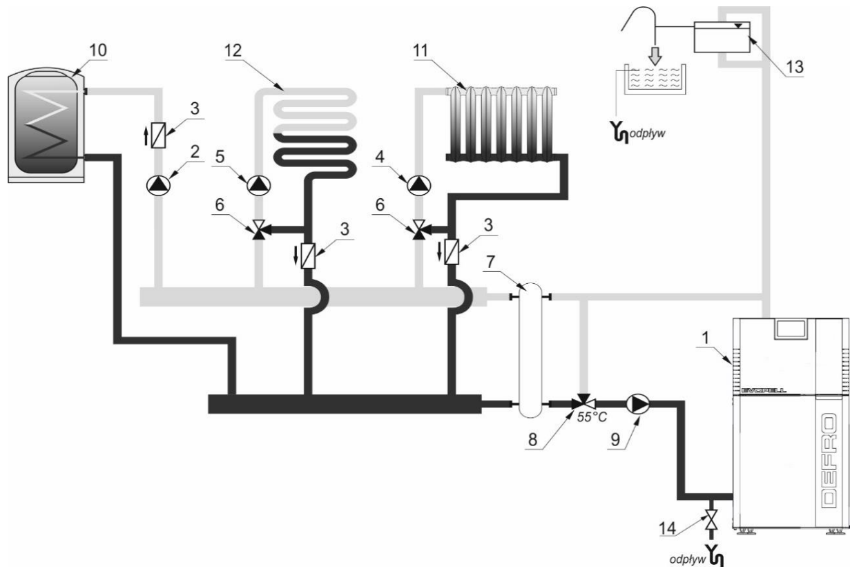
Rysunek 7. Uproszczony schemat instalacji grzewczej systemu otwartego.
