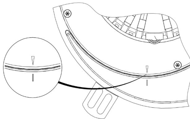
KROK 4. Zamontować ponownie wirnik wentylatora, sprawdzić poprawność montażu - znaczniki na wirniku i korpusie powinny się pokrywać.
