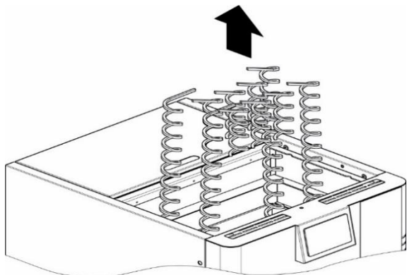
KROK 3. Ostrożnie wysunąć zawiówywacze
