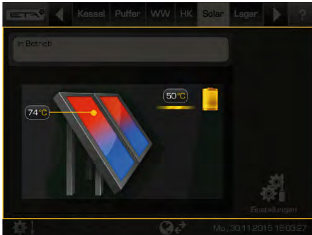
Abb. 5-84: Solaranlage mit externem Wärmetauscher am Puffer angeschlossen
