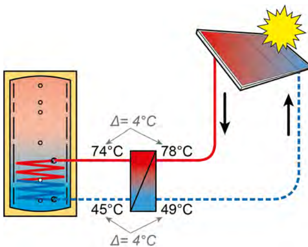
Abb. 5-85: Regelungsprinzip
