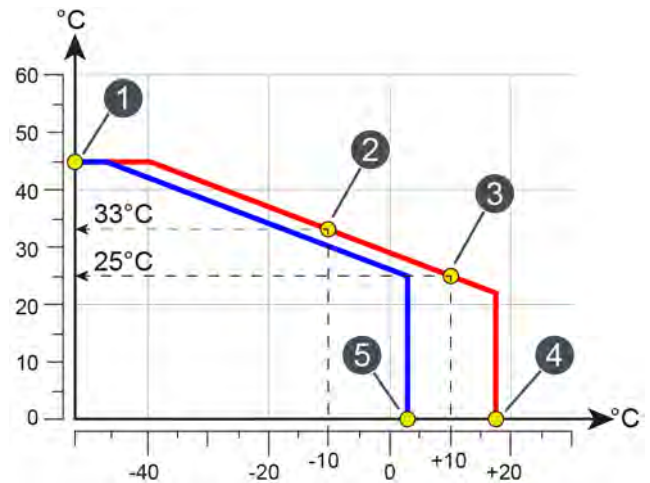
Abb. 5-71: Heizkurve einer Fußbodenheizung
