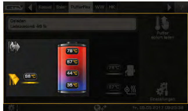
Abb. 5-60: Solaranlage am Puffer
