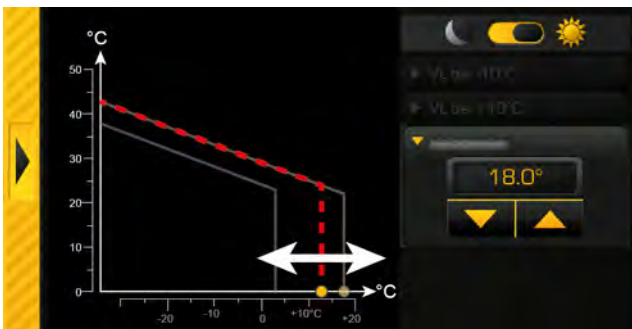
Abb. 5-79: Heizgrenze für den Heizbetrieb
