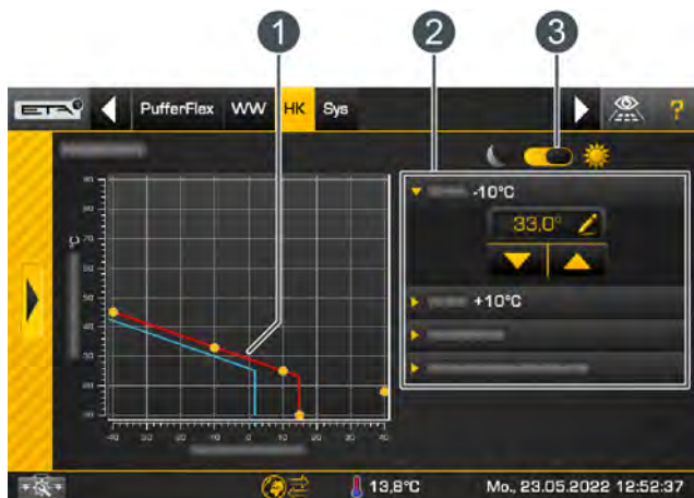
Abb. 5-70: Einstellungen der Heizkurve
