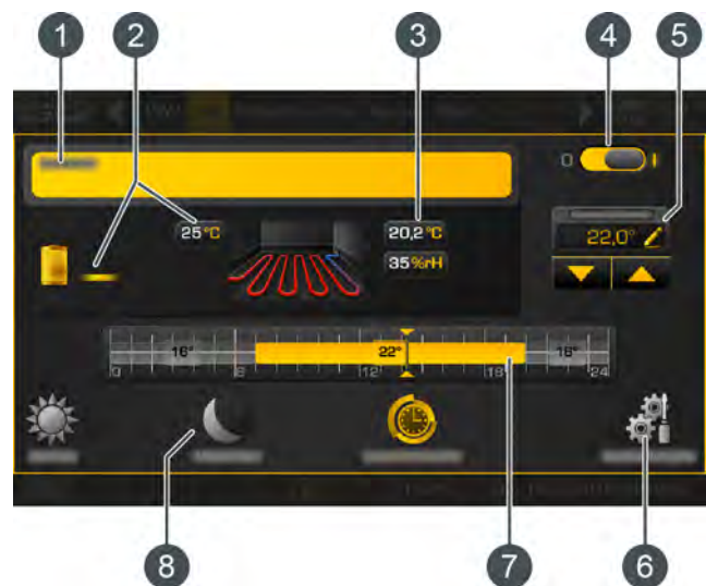
Abb. 5-3: Benutzeroberfläche des Heizkreises
