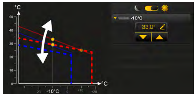
Abb. 5-77: Heizkurve anpassen (bei Außentemperaturen unter dem Gefrierpunkt)
