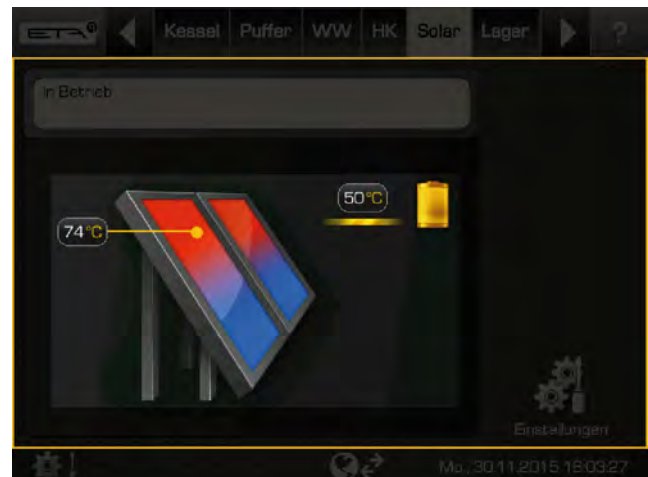
Abb. 5-81: Solaranlage am Puffer angeschlossen
