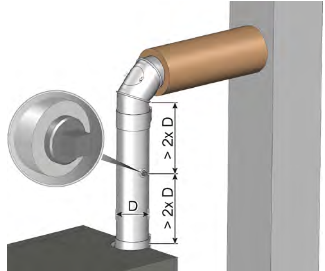
Abb. 6-1: Messöffnung
