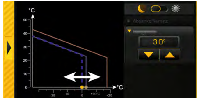
Abb. 5-80: Heizgrenze für den Absenkbetrieb
