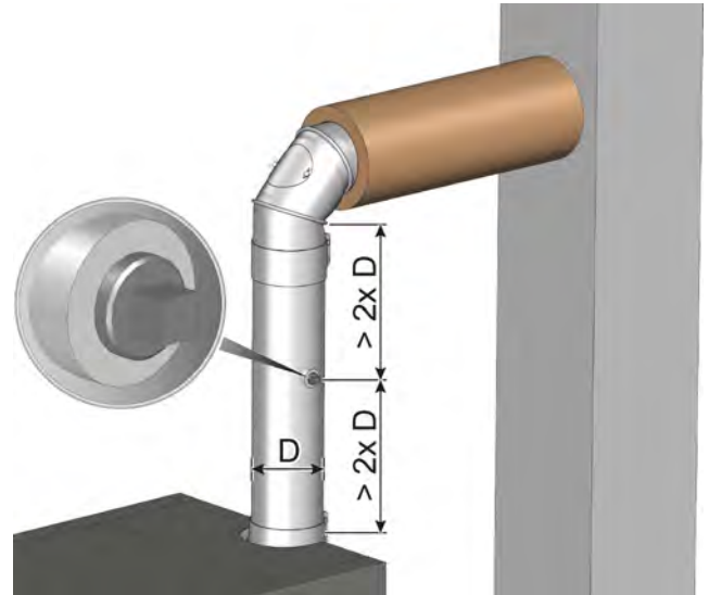
Abb. 6-1: Messöffnung
