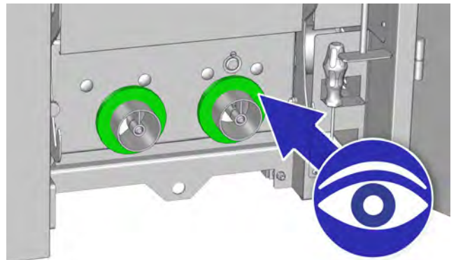
Abb. 4-4: Dichtungen
