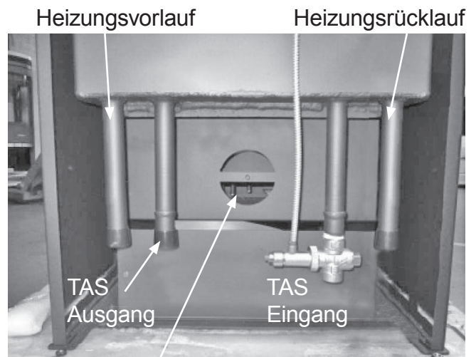
Anschluss externe Luftversorgung
