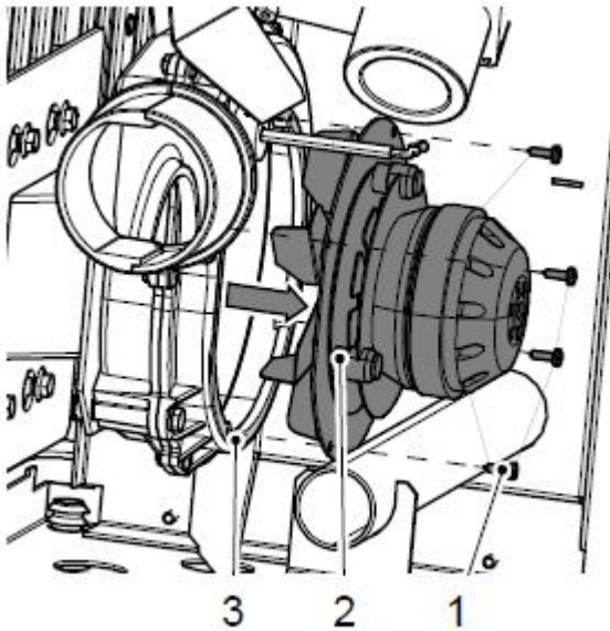
Abbildung 9: Saugzuggebläse
