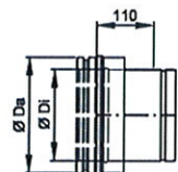
Anschlußübergang DW-EW
