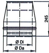
Mündungsabschluss
