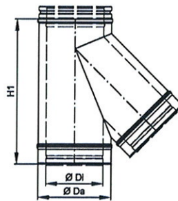
Rauchrohranschluss 45°
