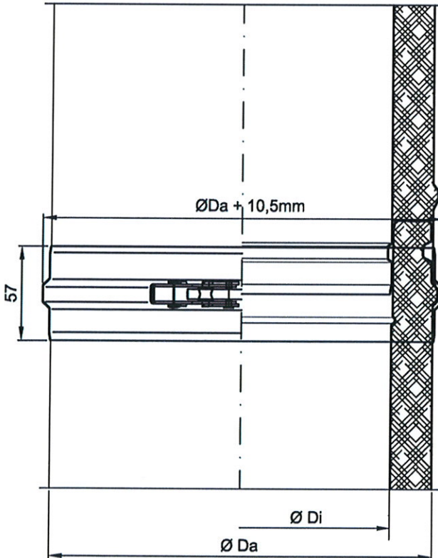
Klemmband schmal
