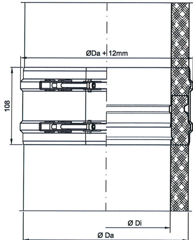
Klemmband breit
