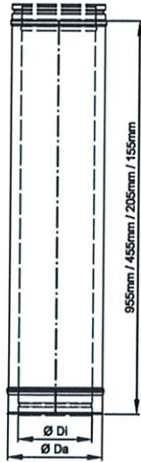
Normalrohr
