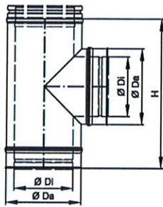
Rauchrohranschluss 90° / 85°
