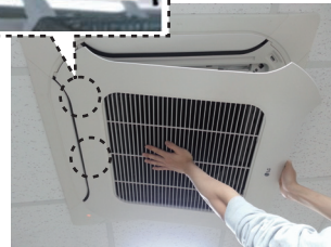
Einfügen der Kante in den Panelkörper
