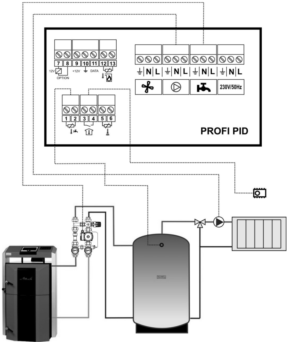
Einstellung der Parameter für Hydraulikschemata 3.3: ur = ur4
