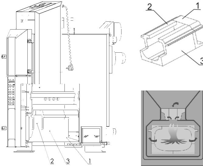
Kesselschnitt – Verbrennungskammer
