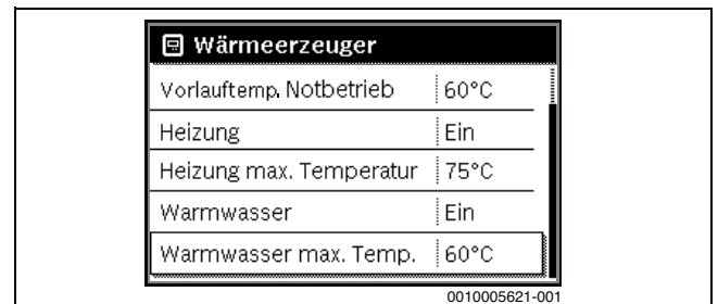
Bild 21 Maximale Warmwassertemperatur
