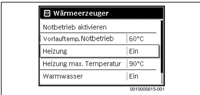
Bild 17 Menü Wärmeerzeuger-Heizung
