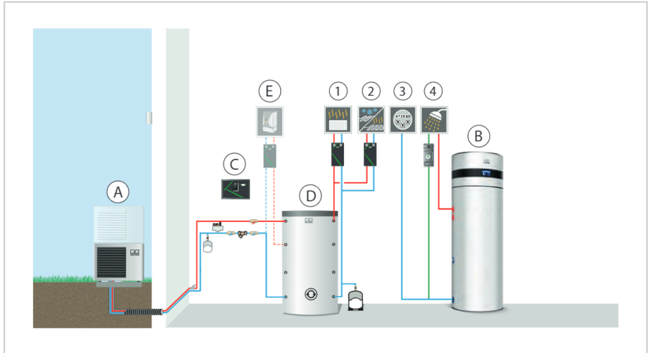
Abb. 12: Beispiel 1 - Hydraulikschema
