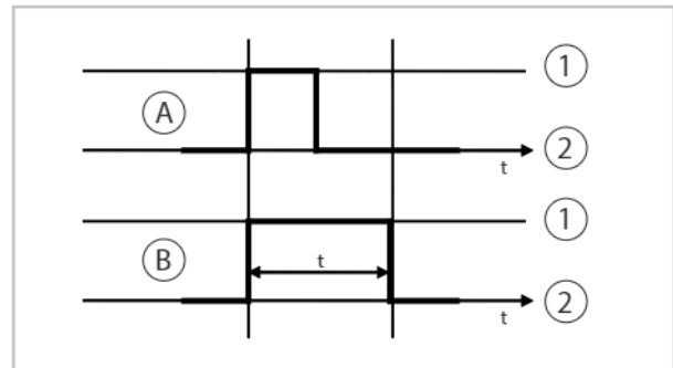
Abb. 16: Kontrolllogik Einschaltzeit
