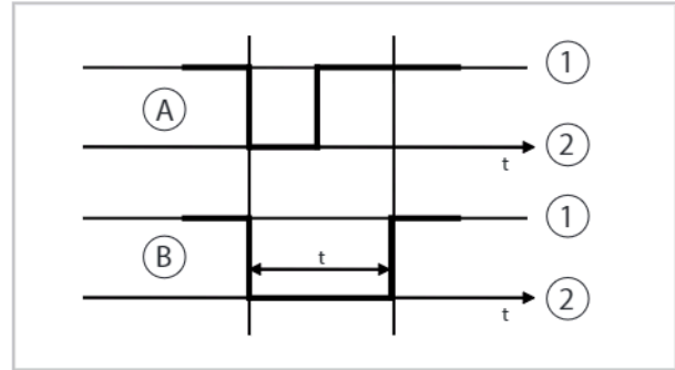
Abb. 15: Kontrolllogik Ausschaltzeit
