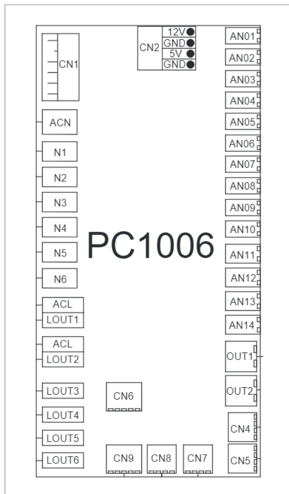
Abb. 14: Anschlüsse Leistungsplatine
