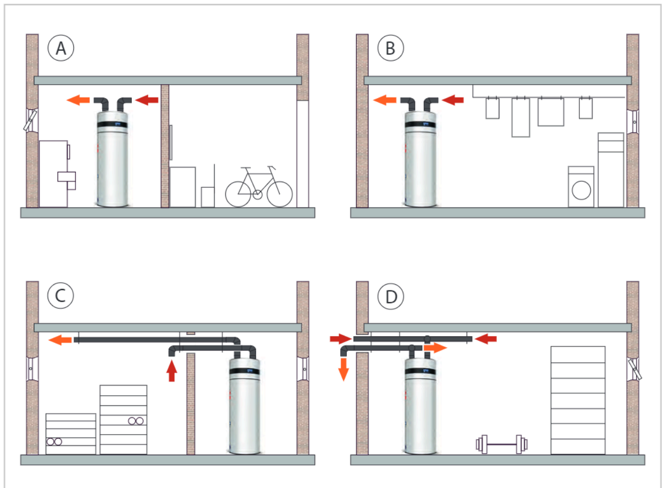
Abb. 10: Installationsmöglichkeiten
