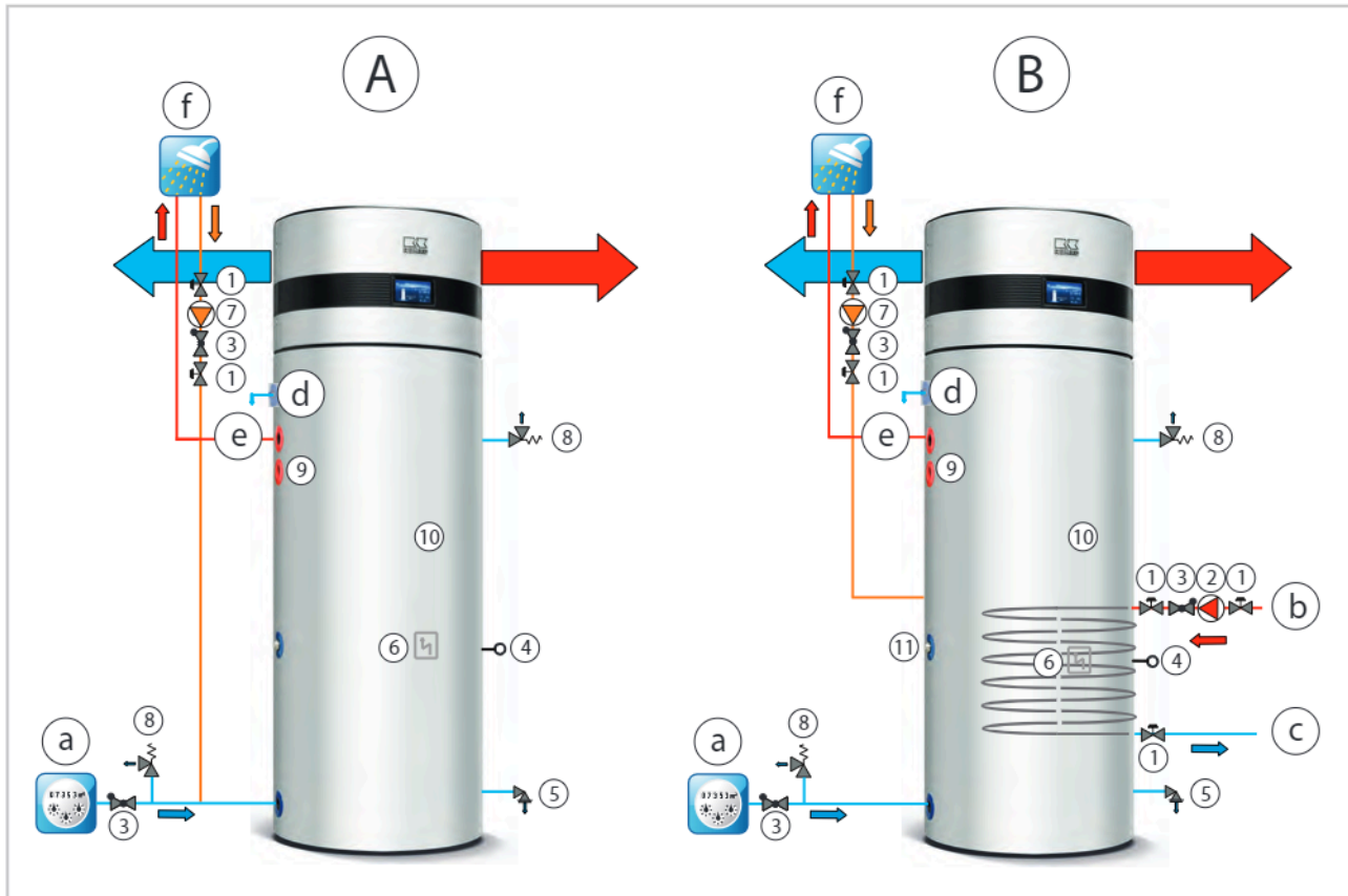
Abb. 11: Hydraulisches Anschlussschema
