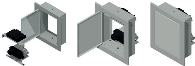
Abb. 6. Montage des Gassteuergerätes zusammen mit dem Empfangsgerät im Verteilerkasten
