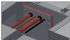
Abb. 9. Ableitung und Abdichtung der Leitung der Kapillare, der Magnetzündleitung, der Röhre des Hauptbrenners und der Röhre des Kontrollbrenners
