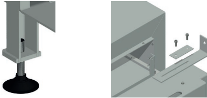
Abb. 3. Nivellierungsfuß und verstellbarer Spannhalter
