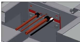
Abb. 9. Ableitung und Abdichtung der Leitung der Kapillare, der Magnetzündleitung, der Röhre des Hauptbrenners und der Röhre des Kontrollbrenners
