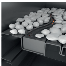
Rys. 18. Poprawne rozmieszczenie elementów dekoracyjnych - kamienie
