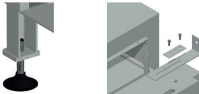
Rys. 3. Stopka poziomująca oraz regulowany uchwyt mocujący
