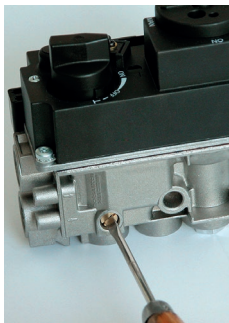
Rys. 13. Sposób regulacji minimalnej wysokości płomienia palnika głównego
