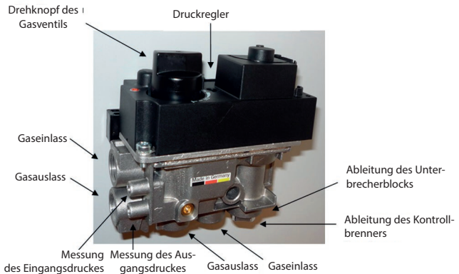
Abb. 11. Steuergerät GV60 in der Grundstellung
