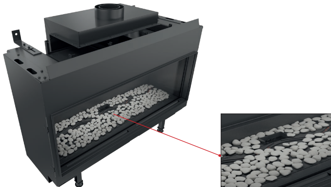
Рис.19. Правильное размещение декоративных элементов- камни
