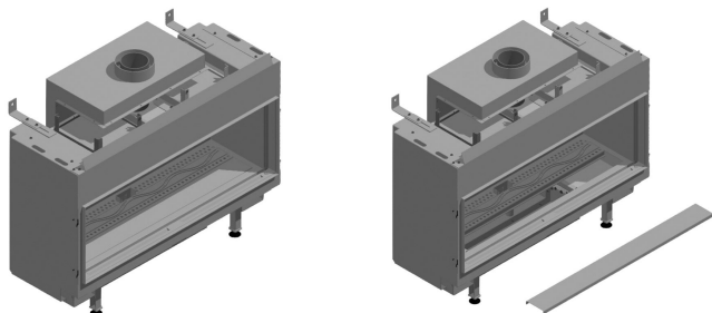
Abb. 8. Demontage des Revisionselementes
