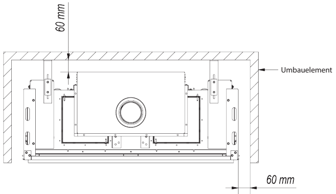
Abb. 4. Mindestentfernungen des Gaskamineinsatzes von unbrennbaren Umbaelementen
