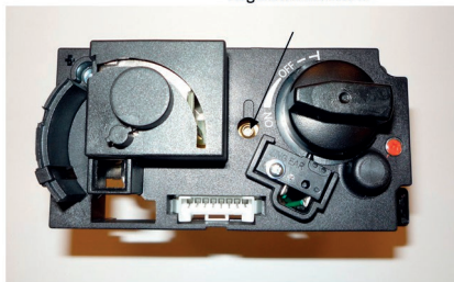
Rys. 12. Sposób regulacji ciśnienia wylotowego
