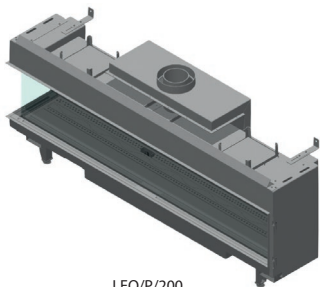
Abb. 1 Gaskamineinätze von der Serie LEO 100 und LEO 200
