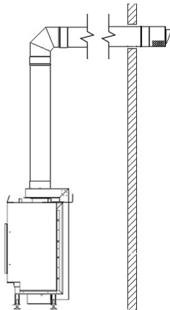
Abb. 5. Durchführung des konzentrischen Schornsteinsystems
