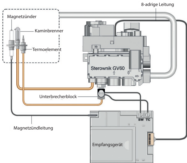
Rys. 7. Schemat podłączenia poszczególnych elementów systemu sterowania gazem.
