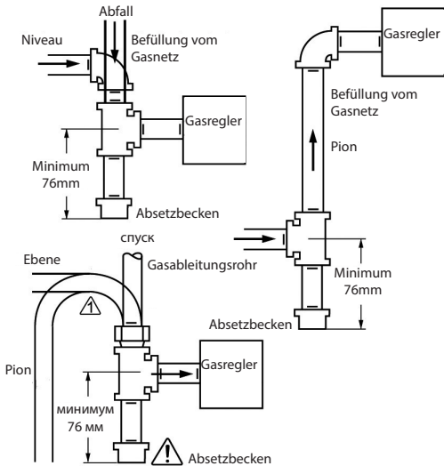
Abb. 10 Montage des Absetzbeckens (falls es erforderlich ist)
