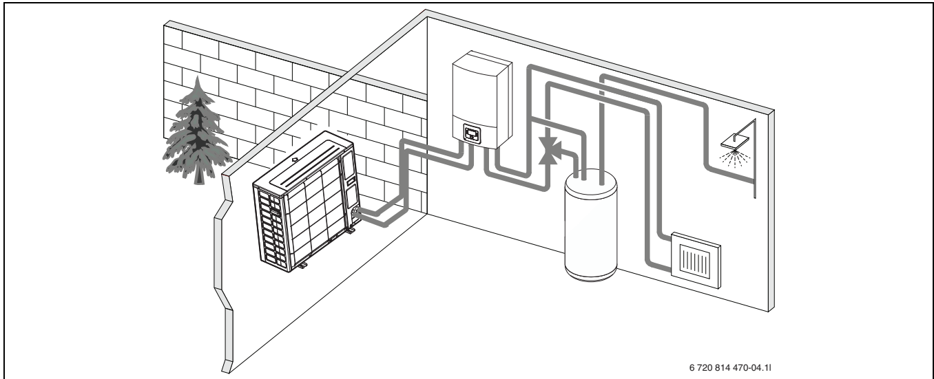
Bild 2 Wärmepumpe Ausseneinheit, Inneneinheit ASE mit elektrischem Zuheizung, externer Warmwasserspeicher
