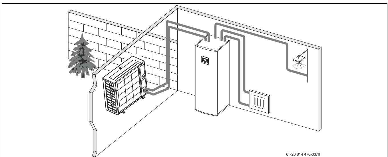
Bild 1 Wärmepumpe Ausseneinheit, Inneneinheit ASM/ASMS mit integriertem Warmwasserspeicher und elektrischem Zuheizter
