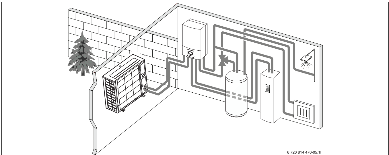
Bild 3 Wärmepumpe Ausseneinheit, Inneneinheit ASB ohne elektrischen Zuheizung, externer Warmwasserspeicher und externer Zuheizung
