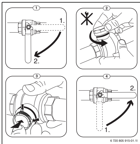
Bild 5 Filtervariante ohne Sicherungsring
