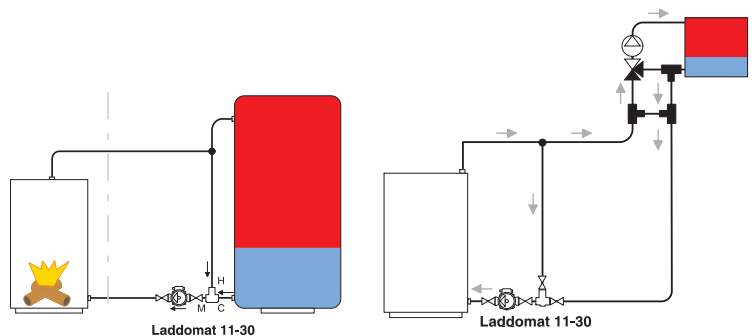
Laddomat 11-30 am Pufferspeicher oder am Kessel anschließen
