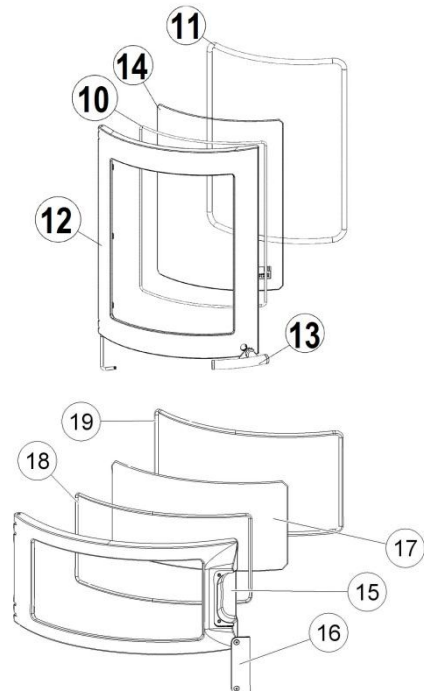
Nummerierung Keramott = Einbaureihenfolge!
